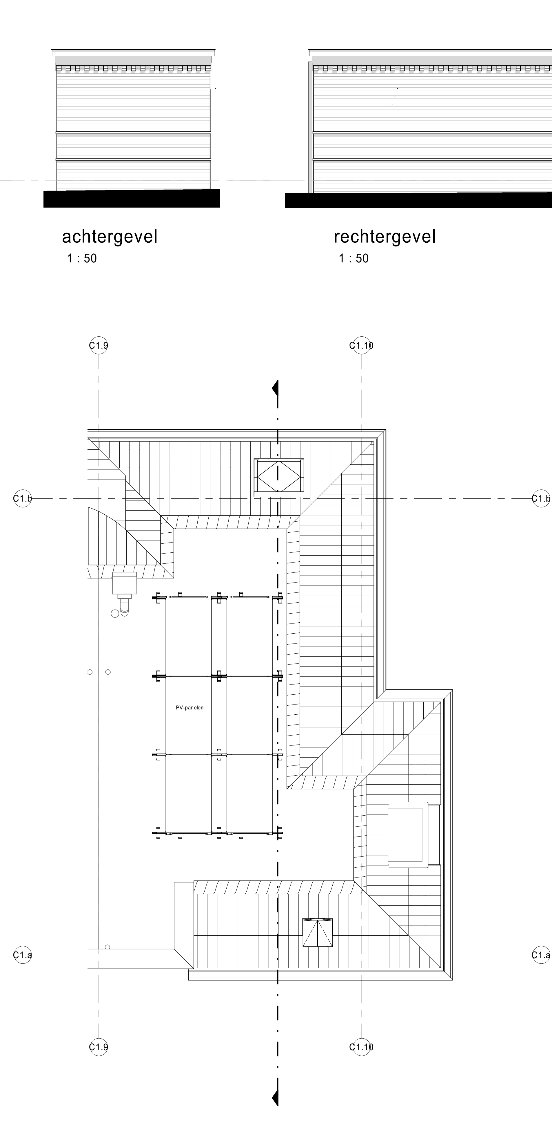
dak 1 : 50
