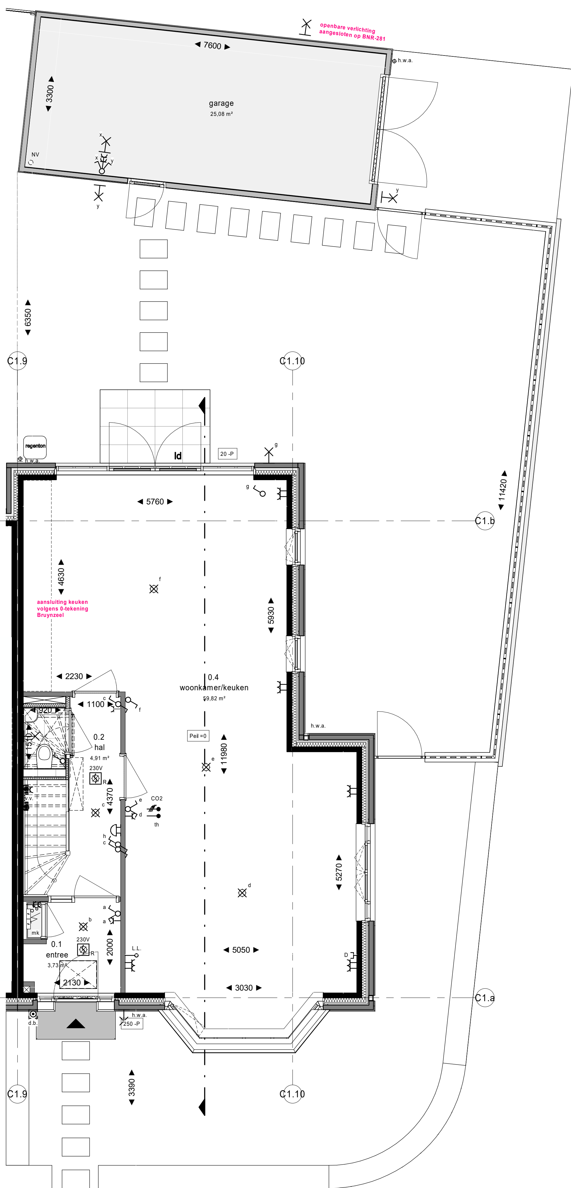
begane grond 1 : 50
