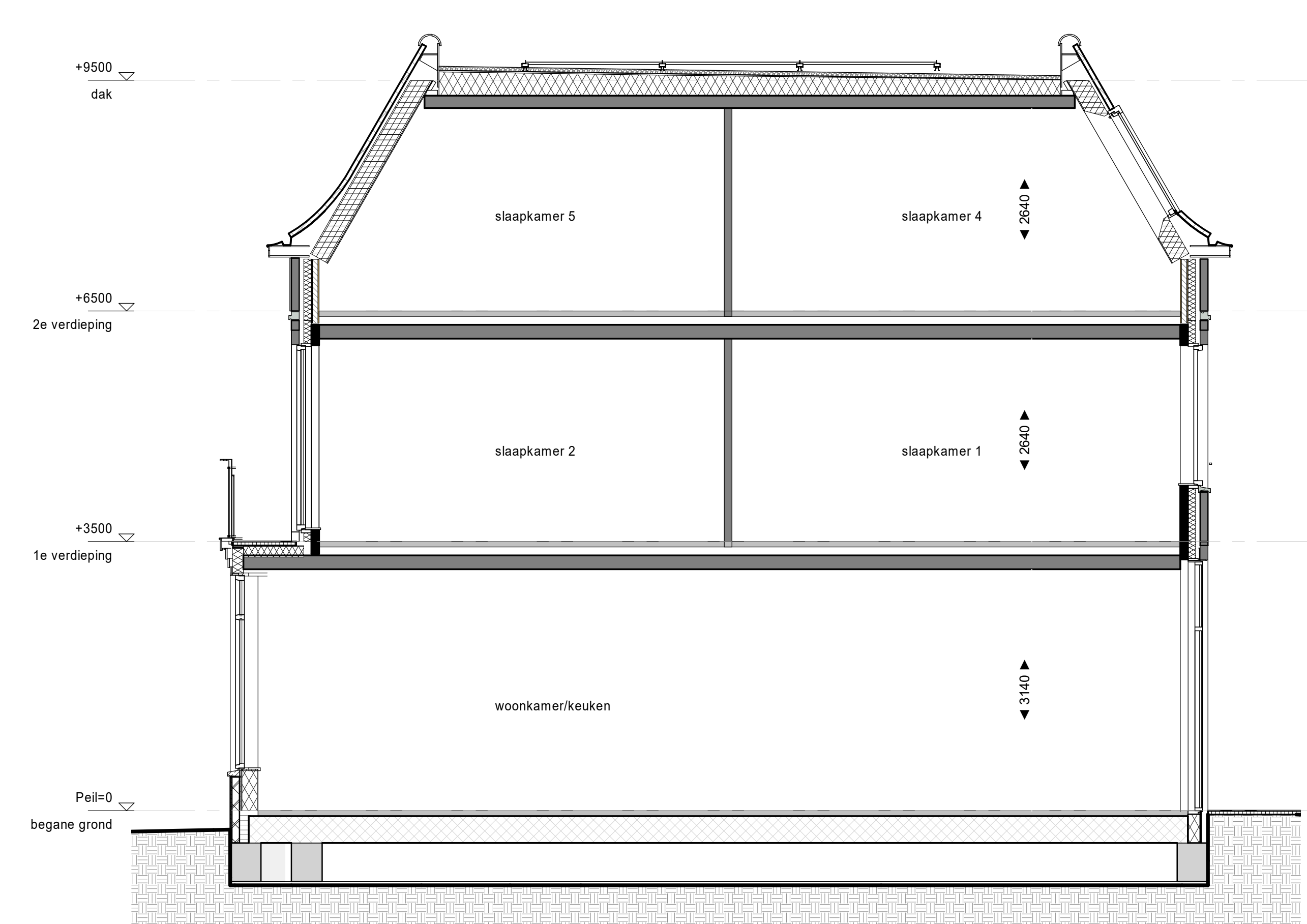
doorsnede 1 : 50
