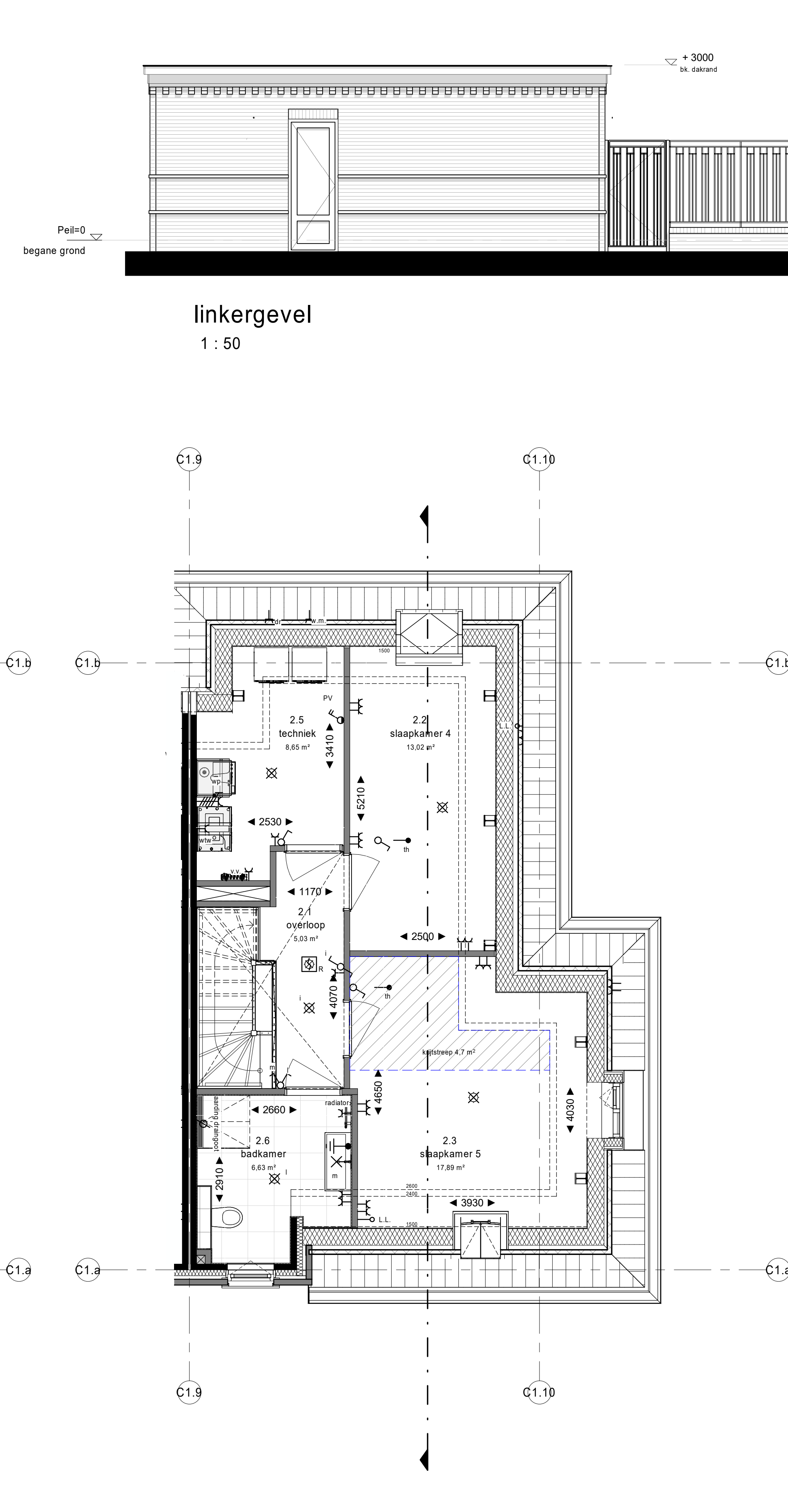
tweede verdieping 1 : 50
