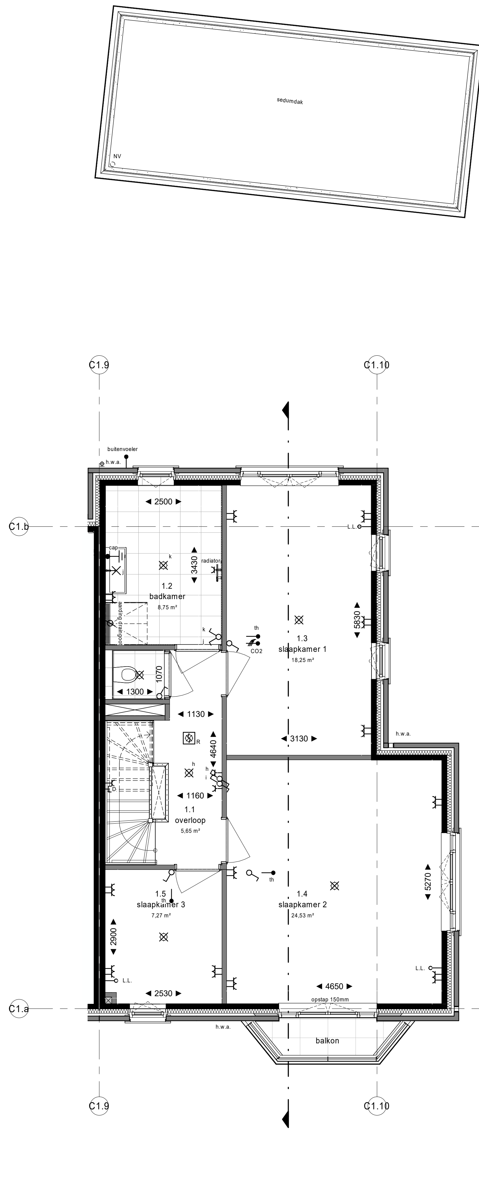
eerste verdieping 1 : 50
