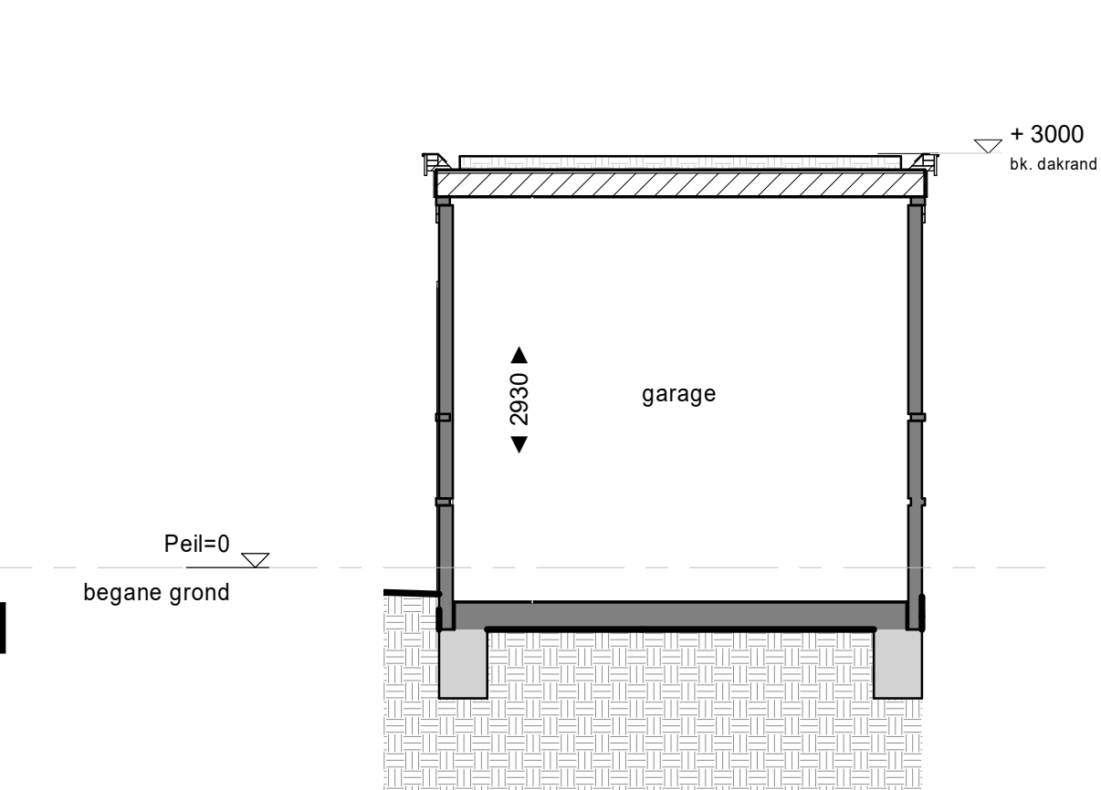
doorsnede 1 : 50
