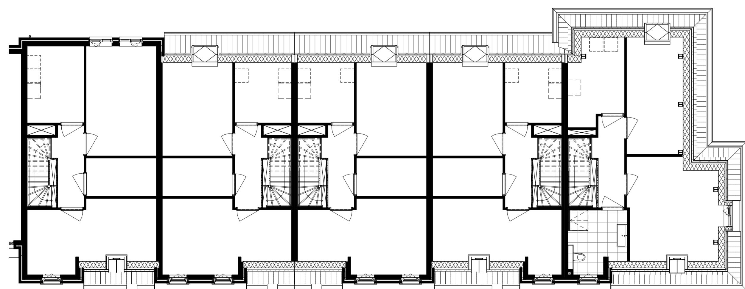
begane grond
