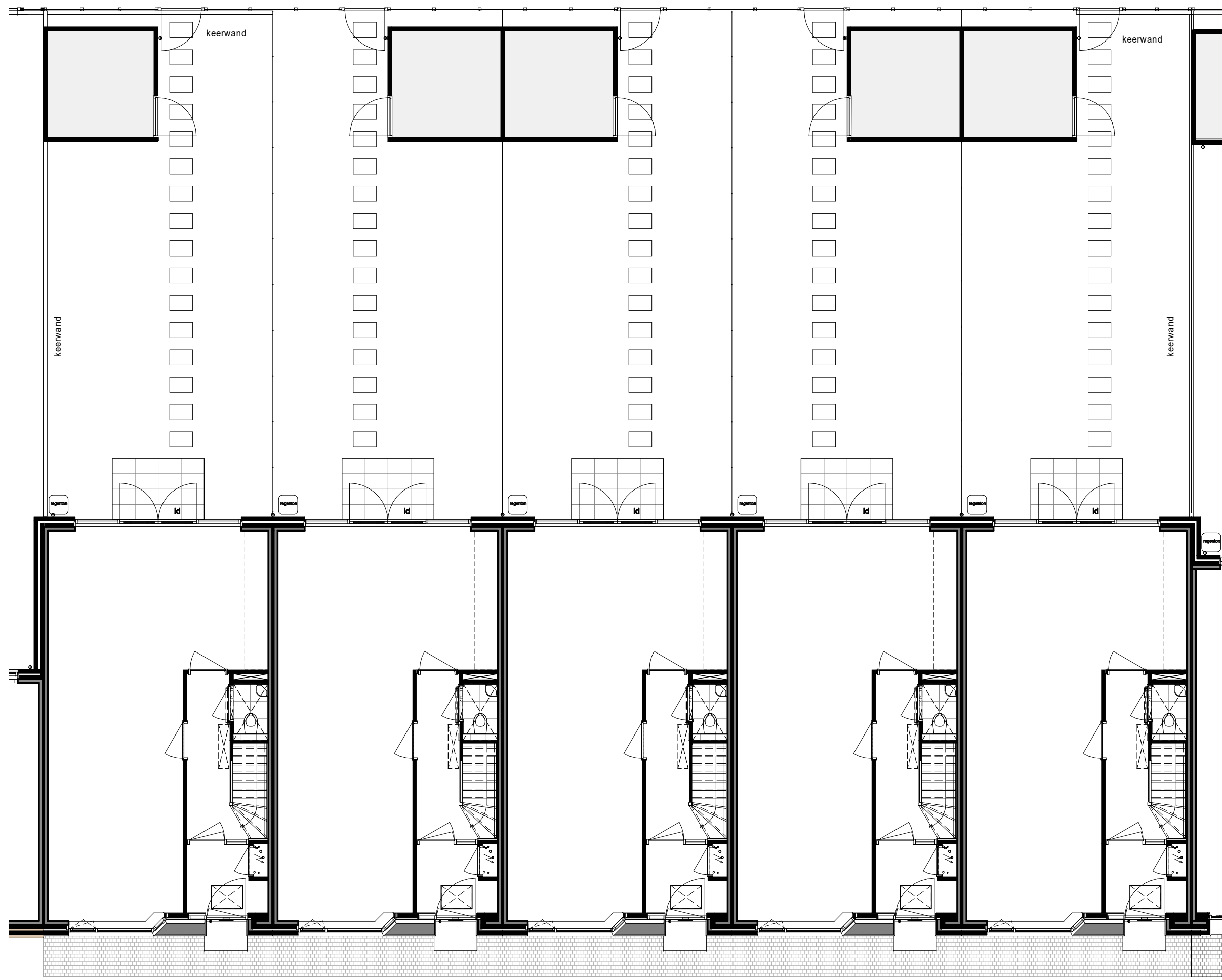
begane grond
