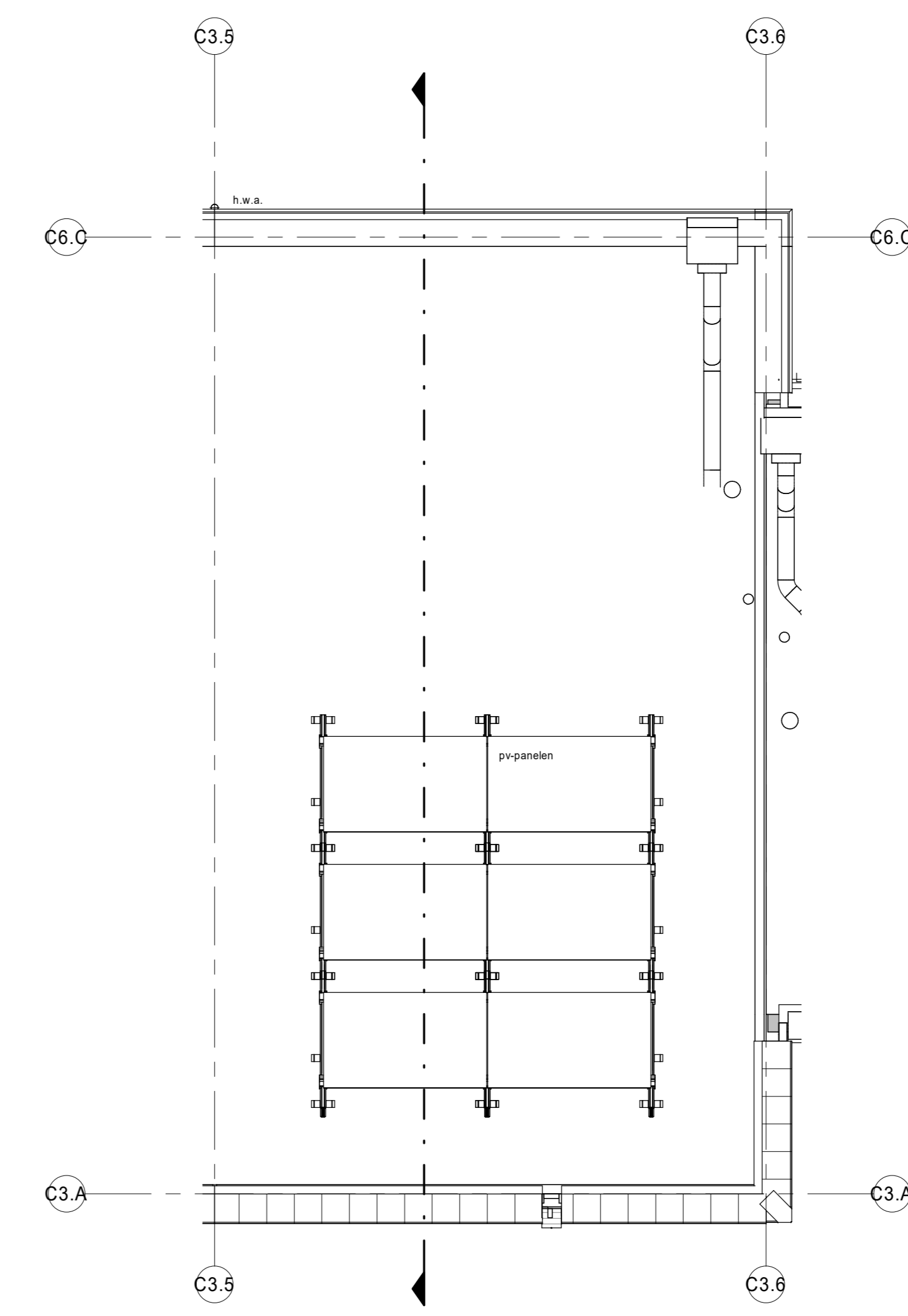
dak 1 : 50 Bnr 311
