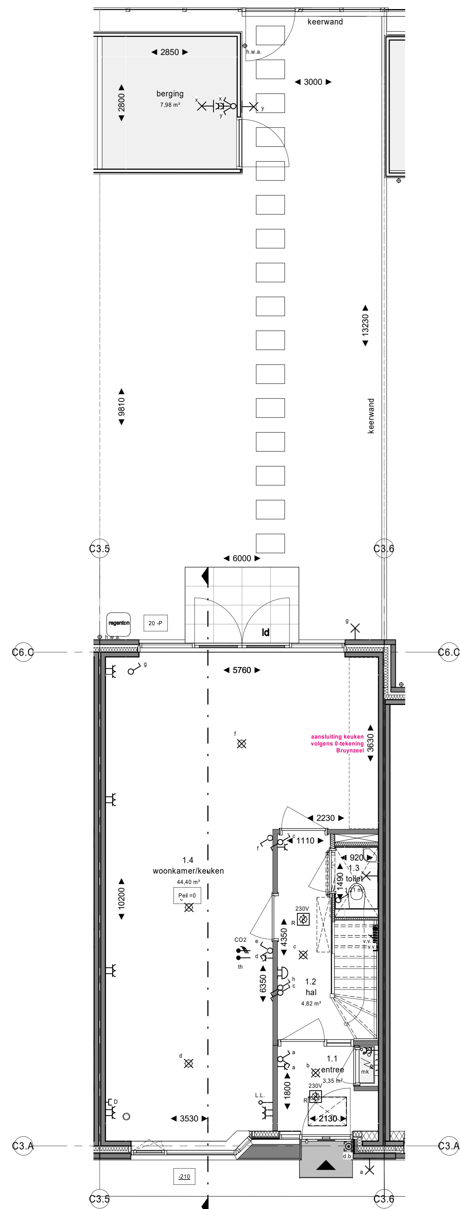
begane grond 1 : 50
