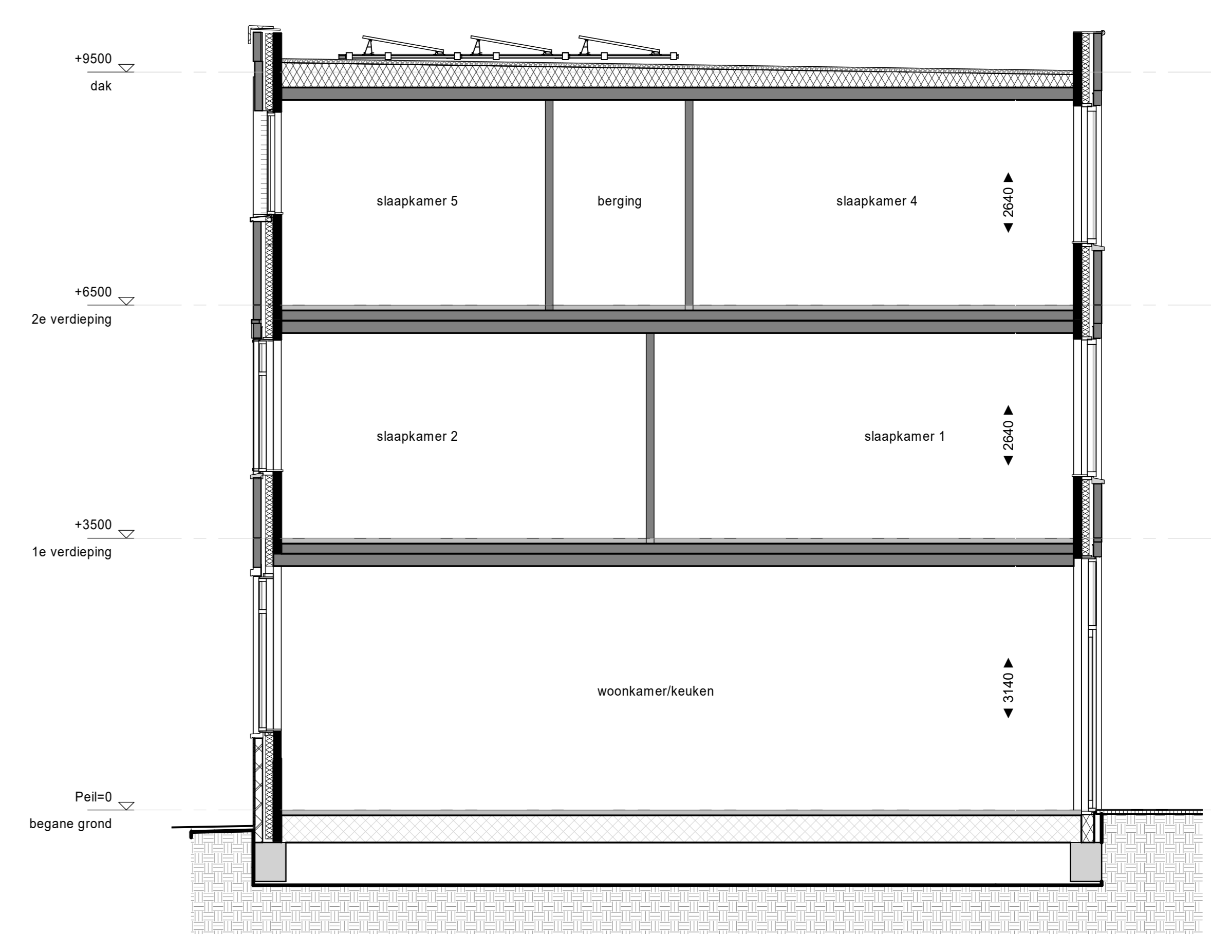
doorsnede 1 : 50
