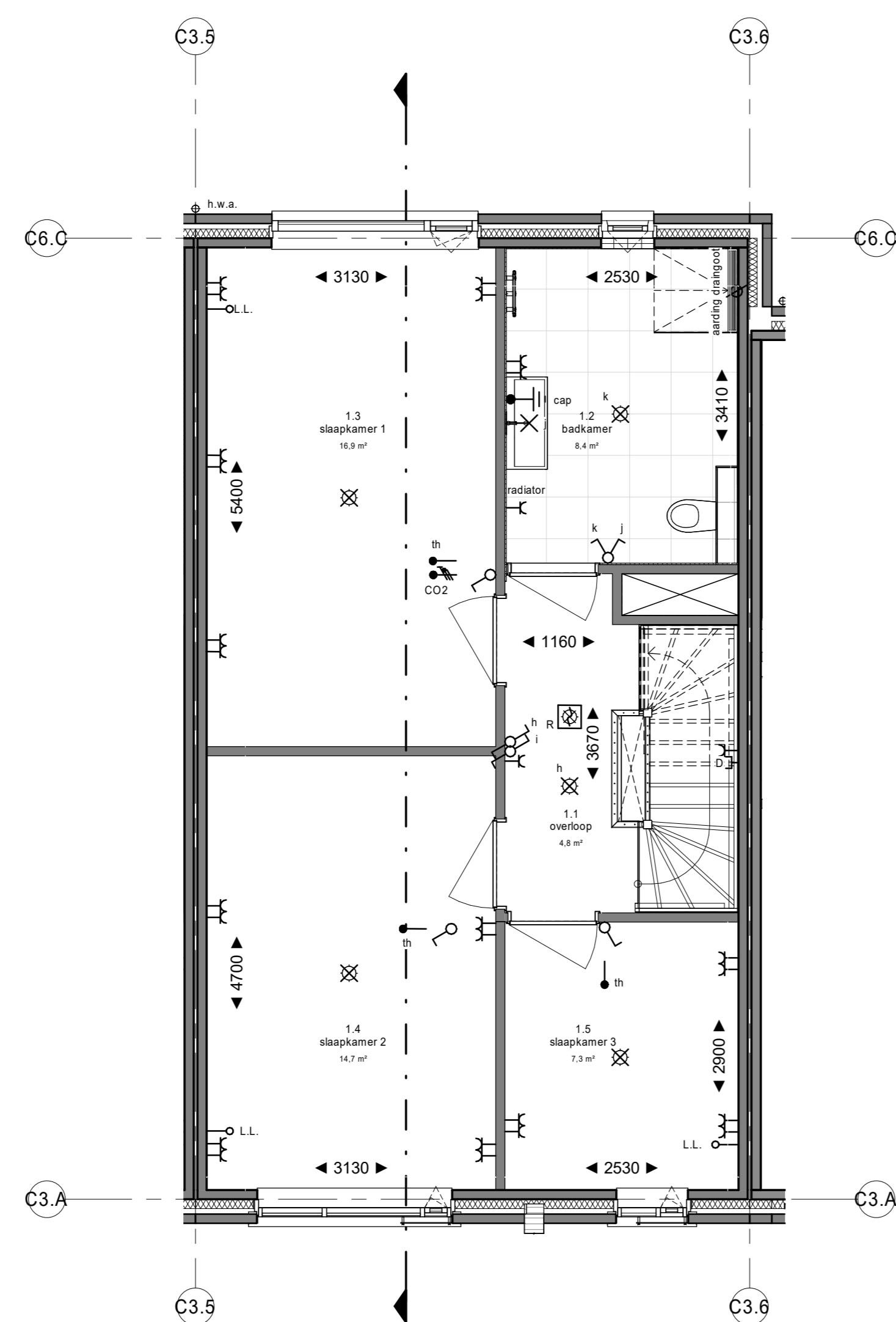
eerste verdieping 1 : 50
