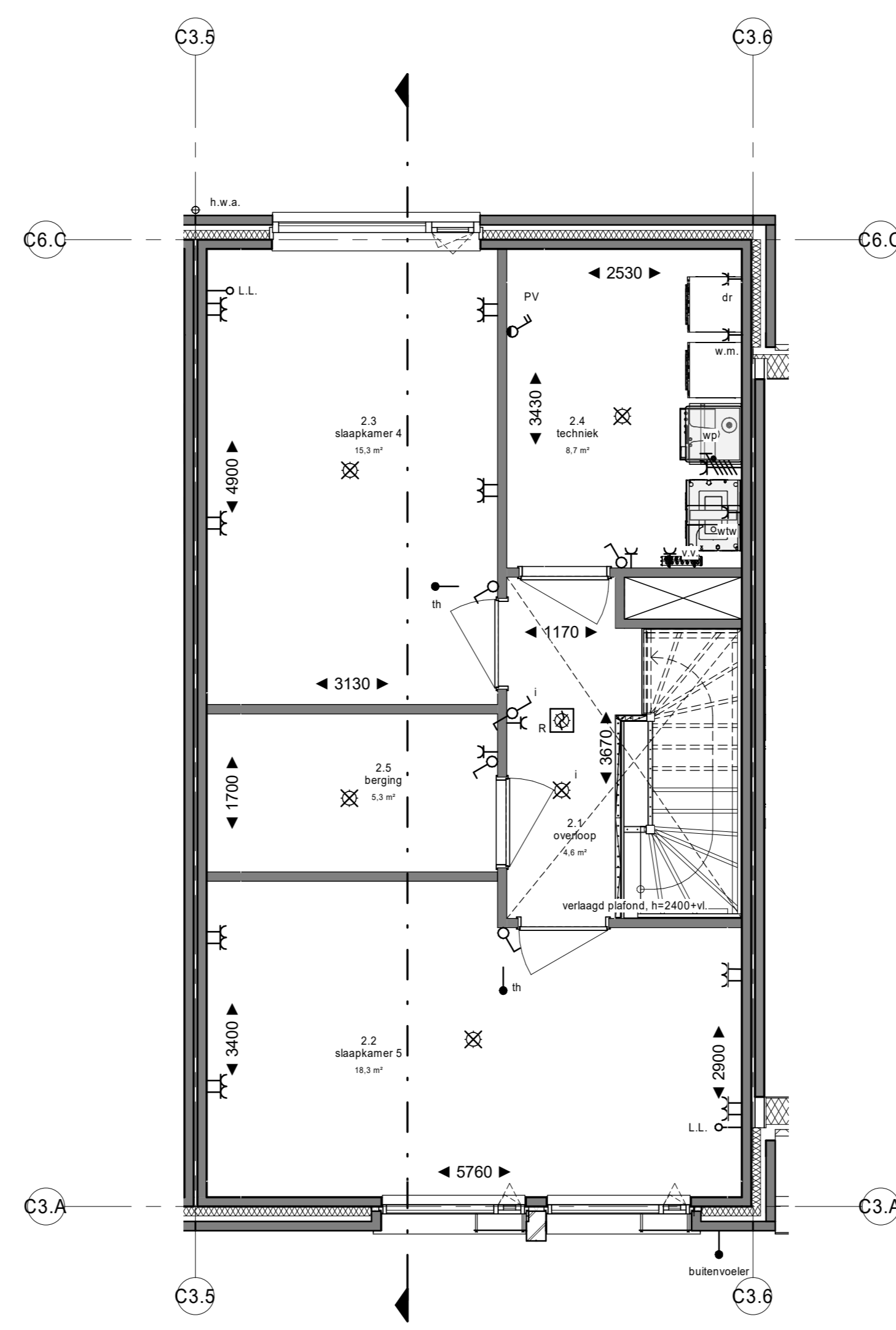
tweede verdieping 1 : 50
