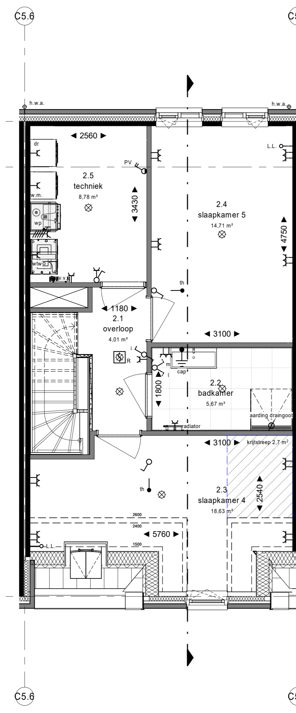
tweede verdieping 1 : 50
