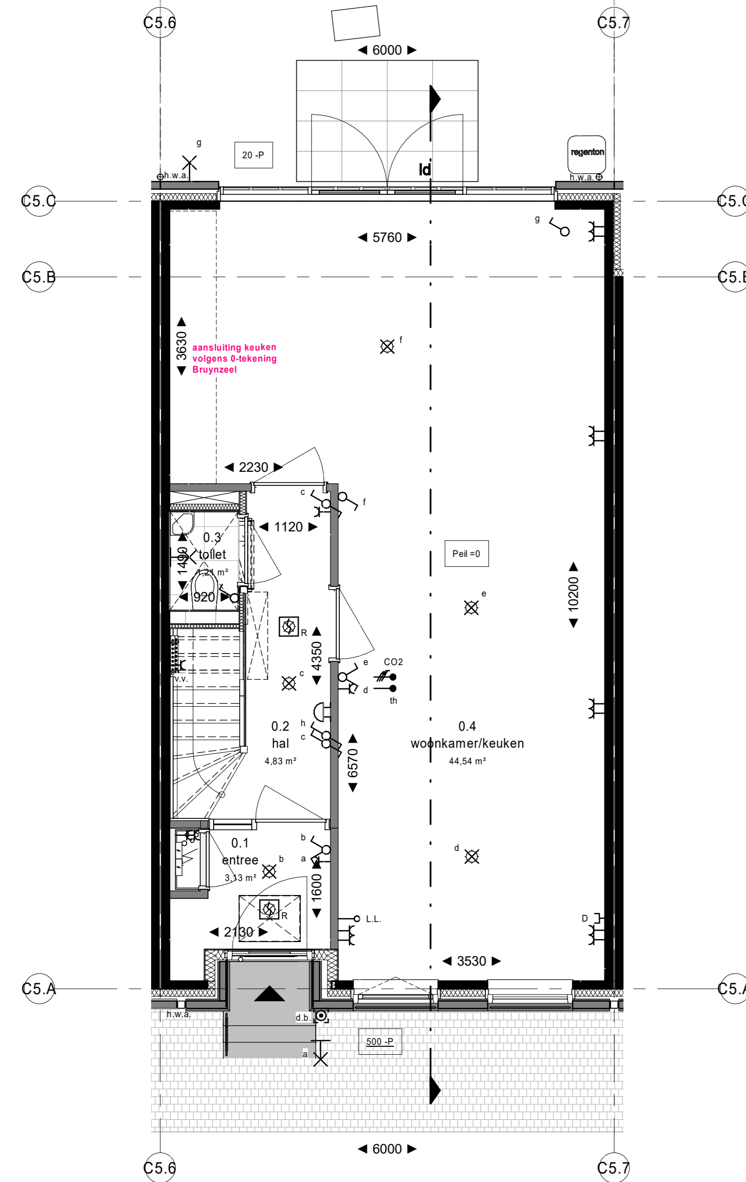
begane grond 1 : 50
