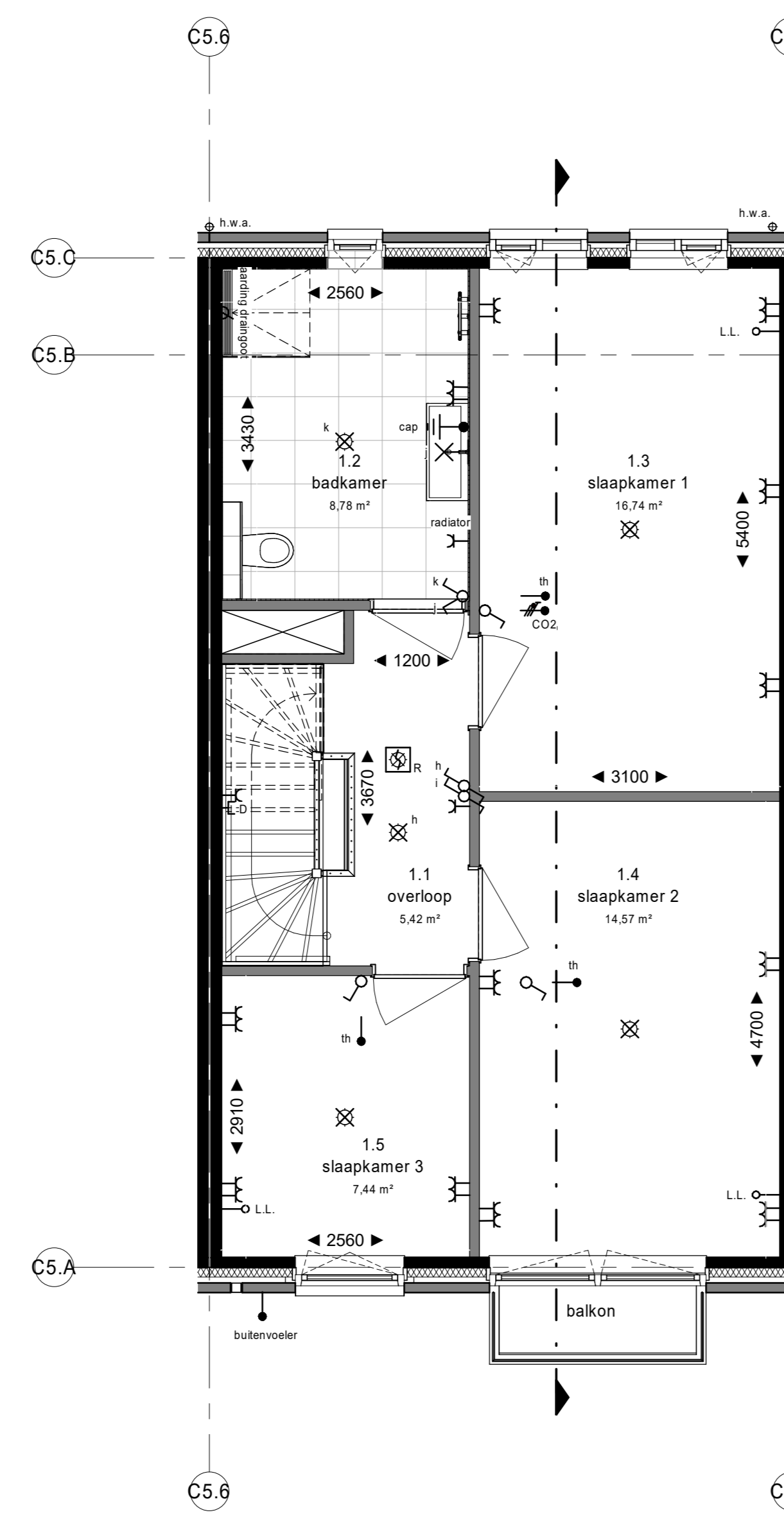
eerste verdieping 1 : 50
