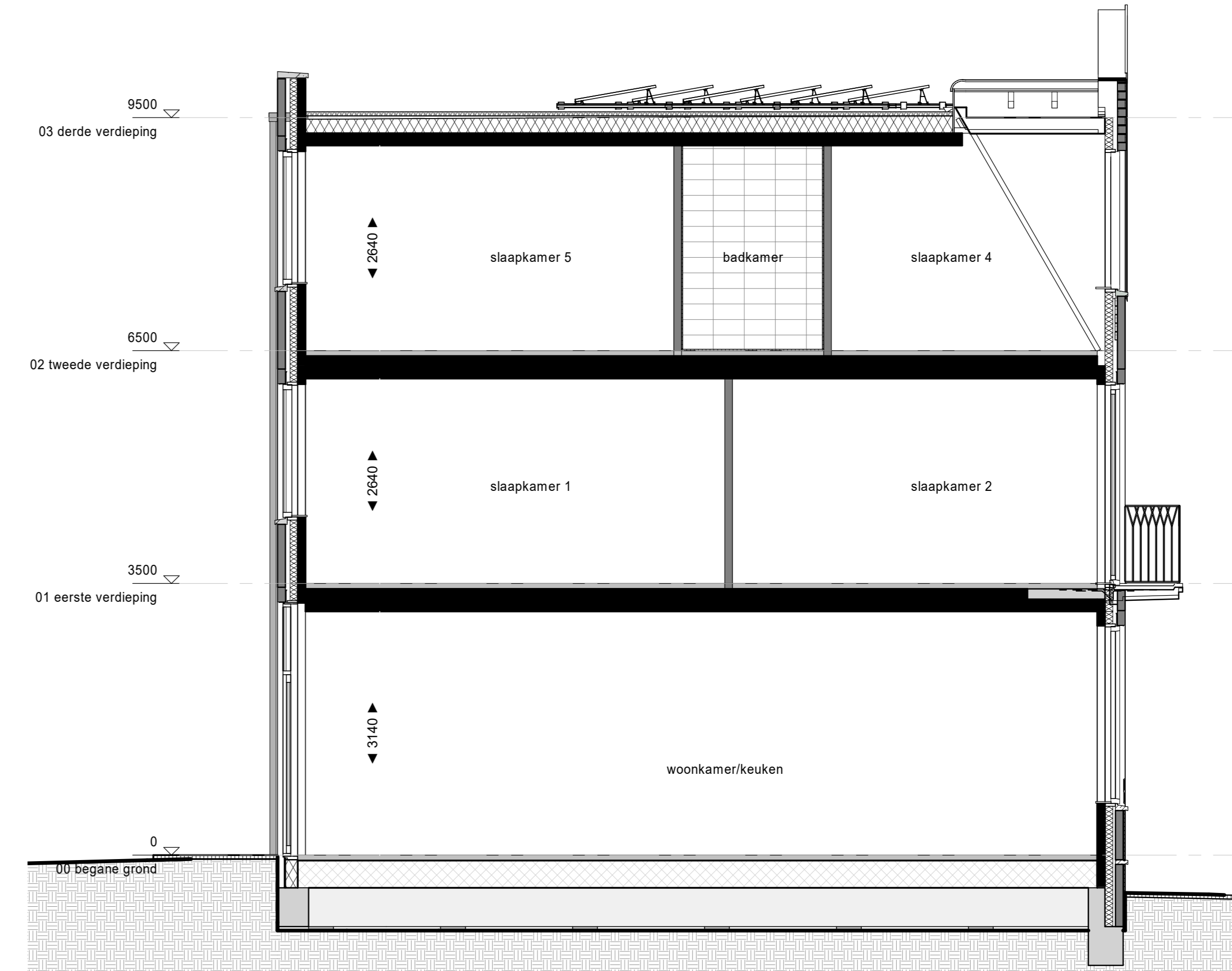
doorsnede 1 : 50
