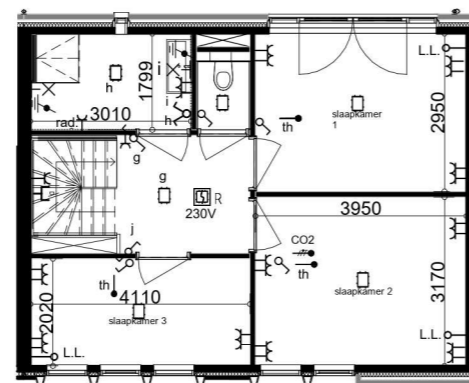
Eerste verdieping bnr. 340 Optie woning indeling i.p.v. casco
