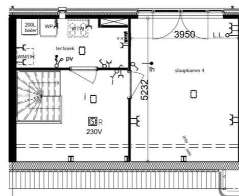
Tweede verdieping bnr. 340 Optie woning indeling i.p.v. casco
