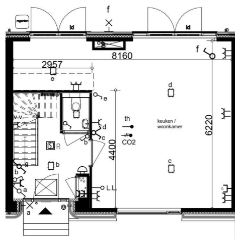
Begane Grond bnr. 340 Optie woning indeling i.p.v. casco
