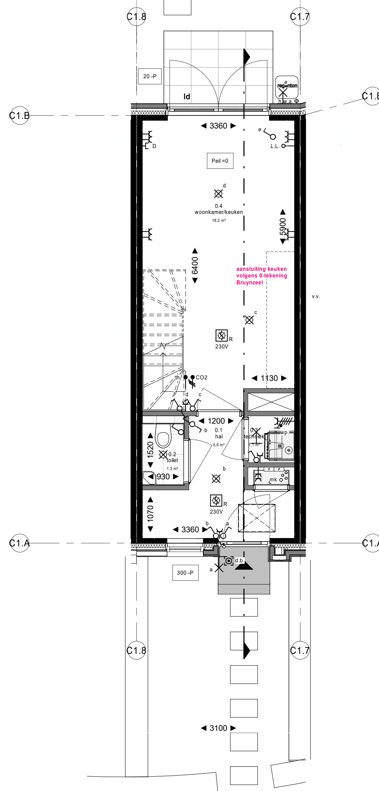
begane grond 1 : 50
