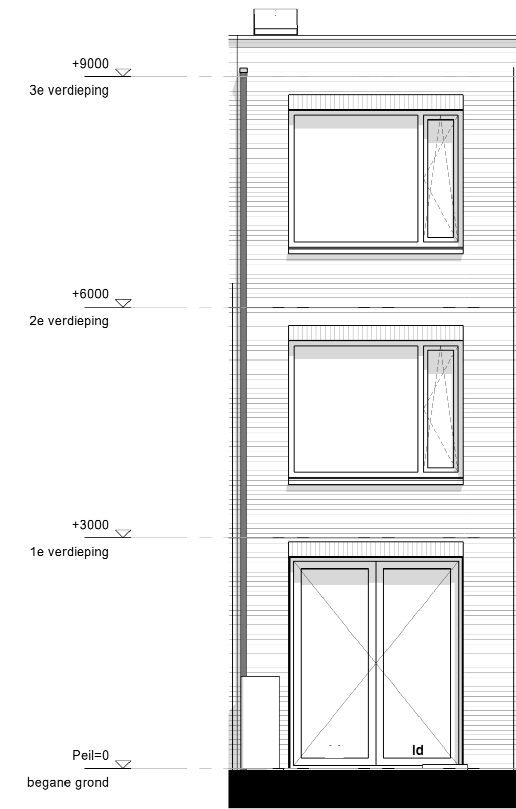
achtergevel 1 : 50
