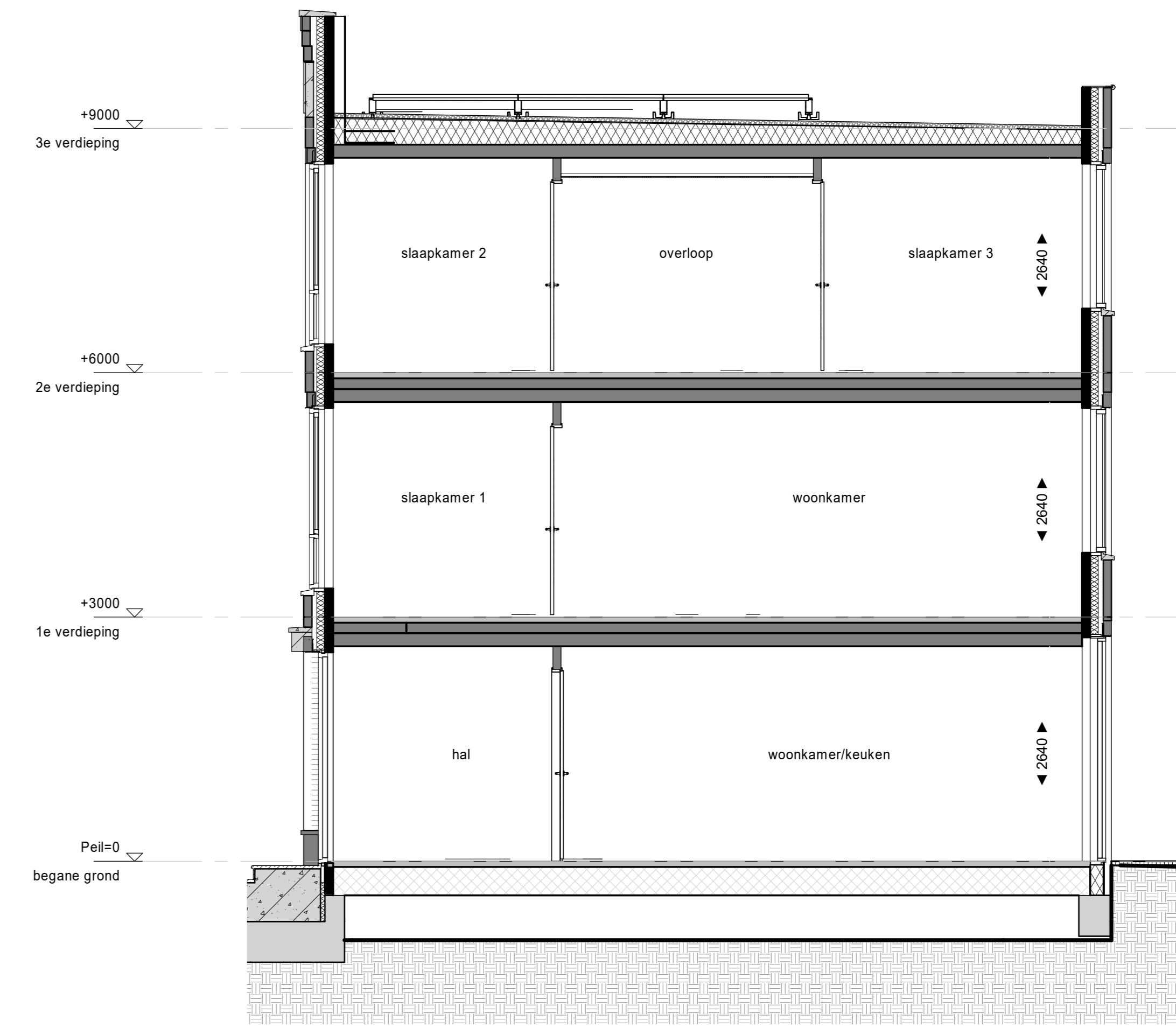
doorsnede 1 : 50
