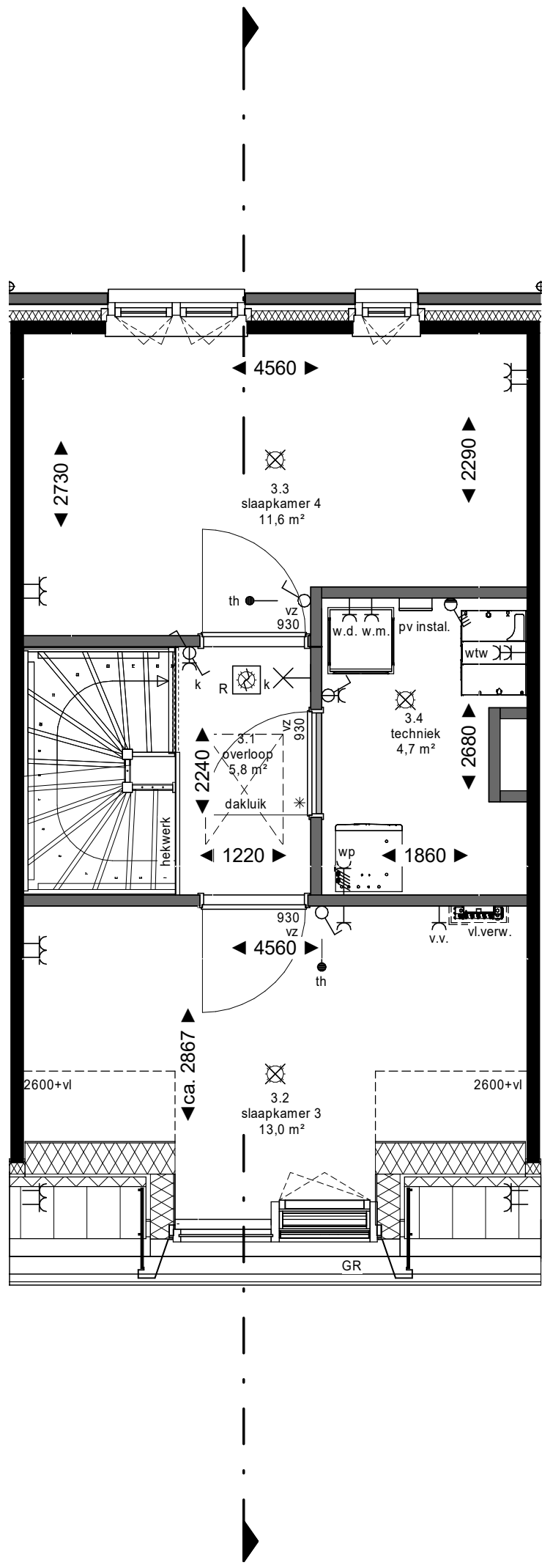
3e verdieping
