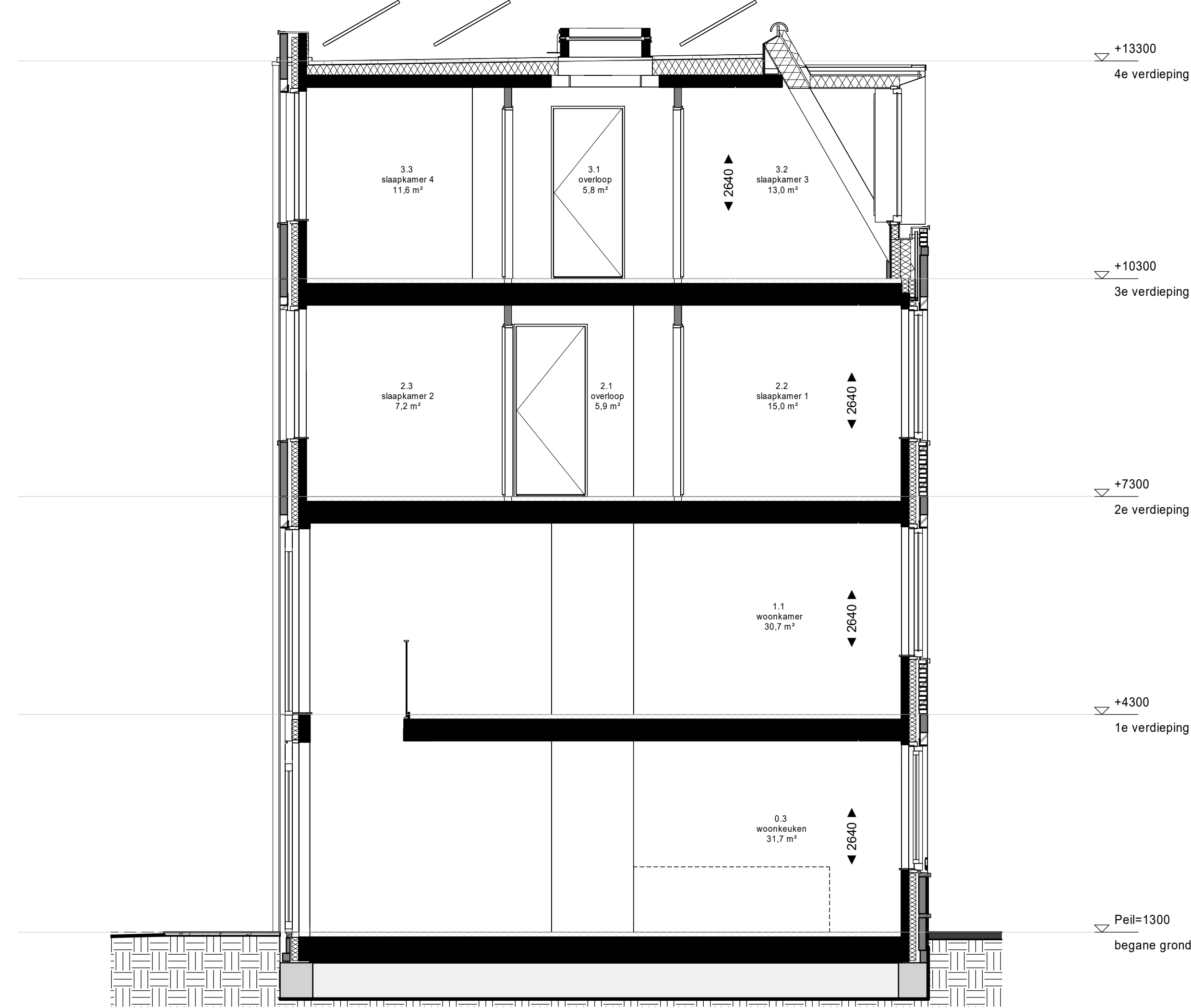
doorsnede
