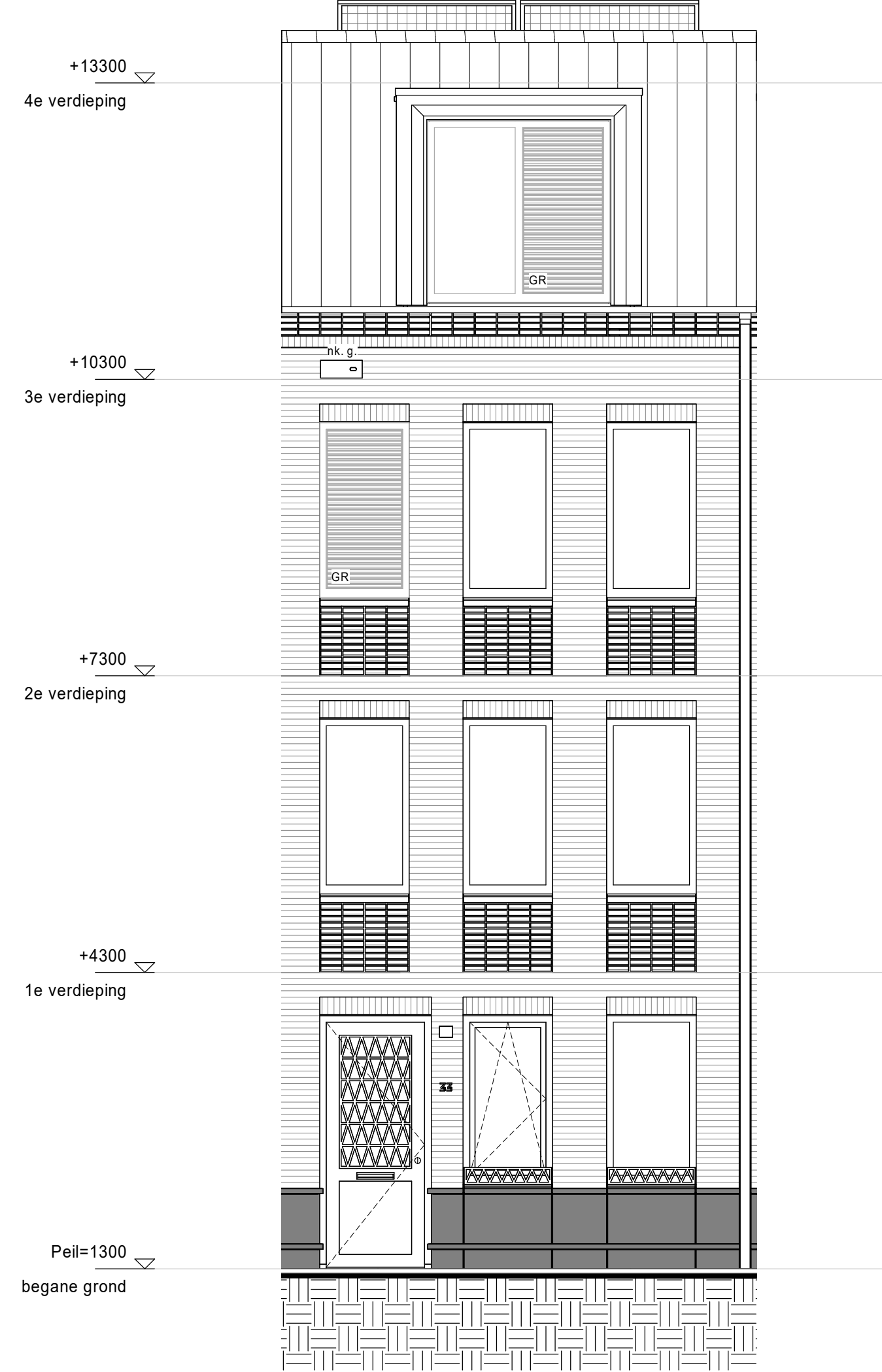
voorgevel
