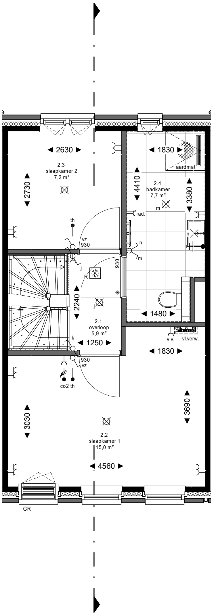
2e verdieping
