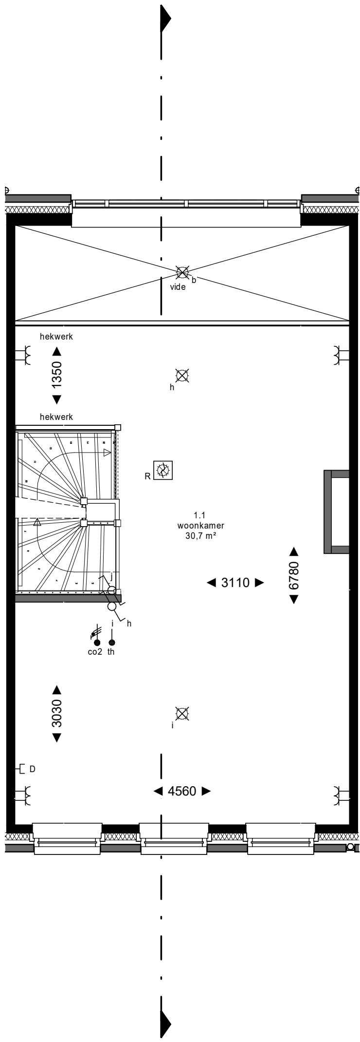
1e verdieping
