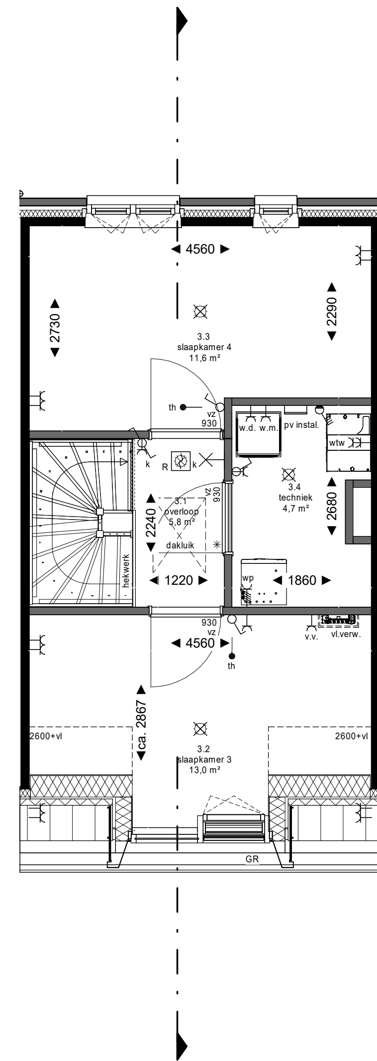
3e verdieping
