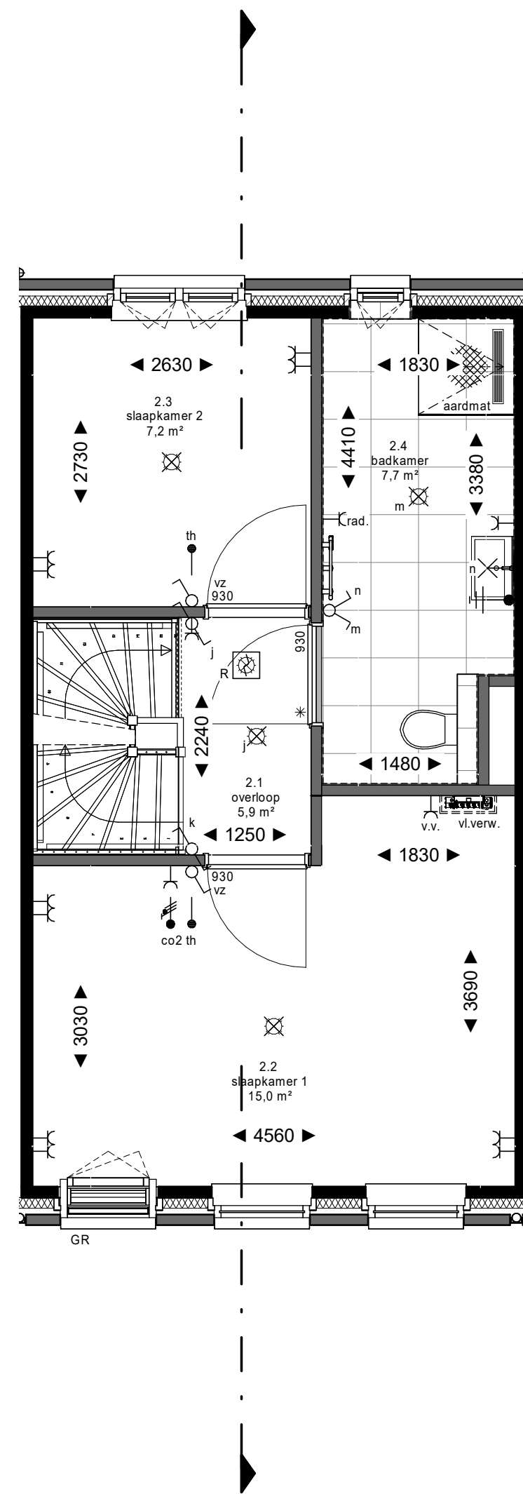
2e verdieping
