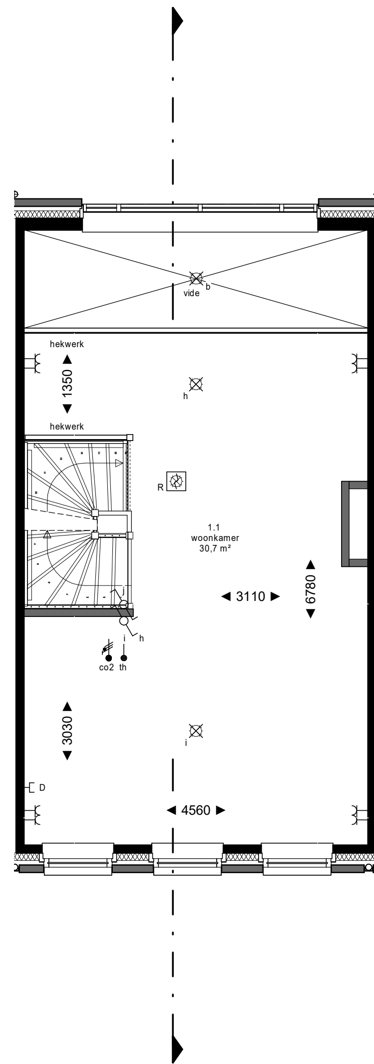
1e verdieping
