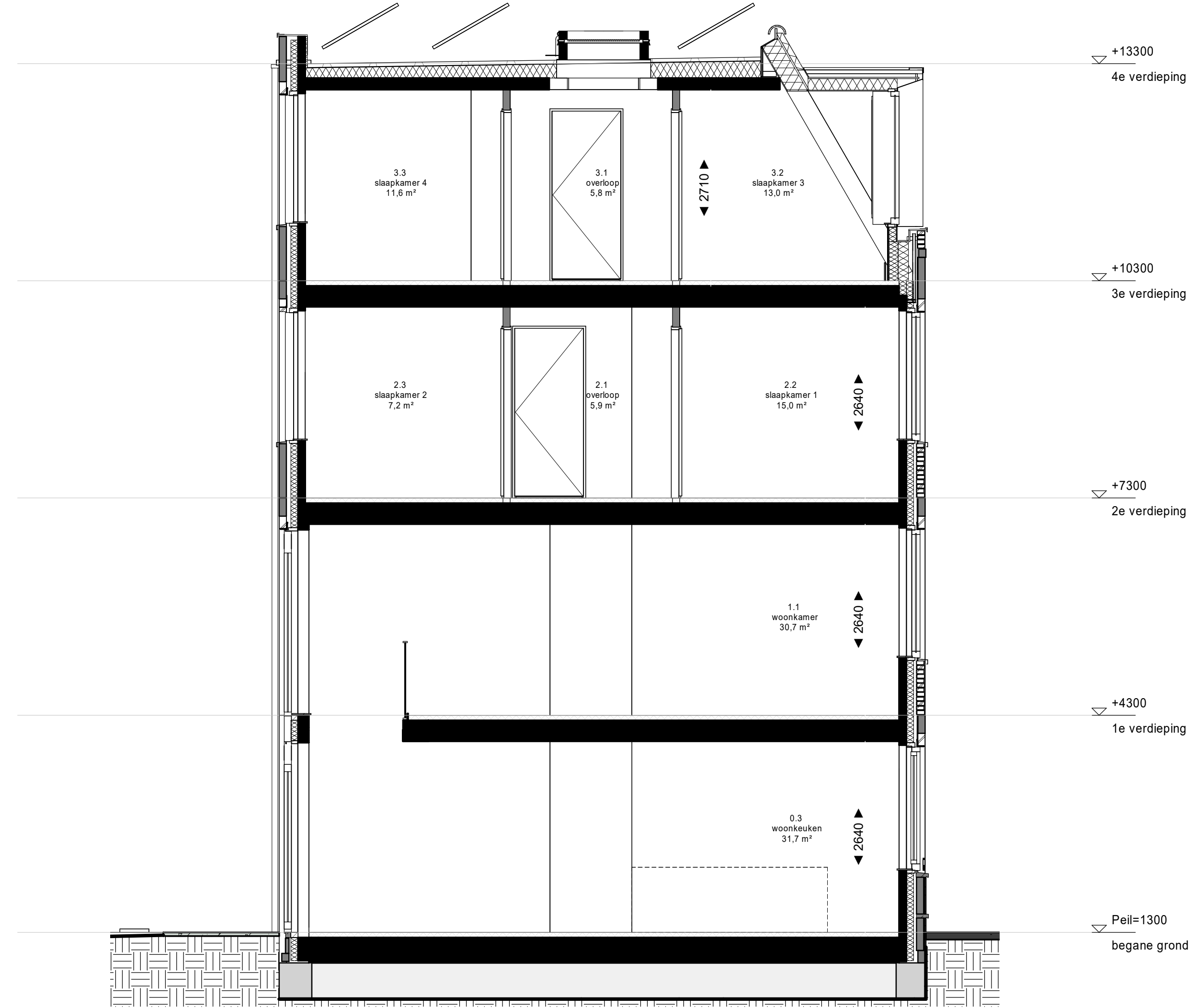
doorsnede
