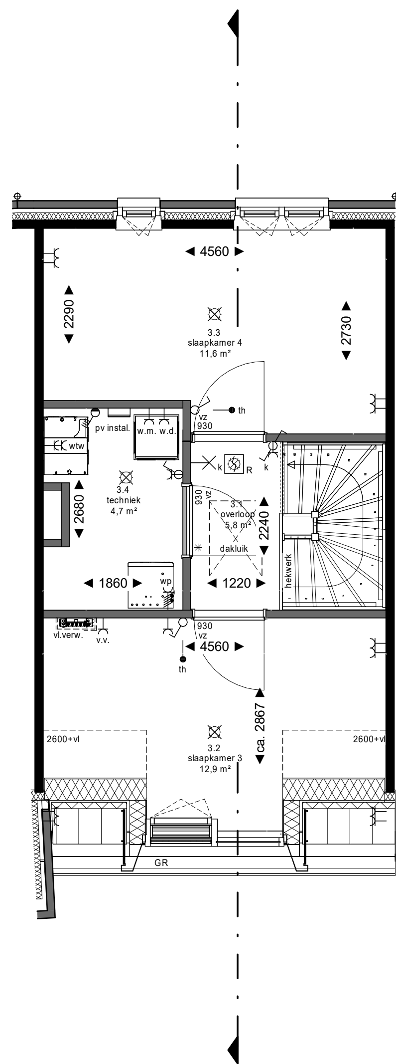
3e verdieping
