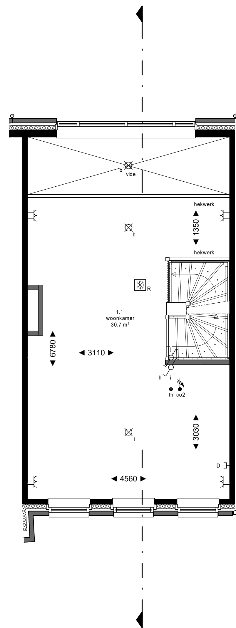
1e verdieping
