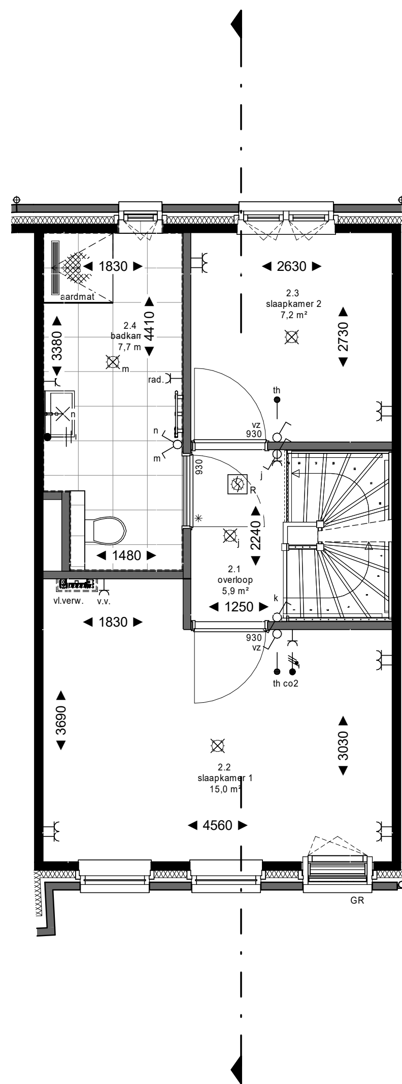
2e verdieping
