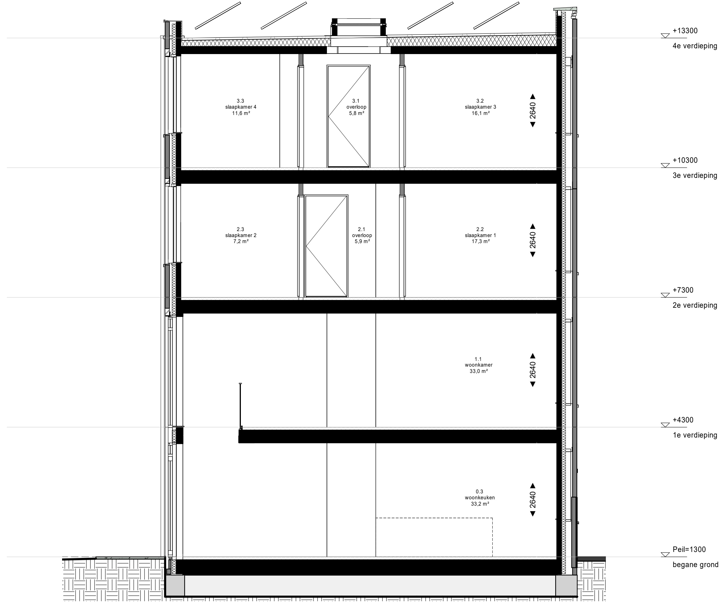
doorsnede
