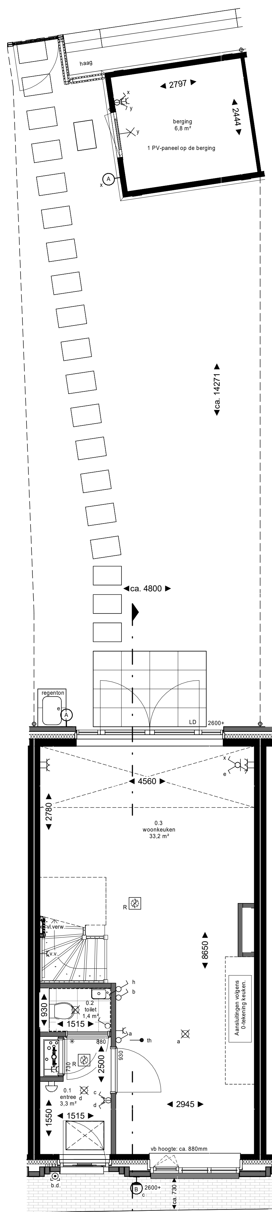
begane grond
