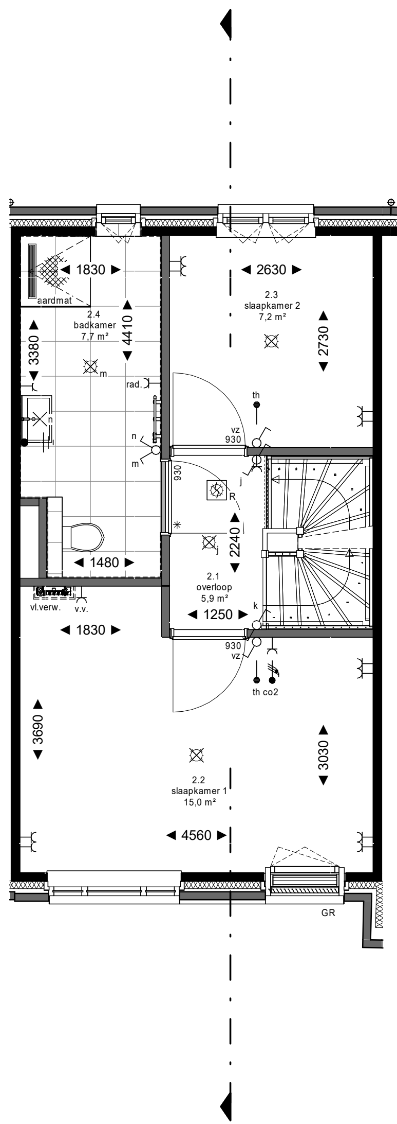
2e verdieping
