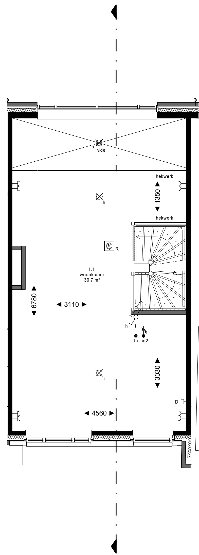
1e verdieping
