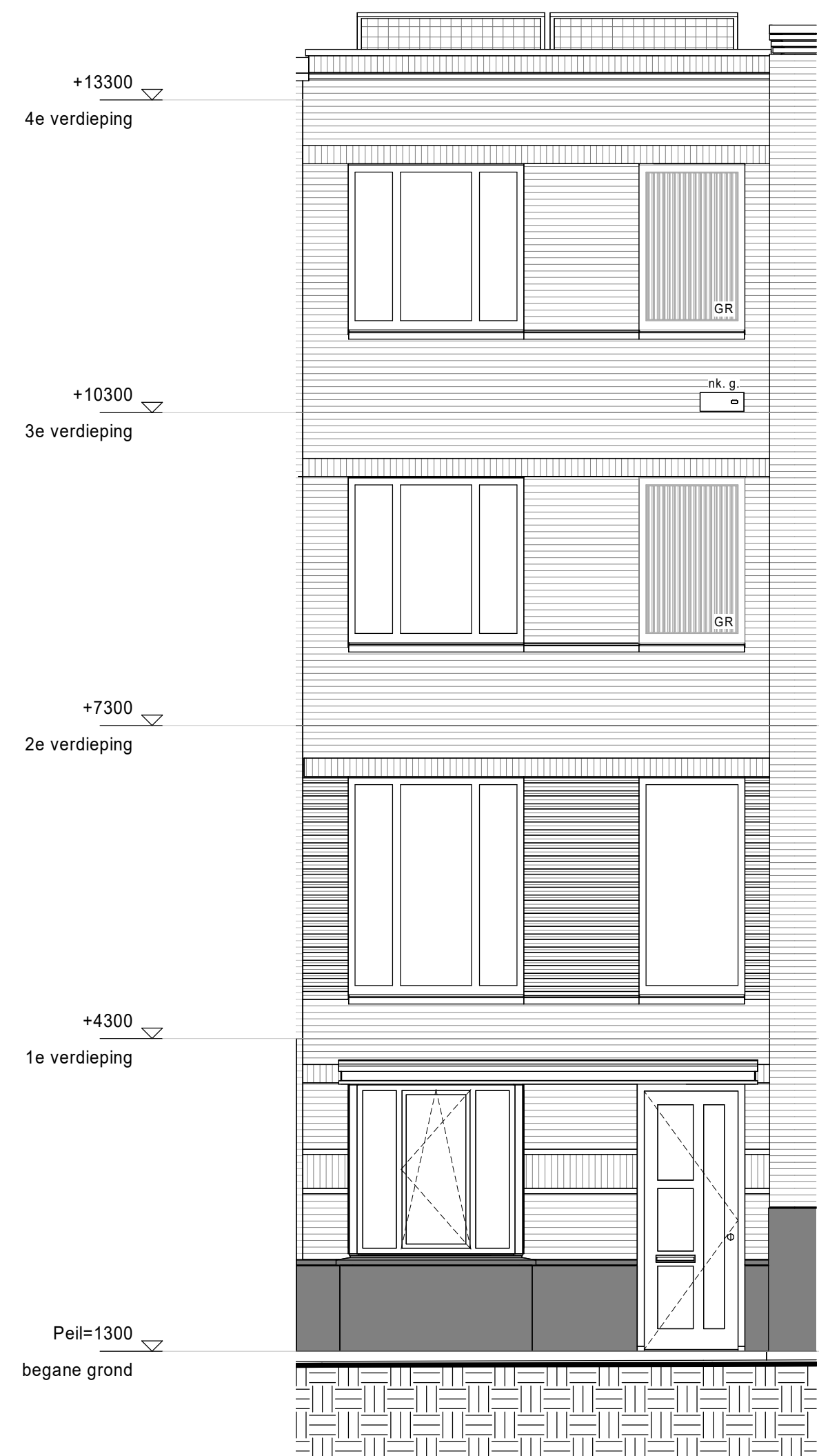
voorgevel
