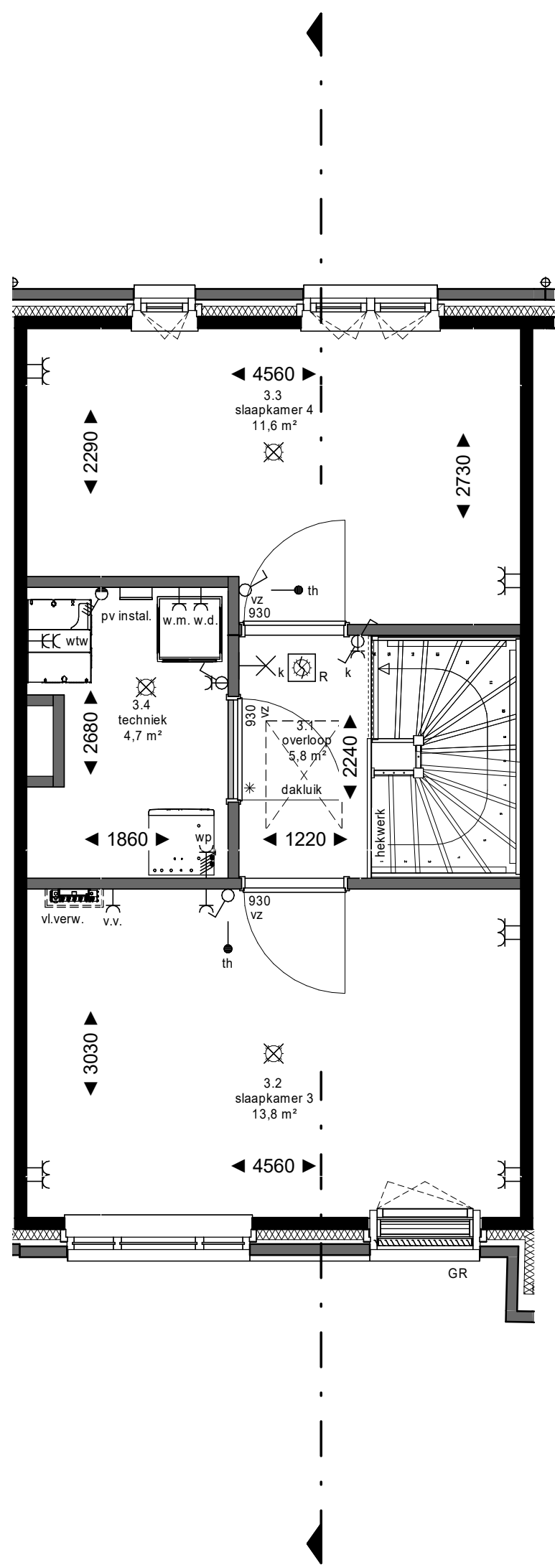
3e verdieping
