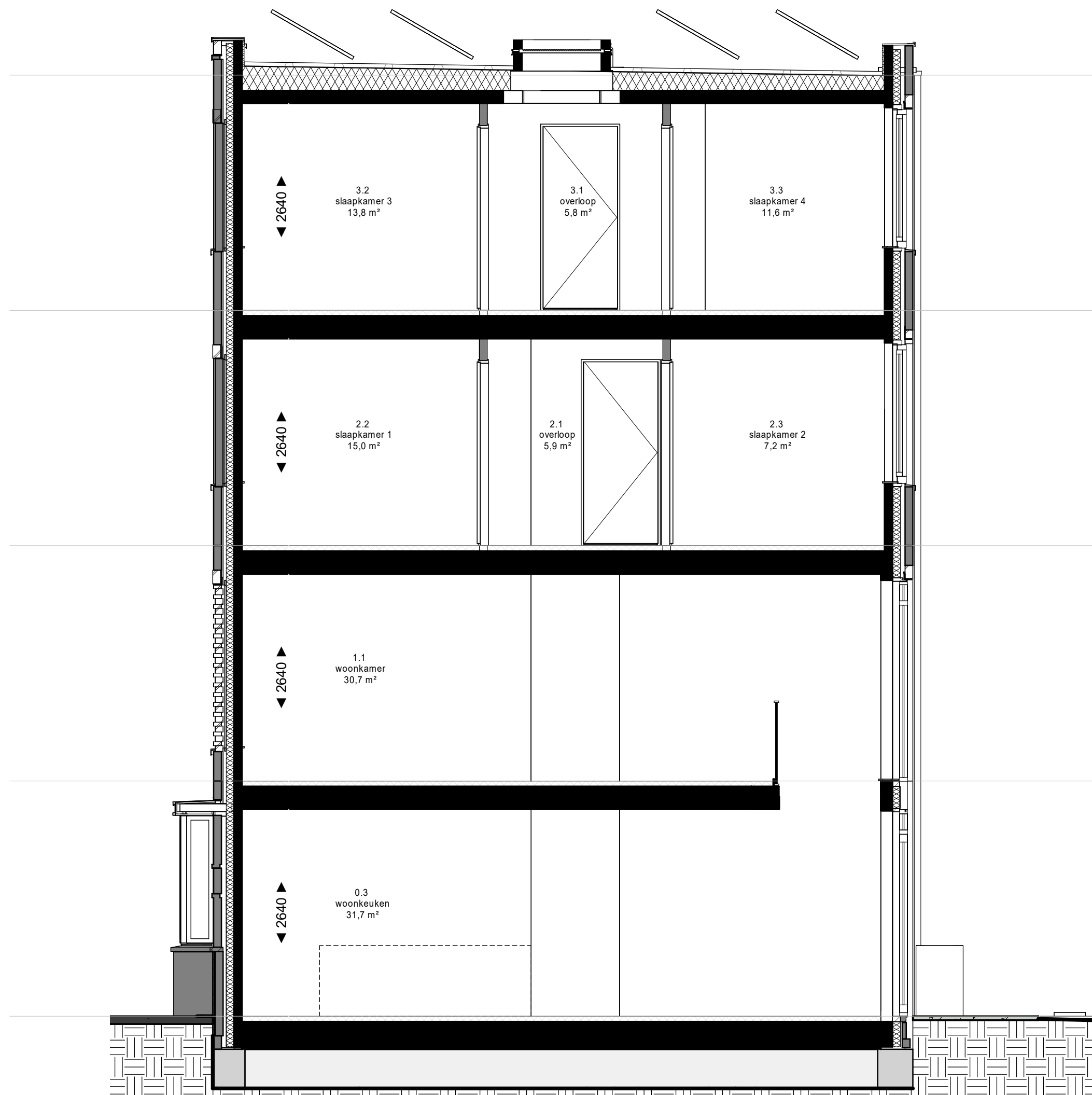
doorsnede
