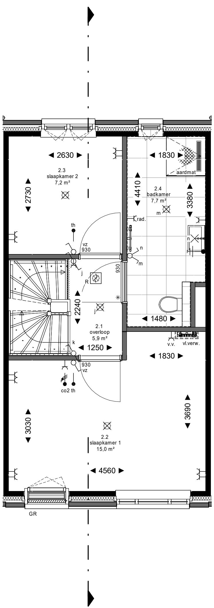
2e verdieping
