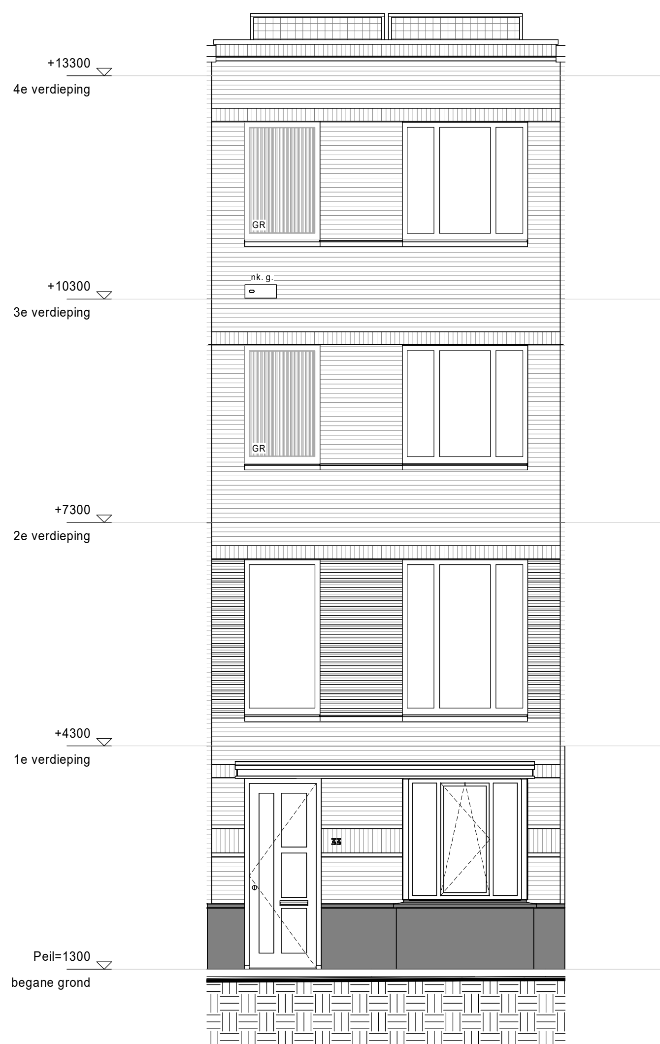
voorgevel
