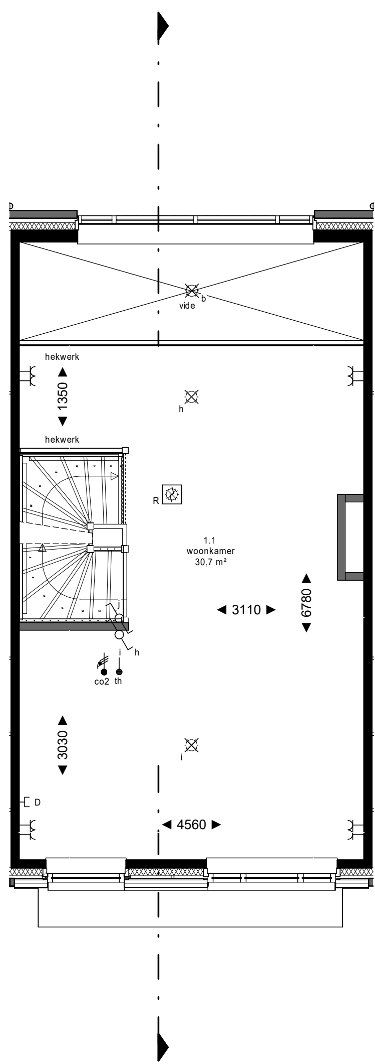
1e verdieping
