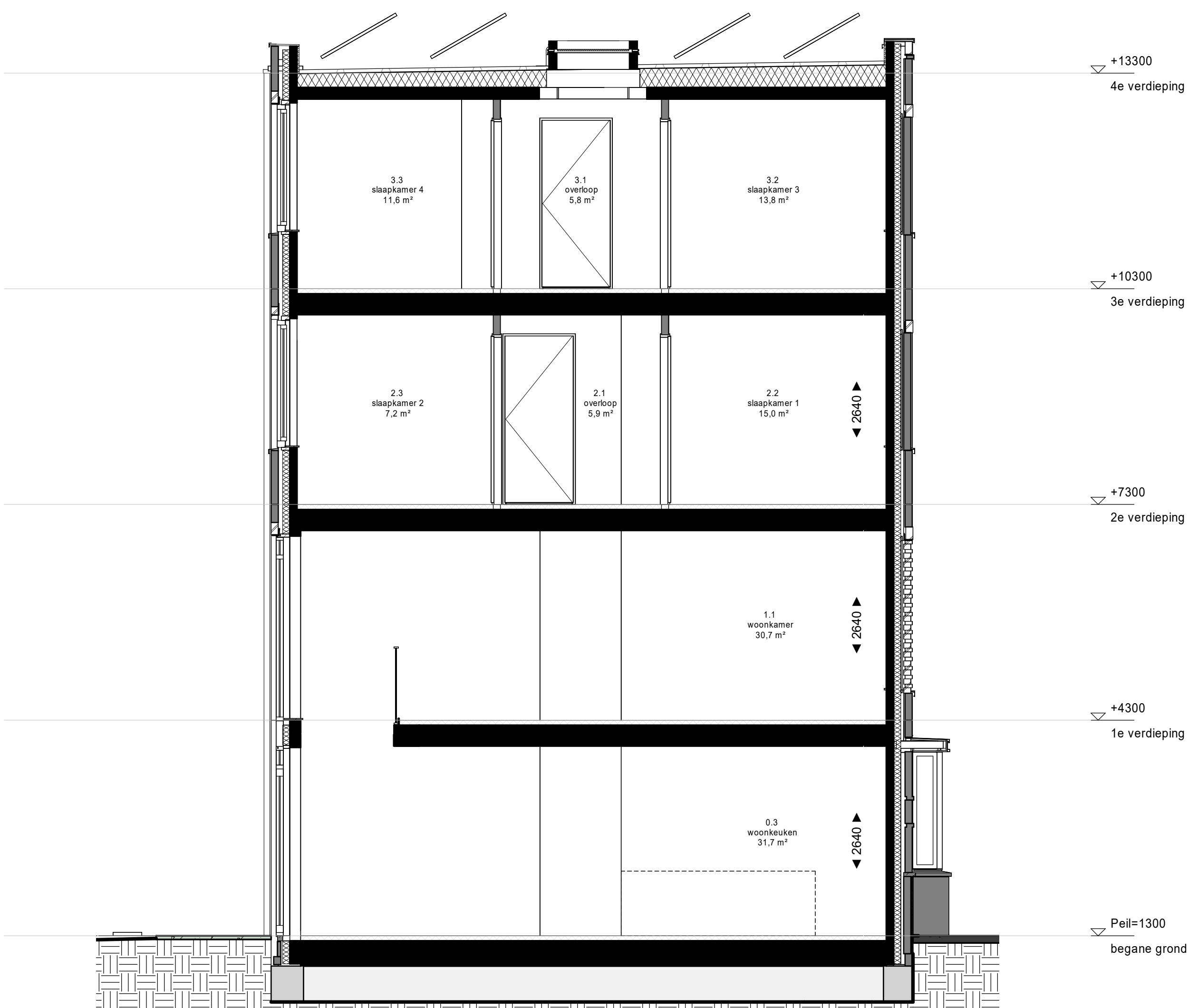
doorsnede
