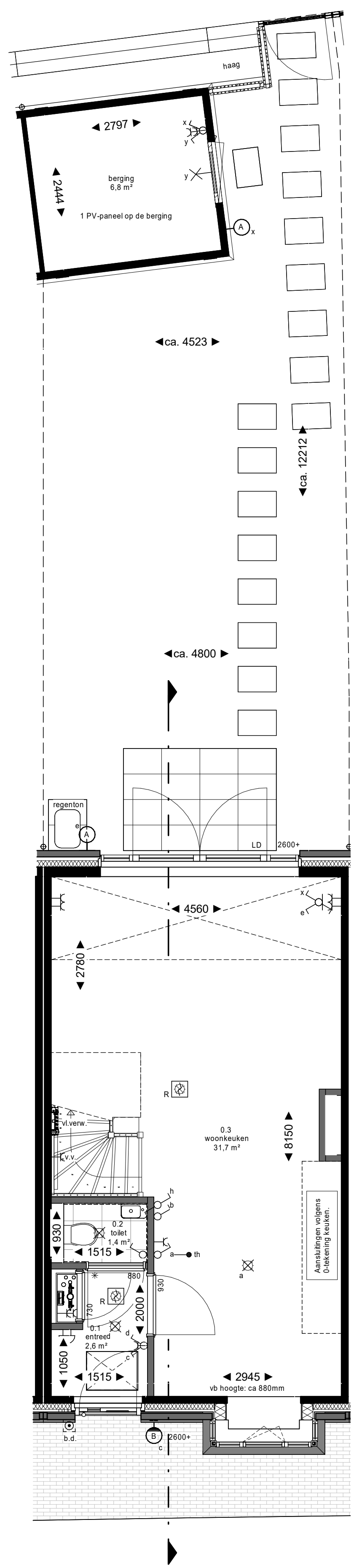
begane grond
