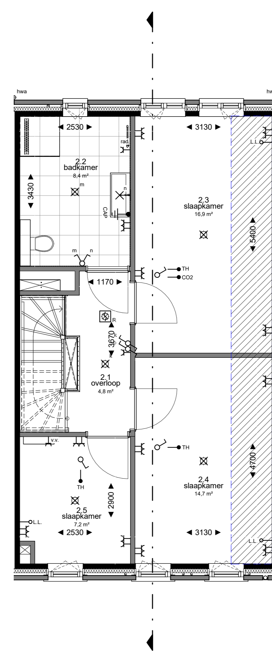
2e verdieping 1 : 50
