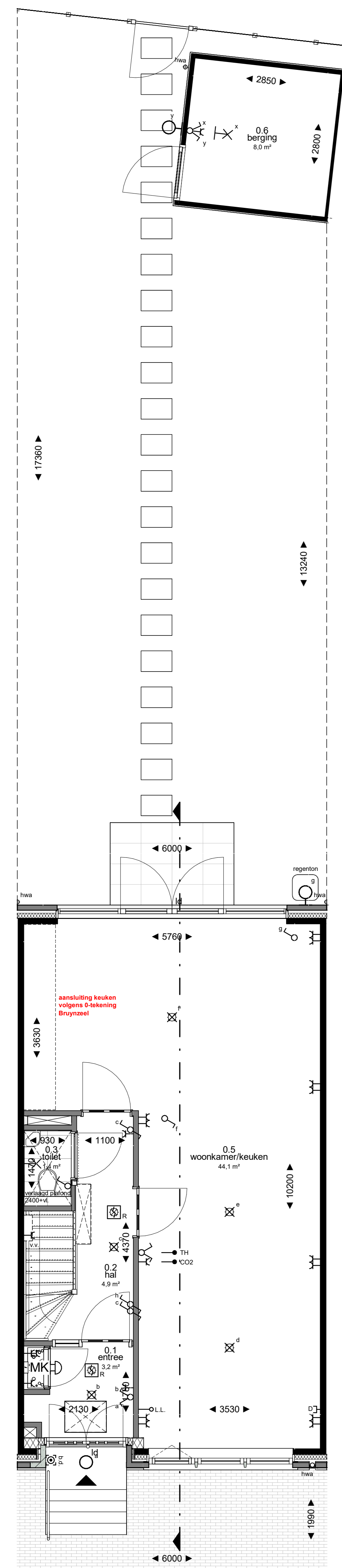
begane grond 1 : 50
