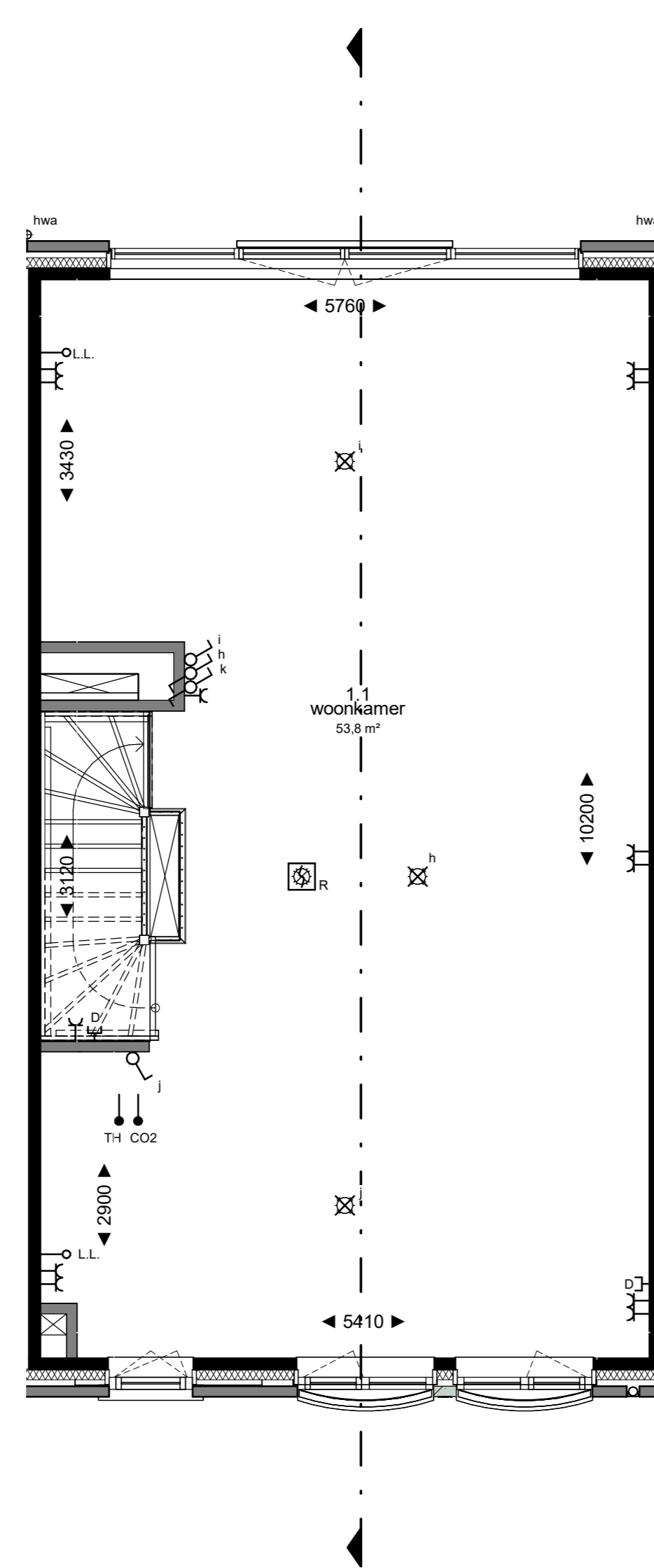
1e verdieping 1 : 50
