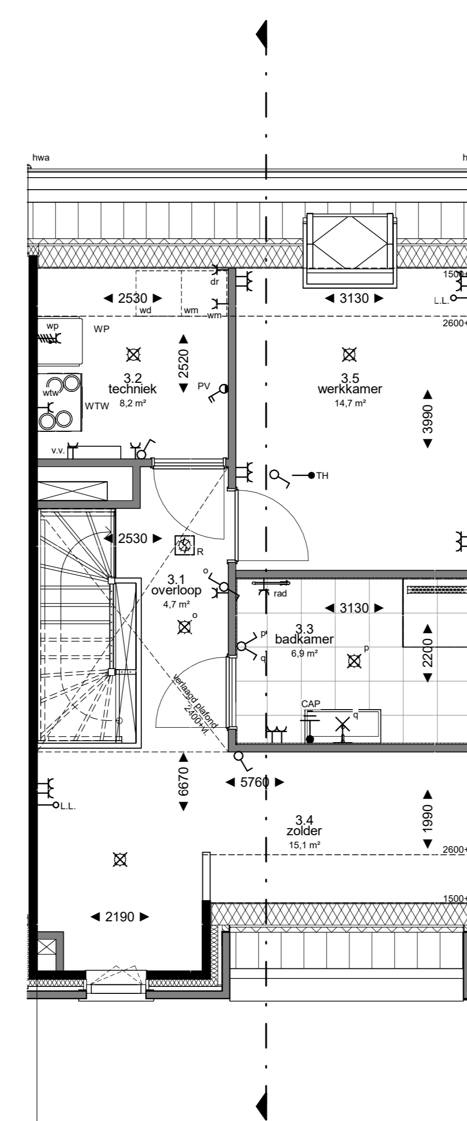
3e verdieping 1 : 50
