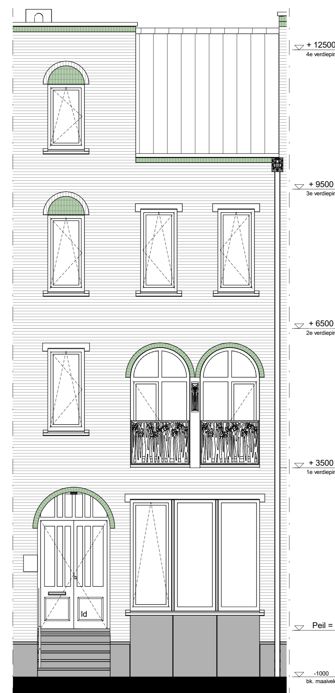
voorgevel 1 : 50
