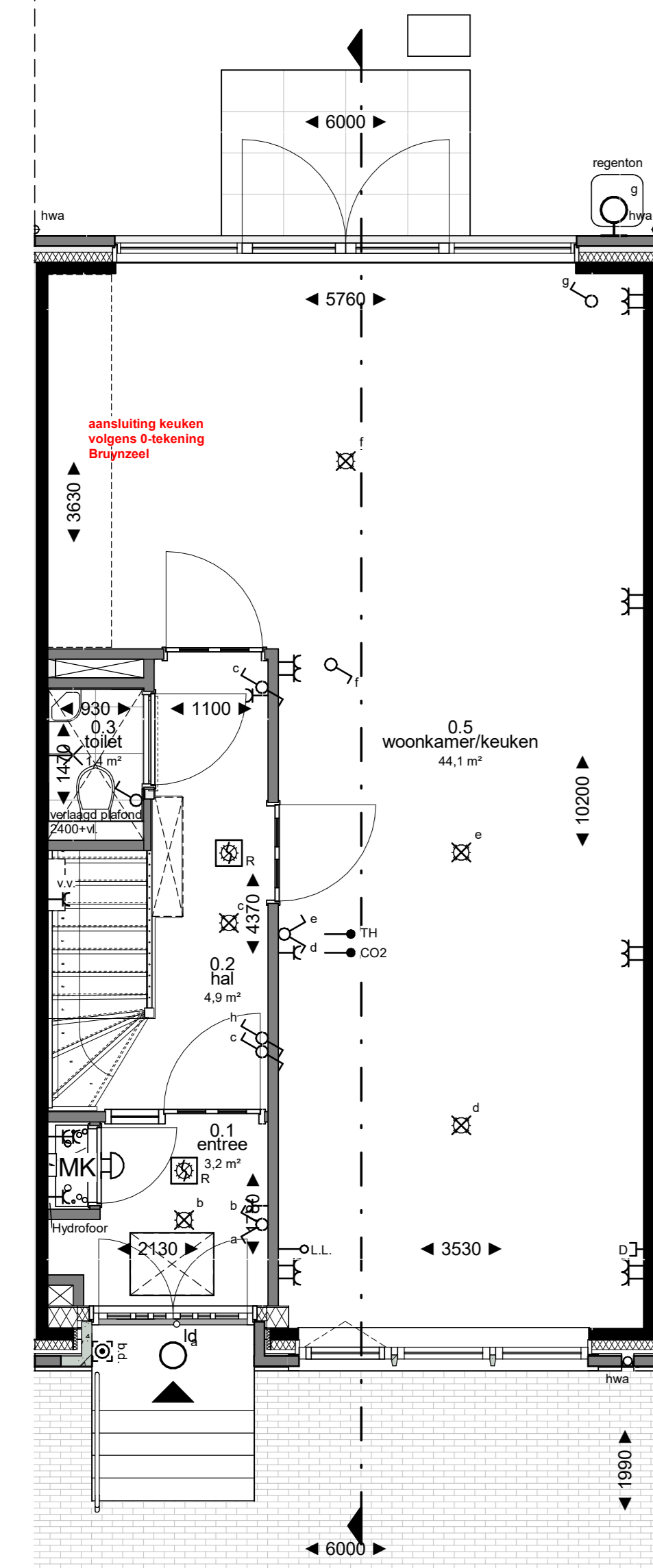
begane grond 1 : 50
