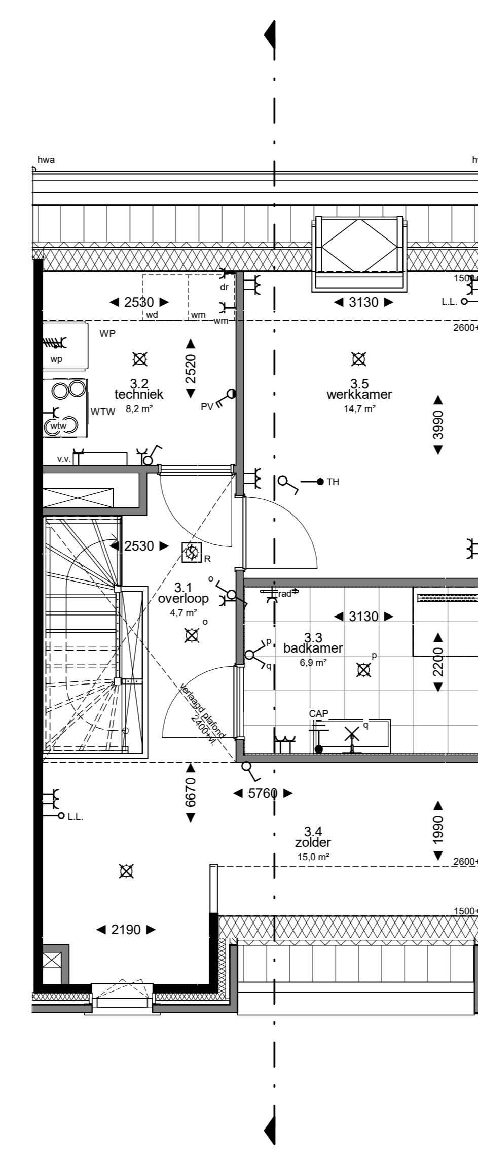
3e verdieping 1 : 50
