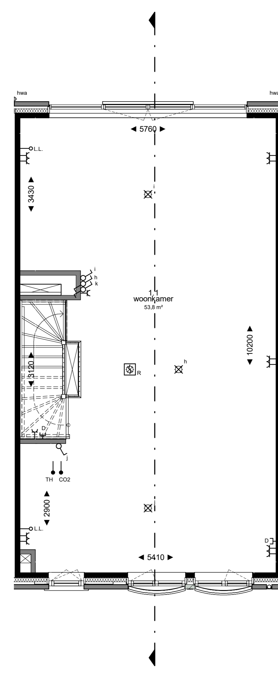
1e verdieping 1 : 50
