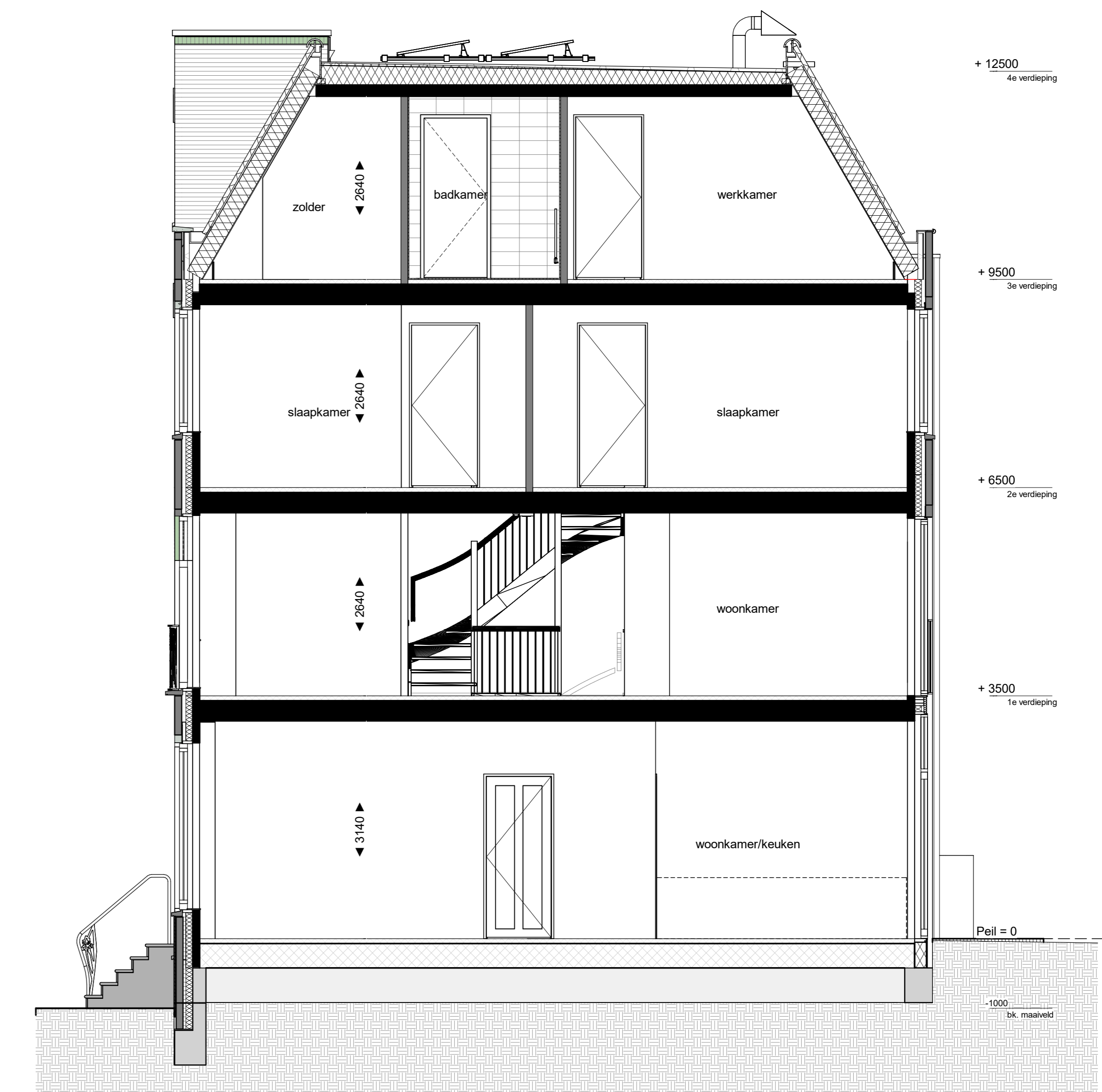
doorsnede A 1 : 50
