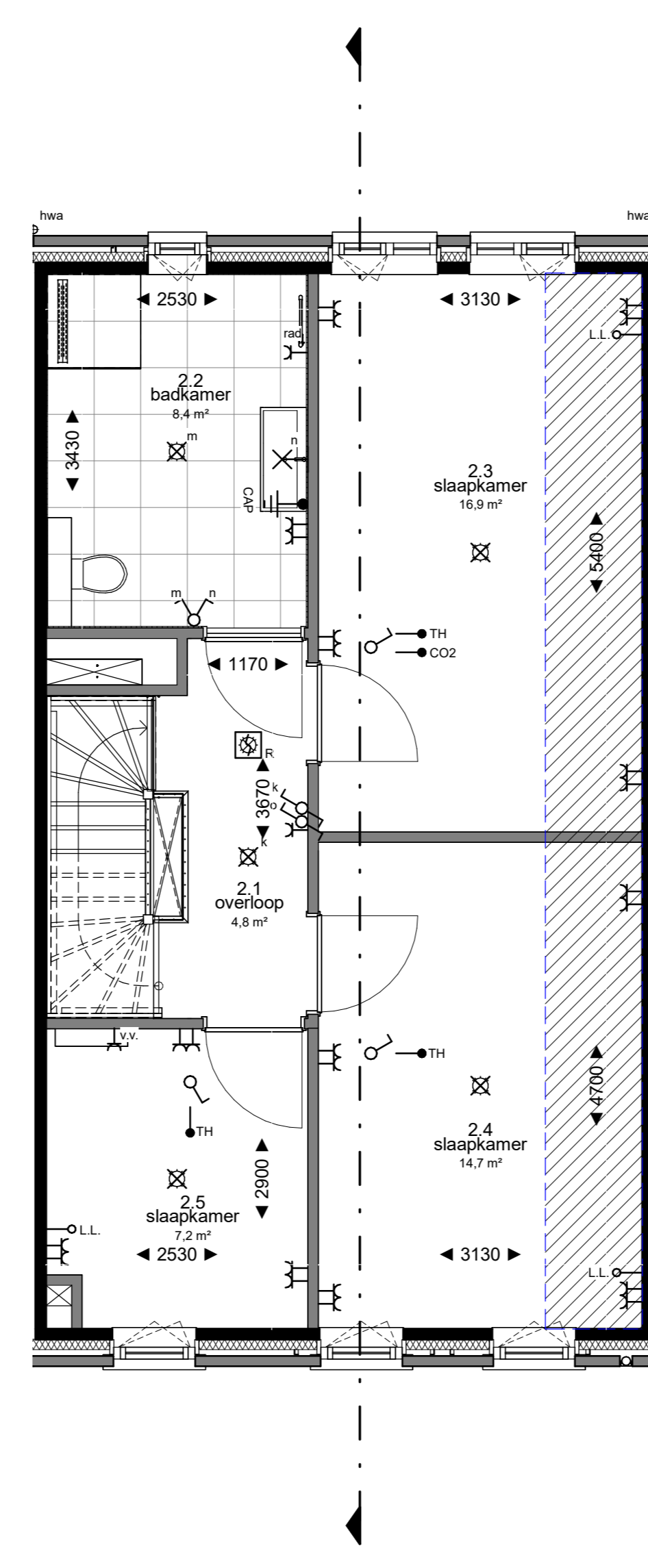
2e verdieping 1 : 50
