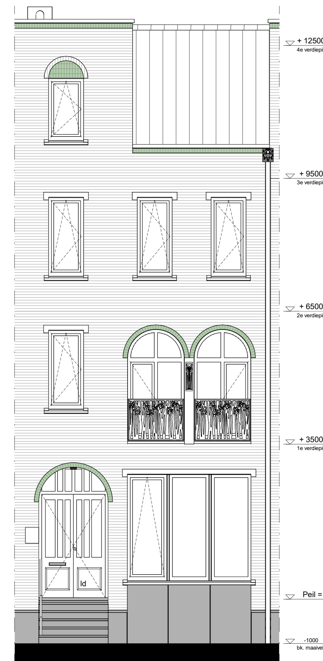
voorgevel 1 : 50
