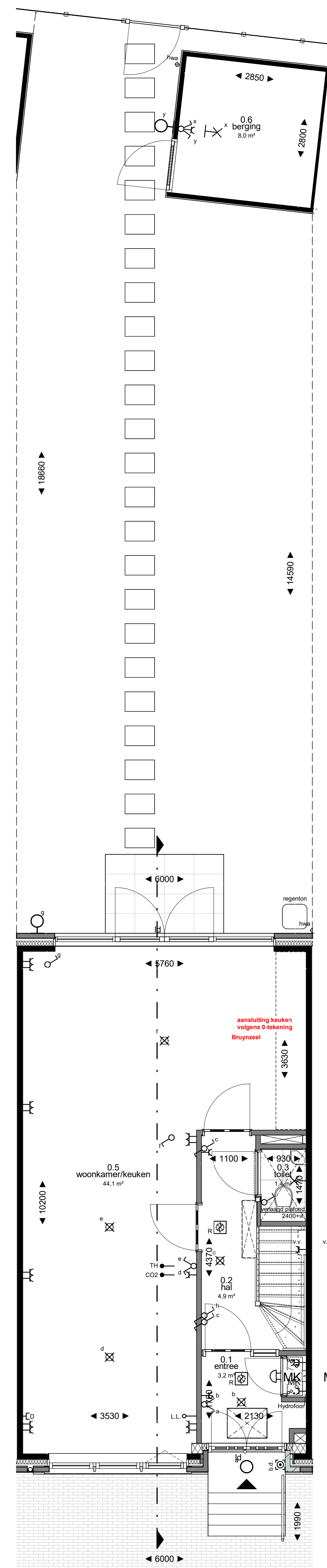
begane grond 1 : 50
