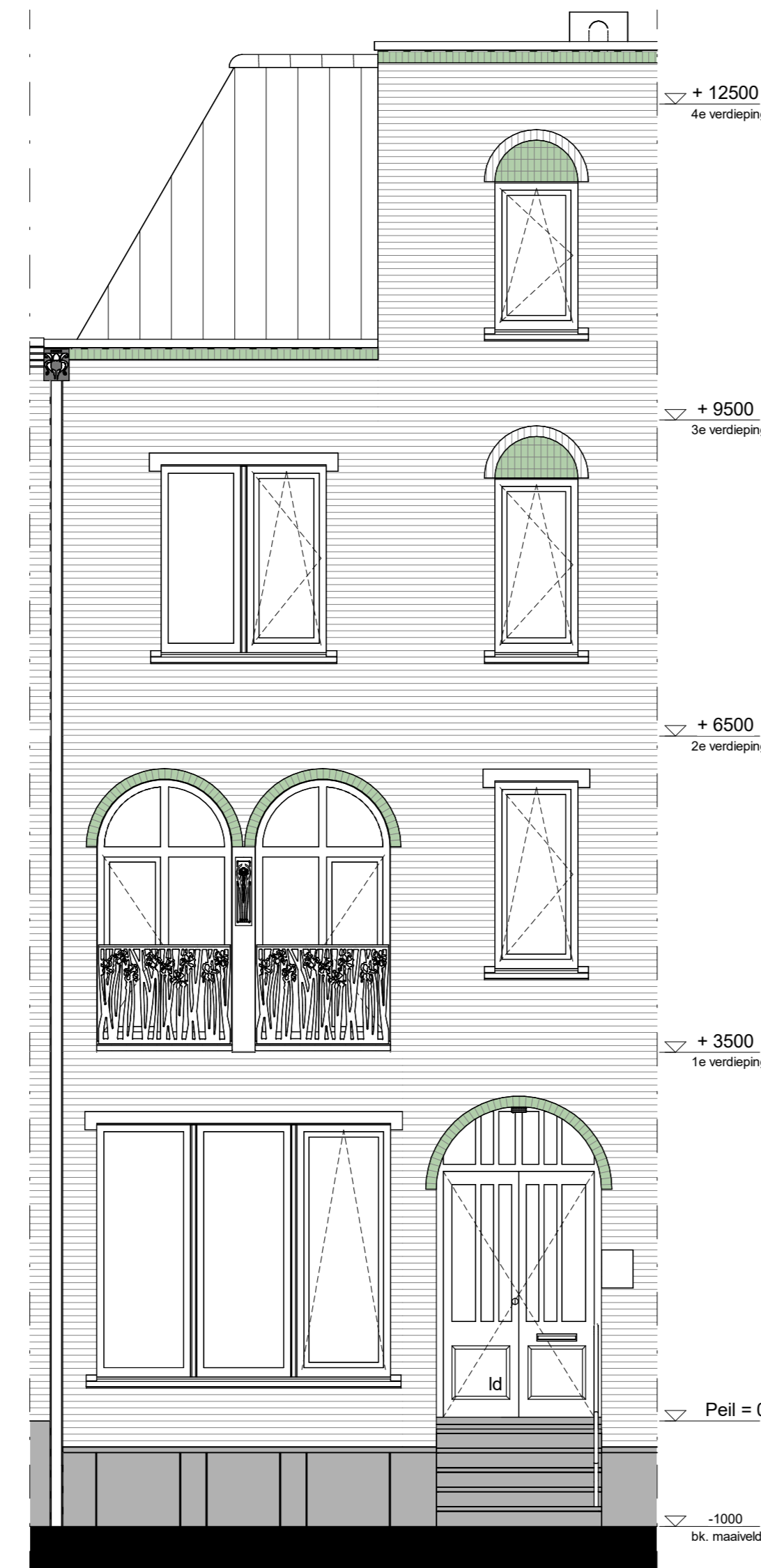
voorgevel 1 : 50
