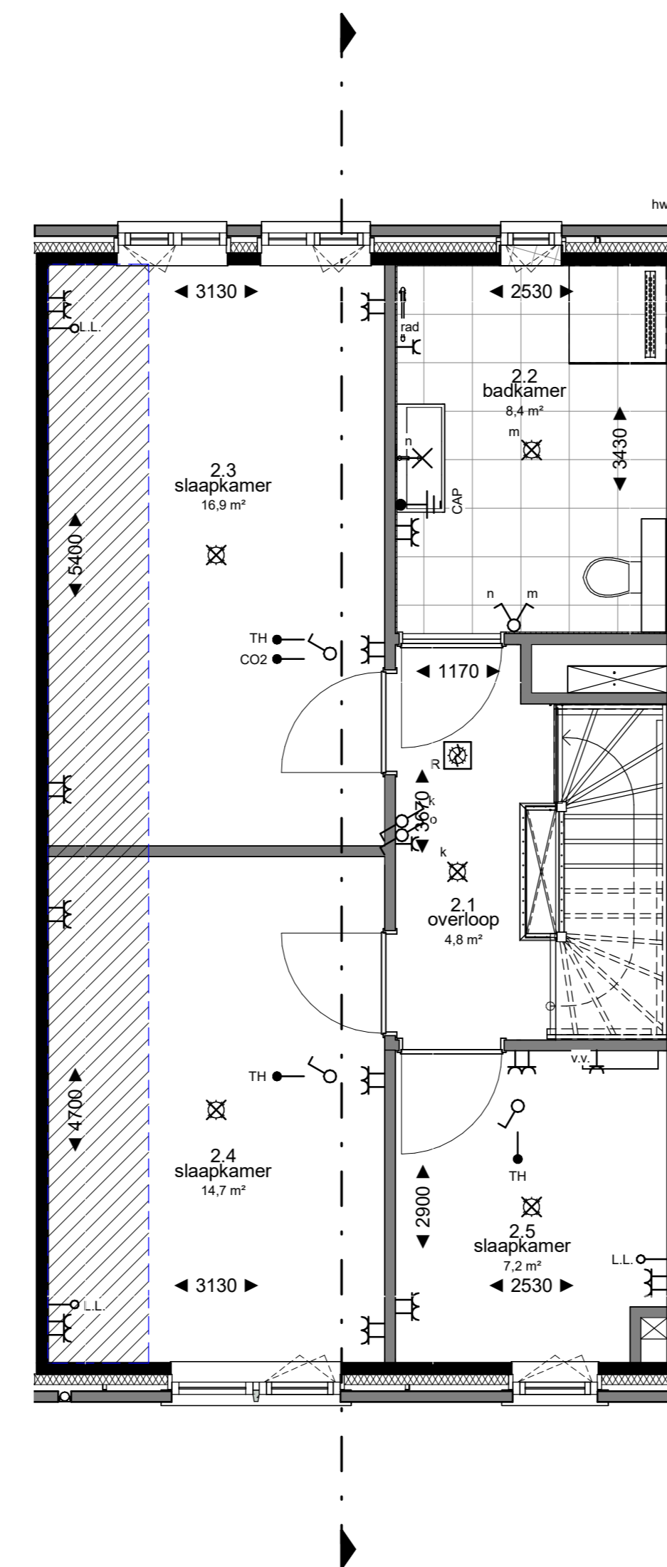
2e verdieping 1 : 50
