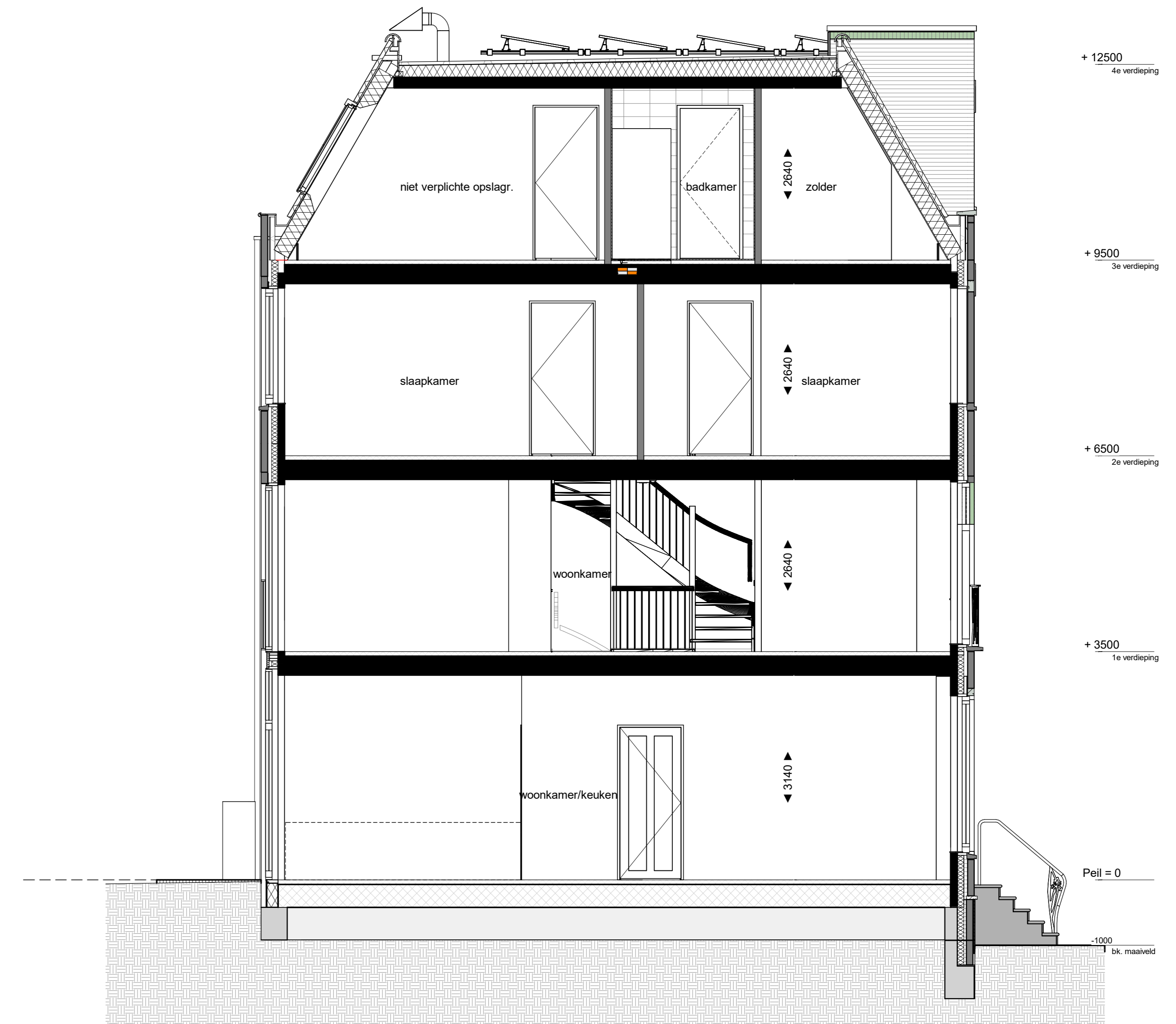
doorsnede A 1 : 50
