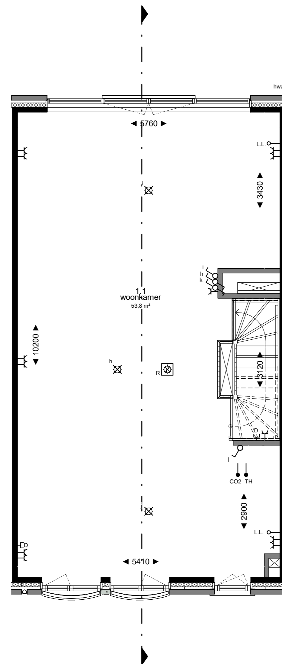
1e verdieping 1 : 50
