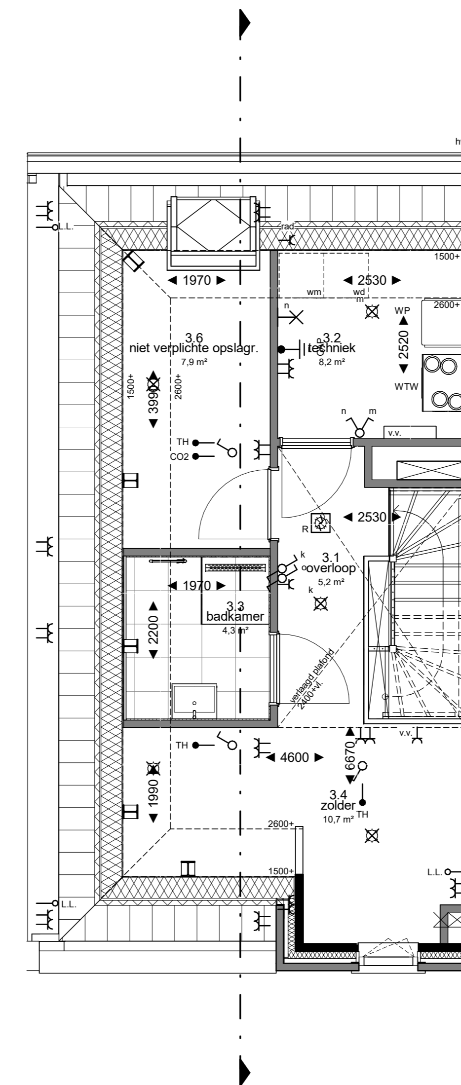
3e verdieping 1 : 50
