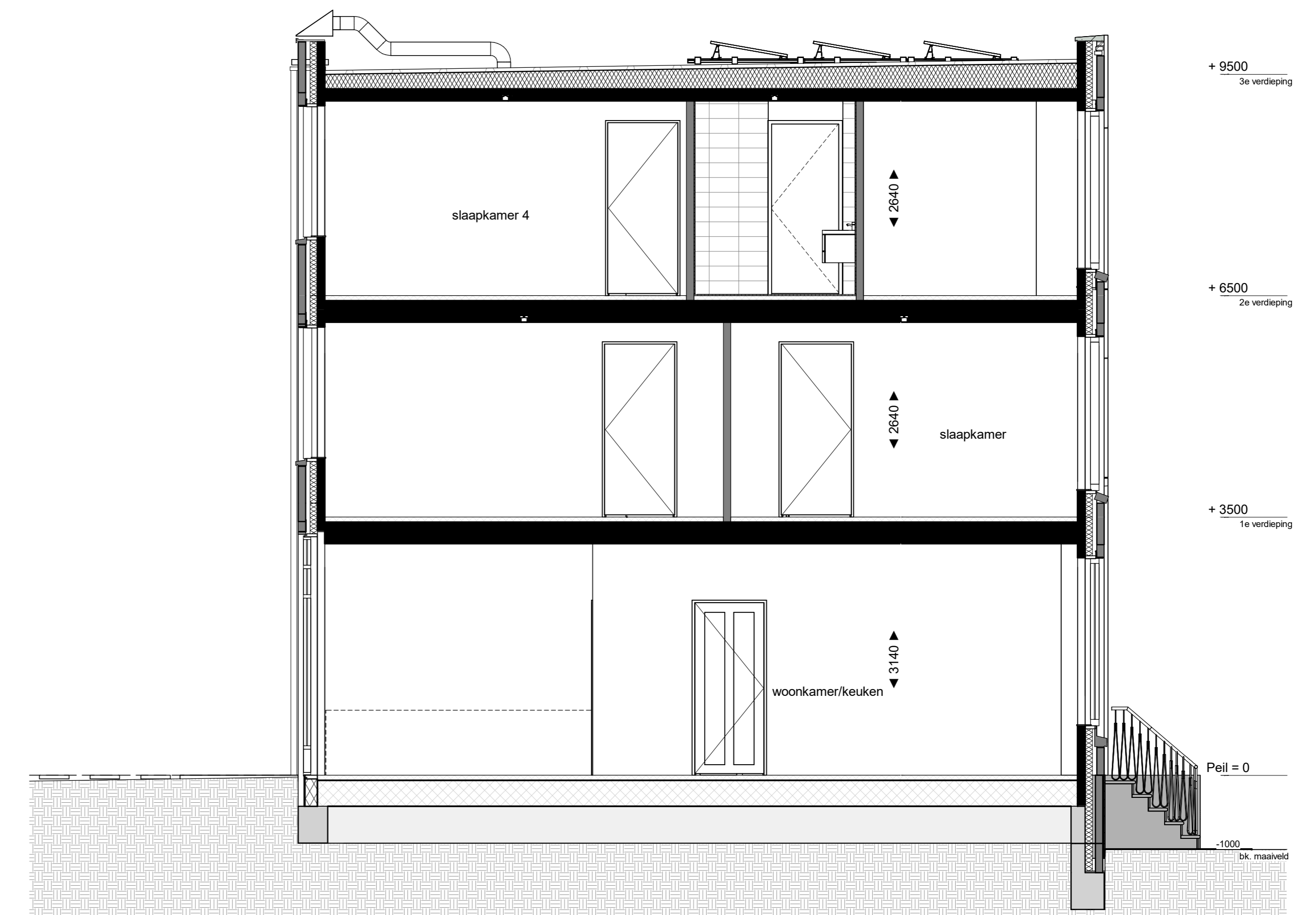
doorsnede A 1 : 50
