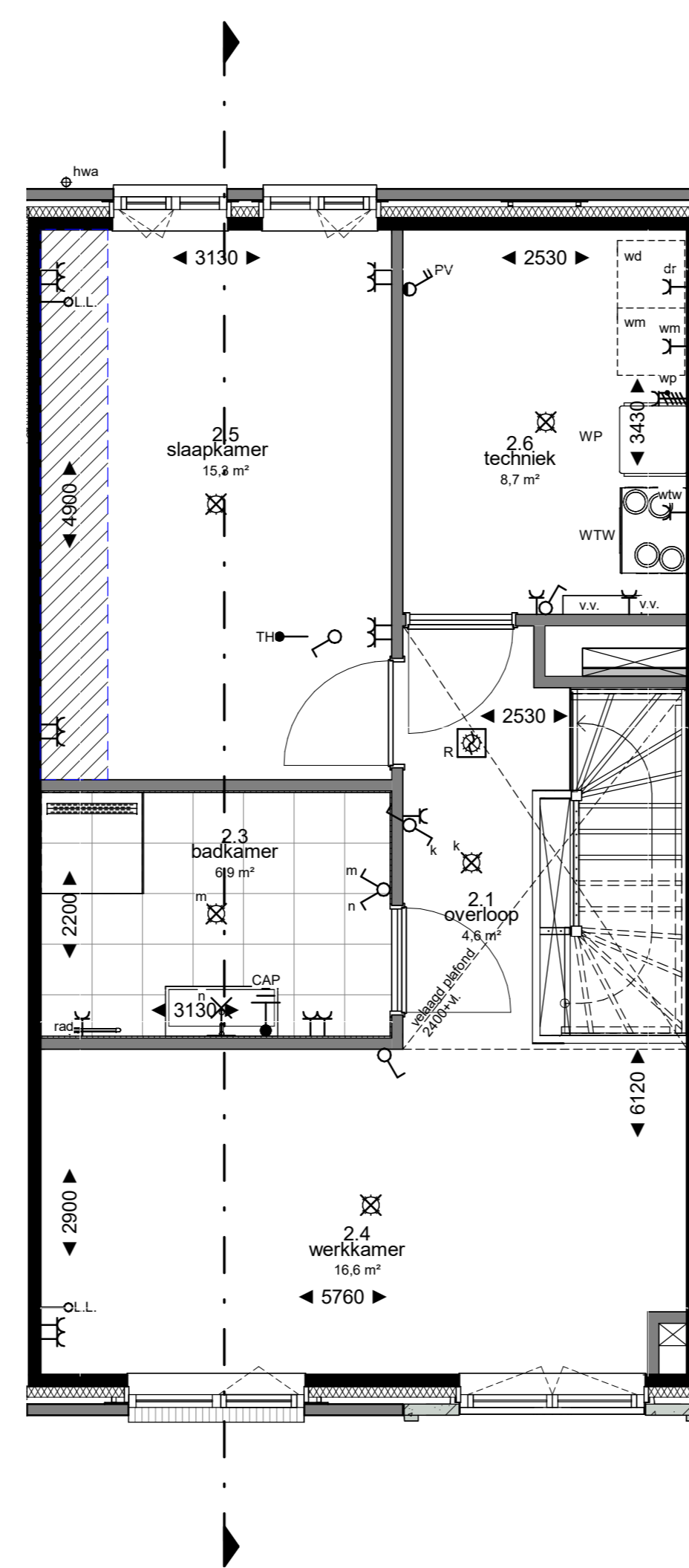
2e verdieping 1 : 50
