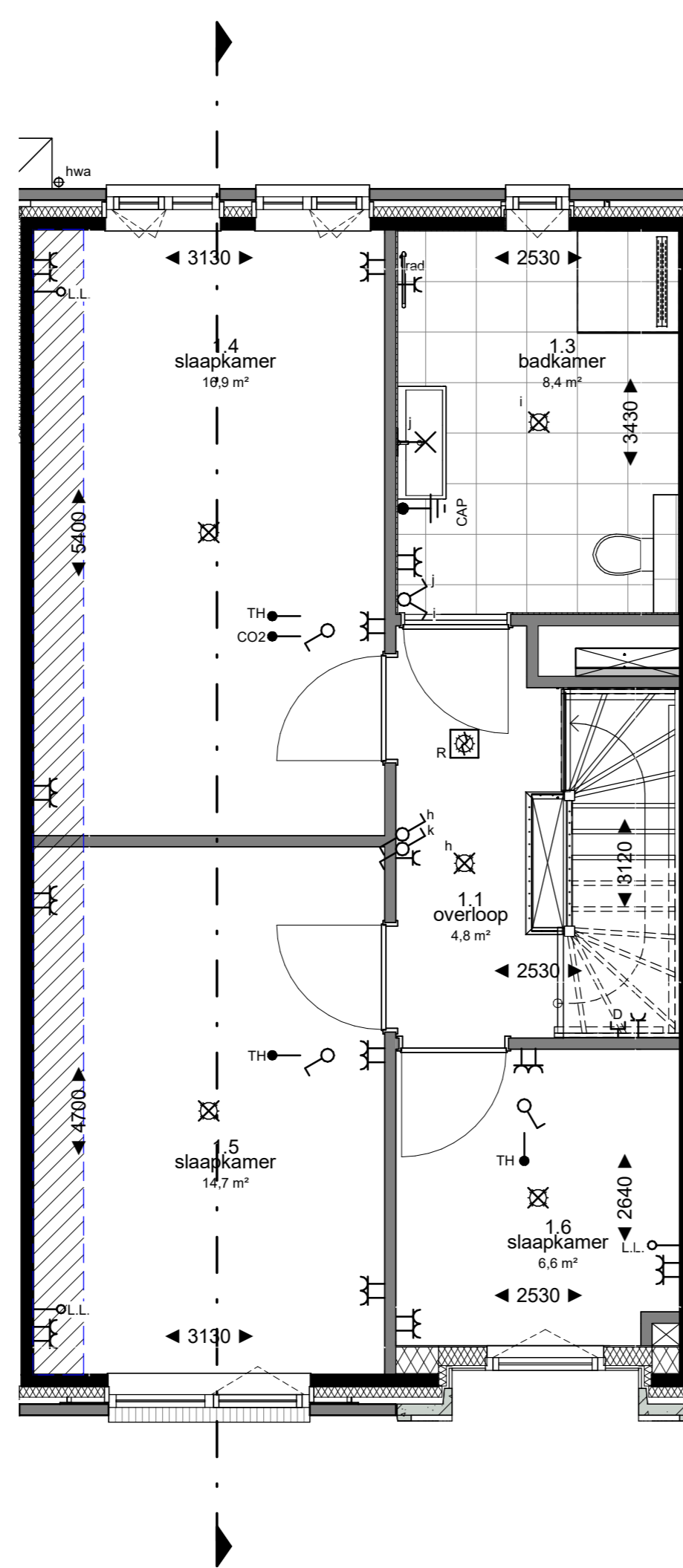
1e verdieping 1 : 50
