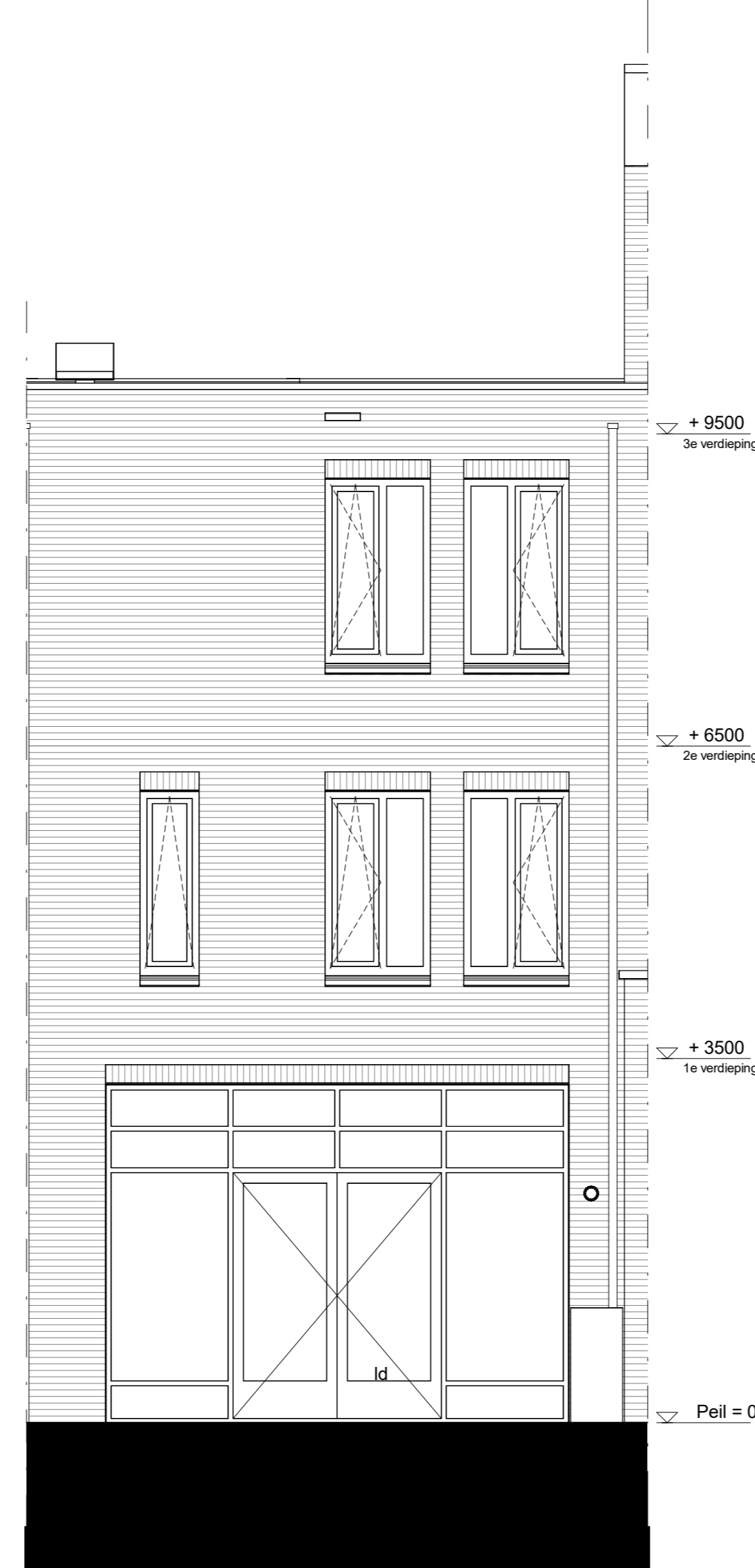
achtergevel 1 : 50
