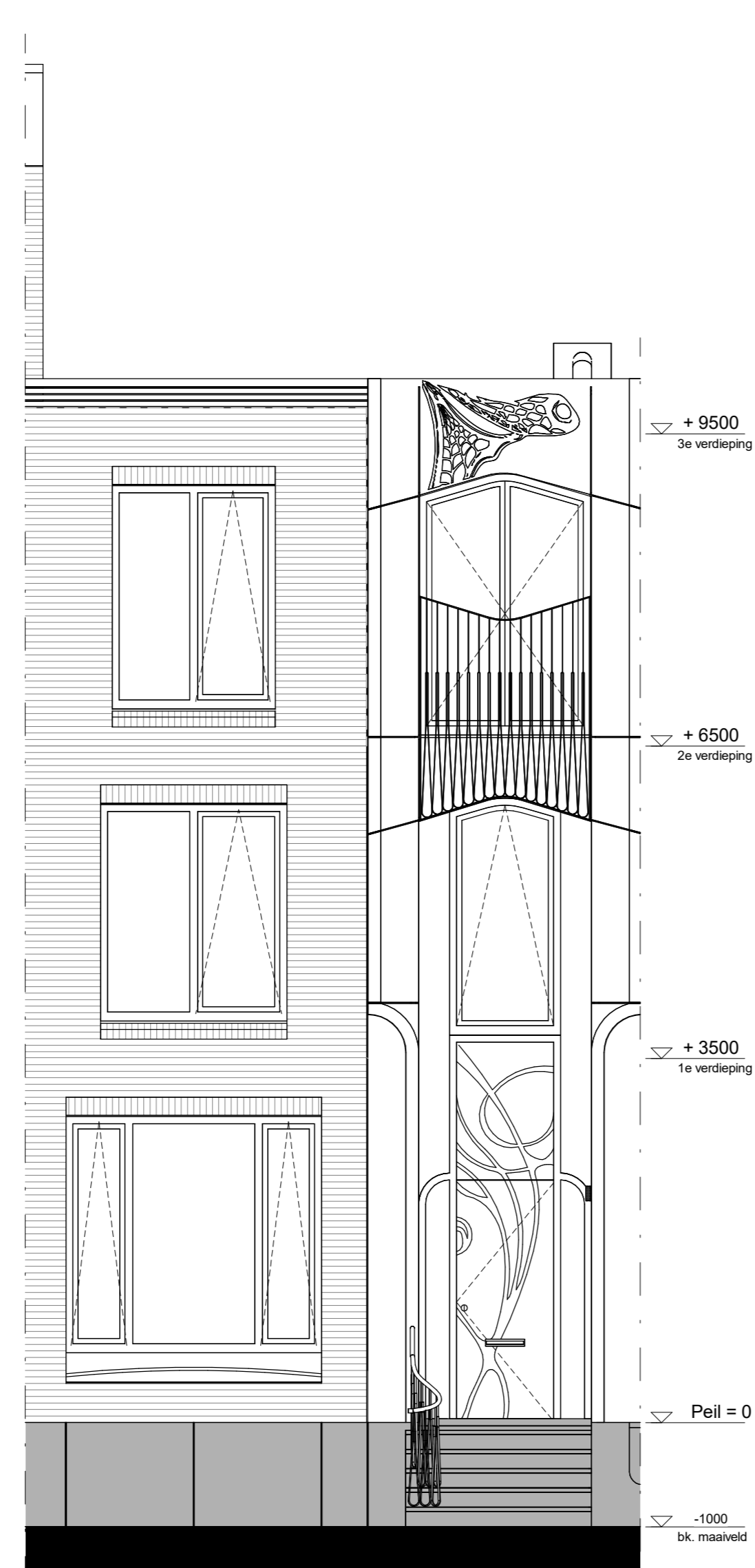
voorgevel 1 : 50
