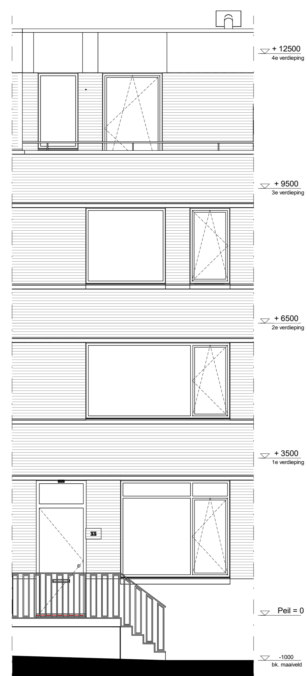
voorgevel 1 : 50
