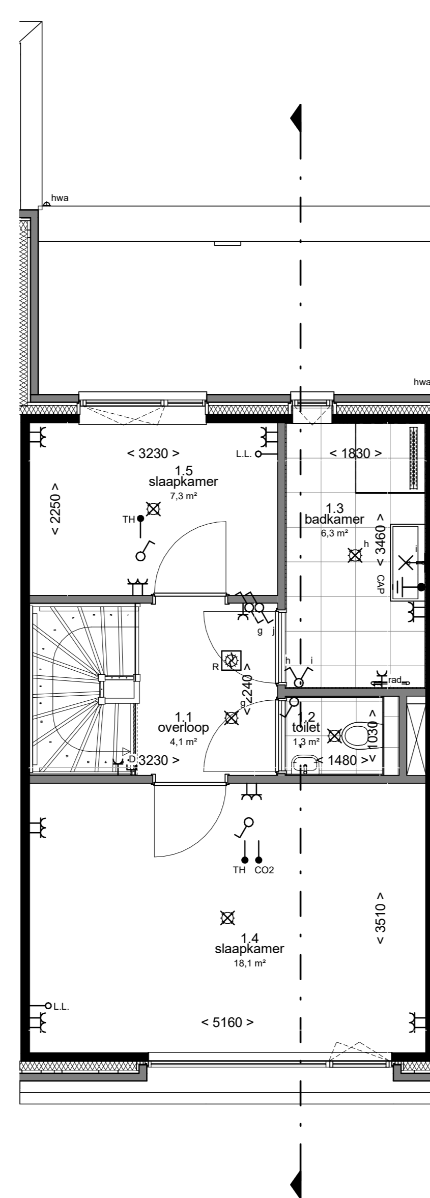
1e verdieping 1 : 50
