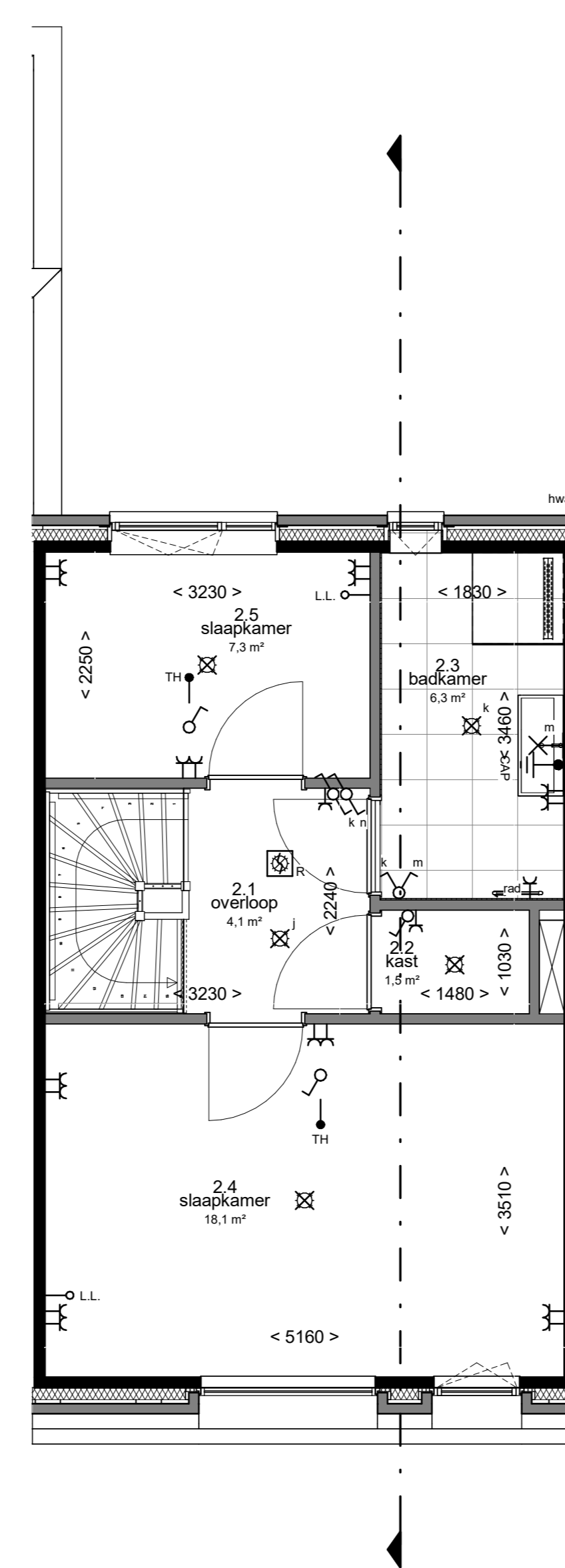
2e verdieping 1 : 50
