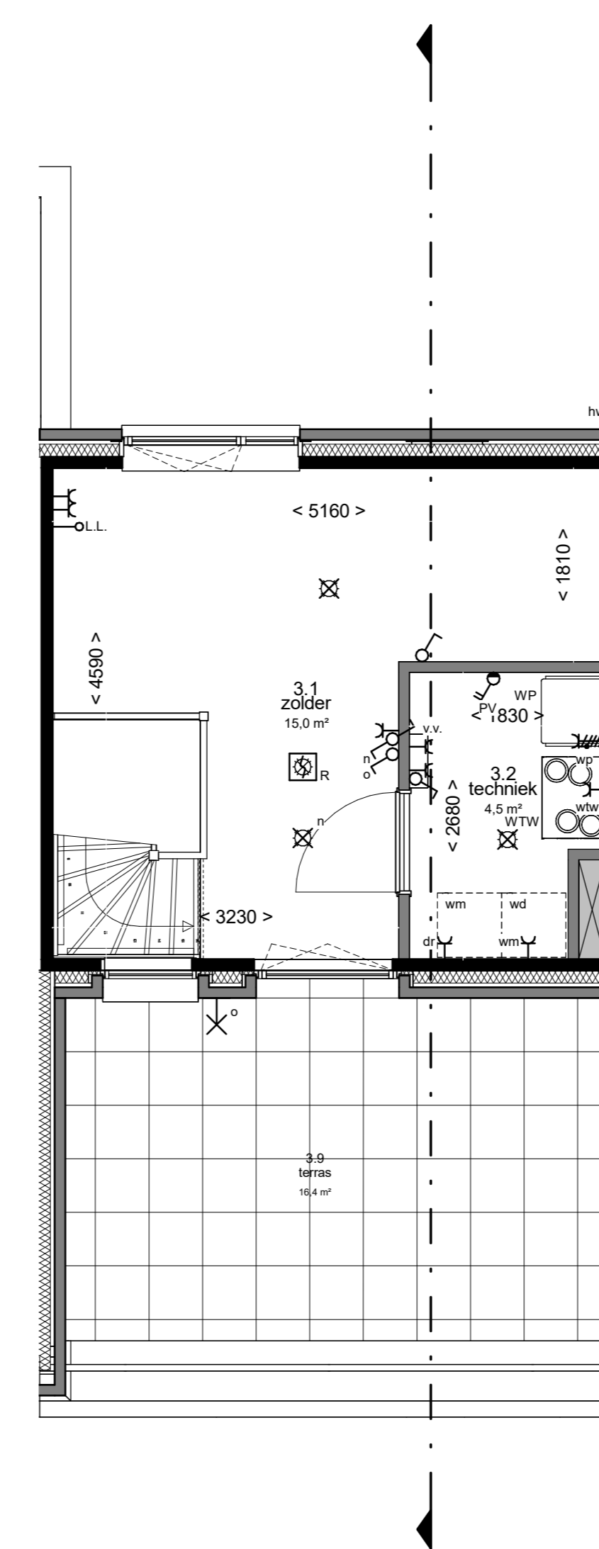
3e verdieping 1 : 50
