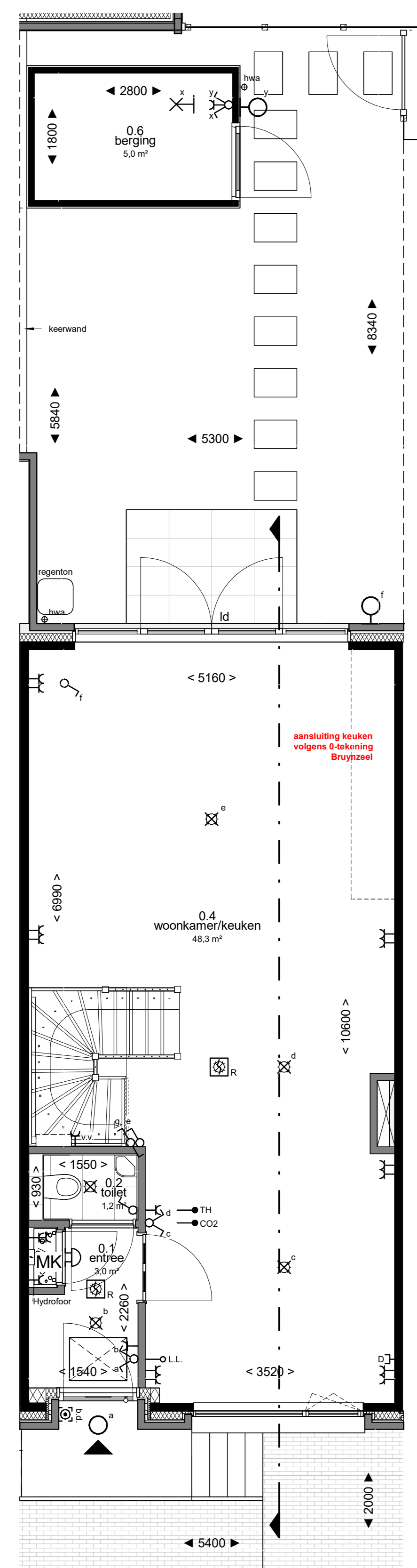
begane grond 1 : 50
