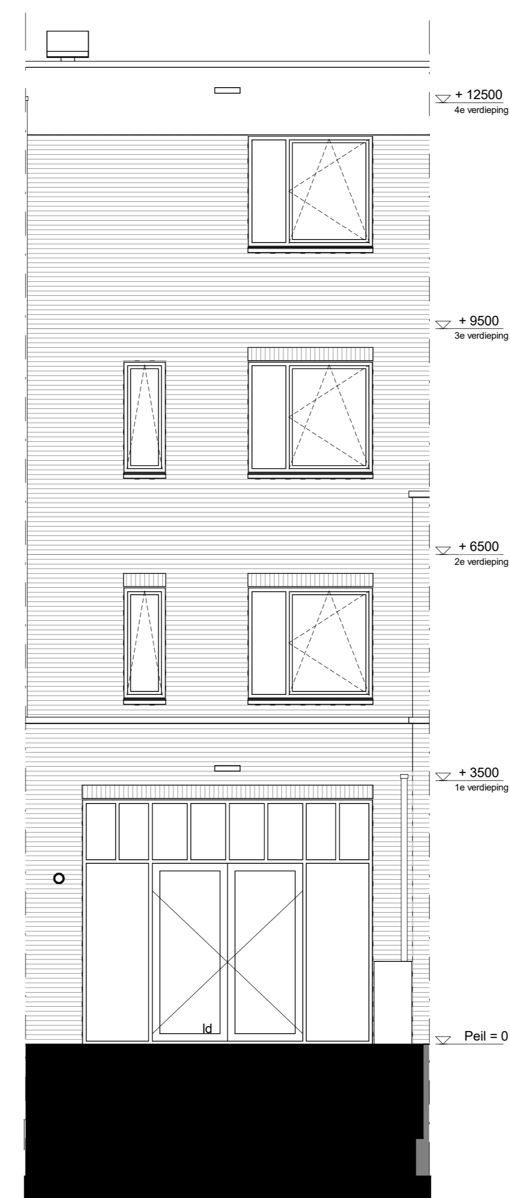
achtergevel 1 : 50
