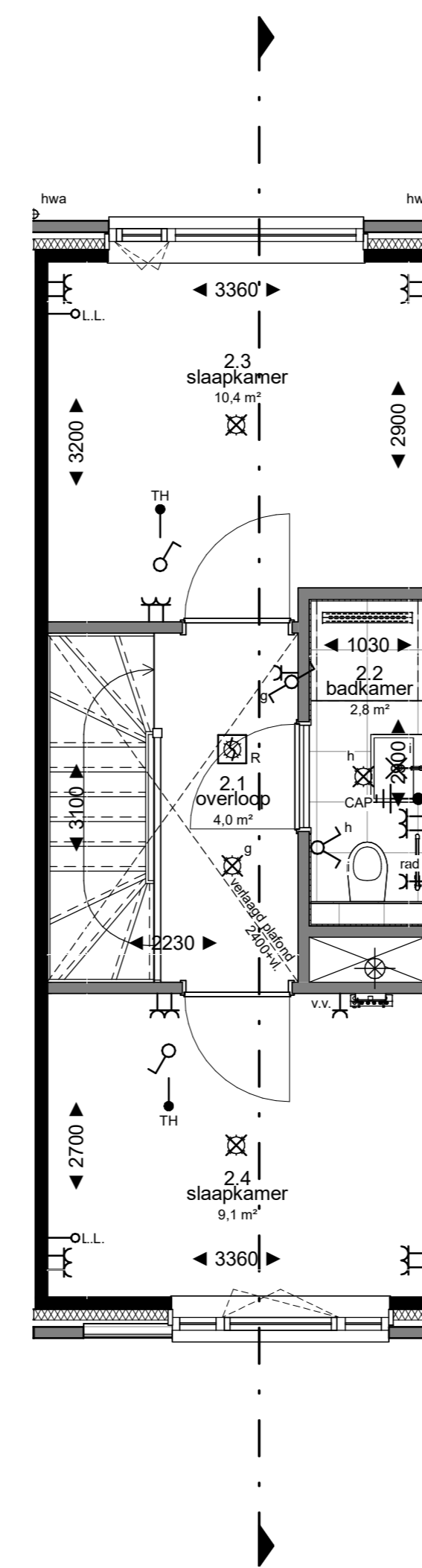
2e verdieping 1 : 50
