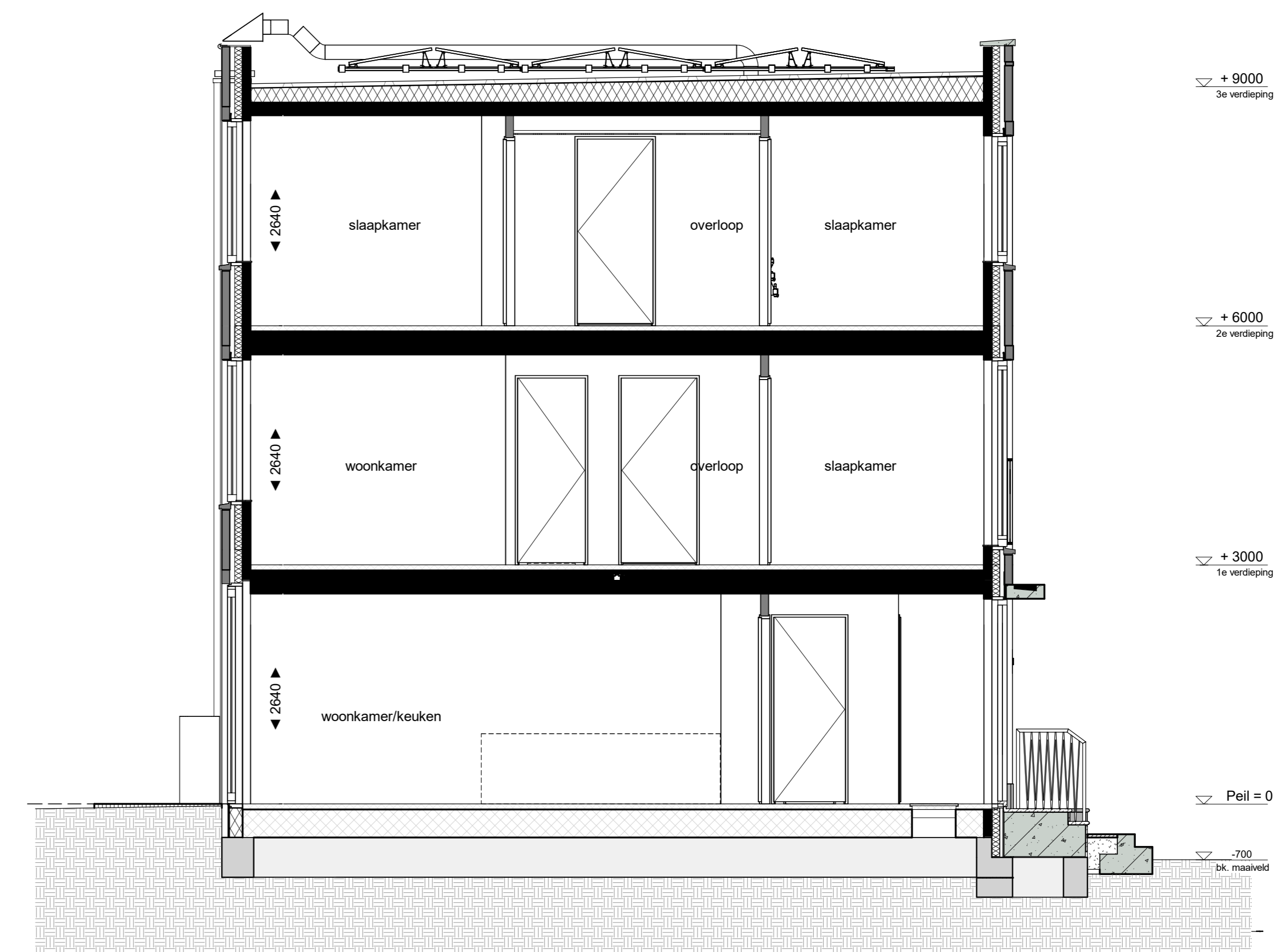
doorsnede A 1 : 50
