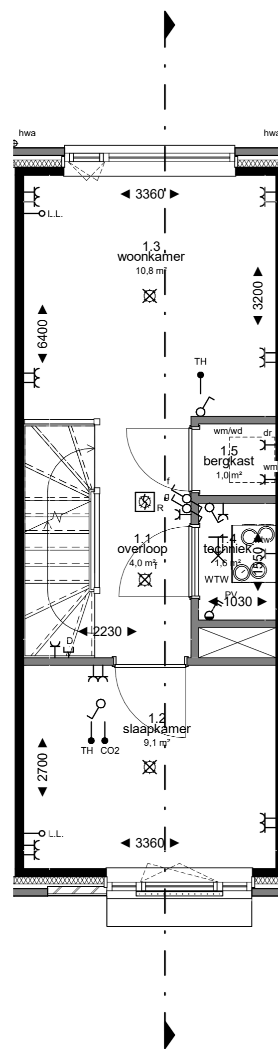
1e verdieping 1 : 50
