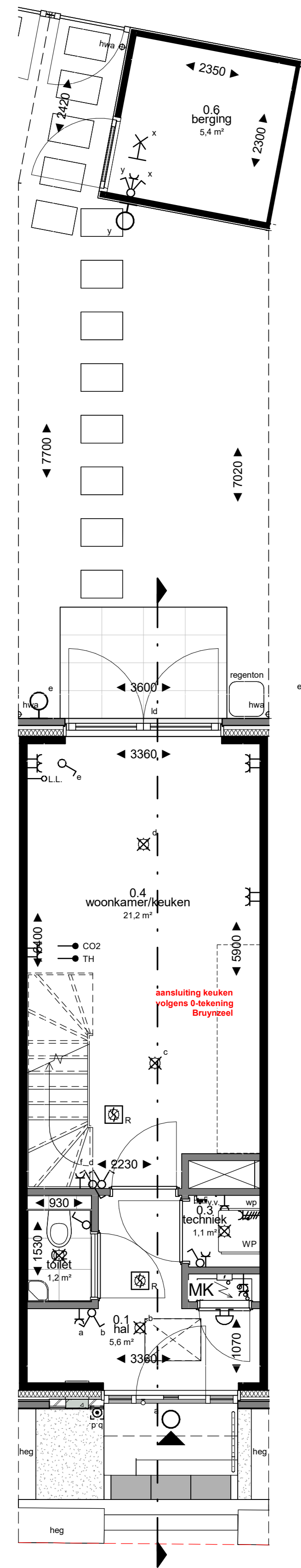
begane grond 1 : 50
