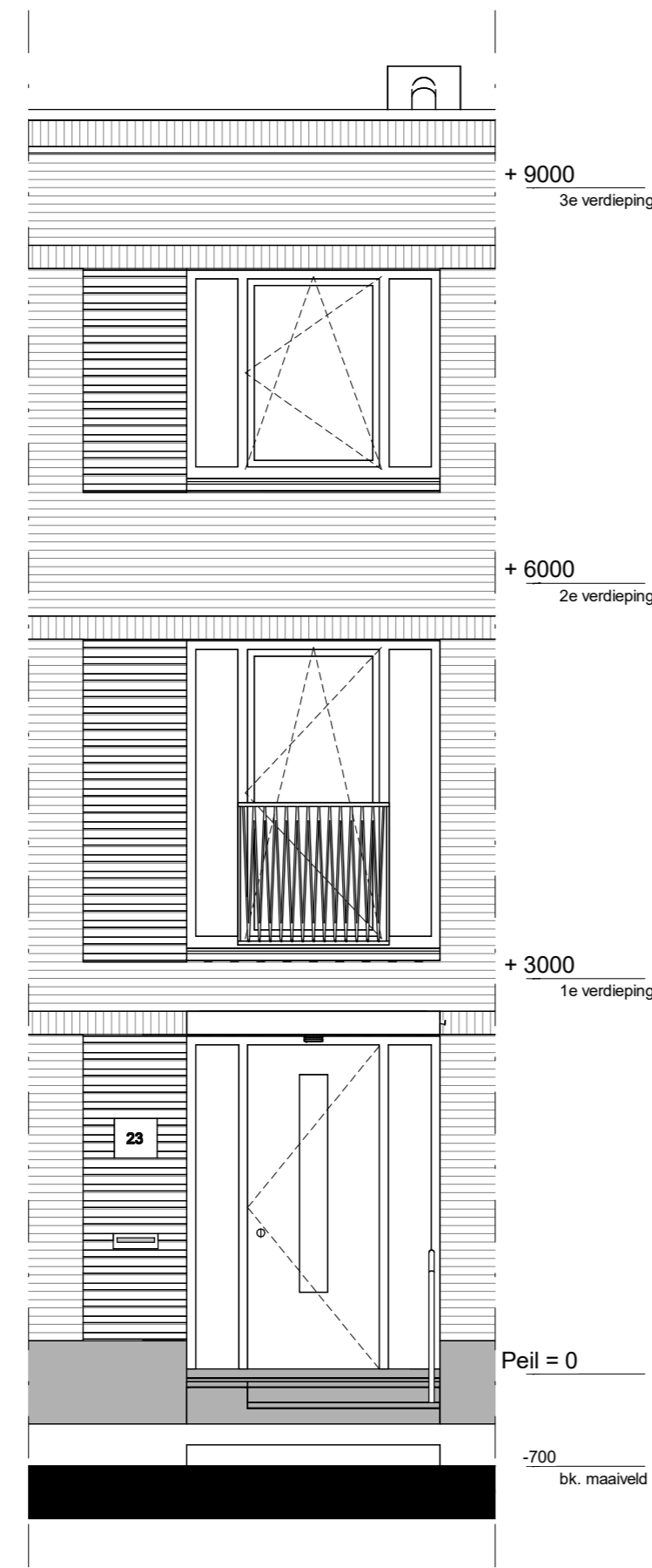
voorgevel 1 : 50
