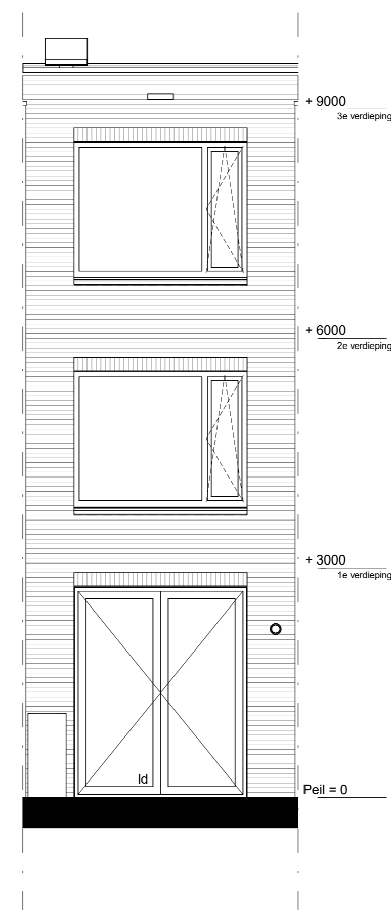
achtergevel 1 : 50
