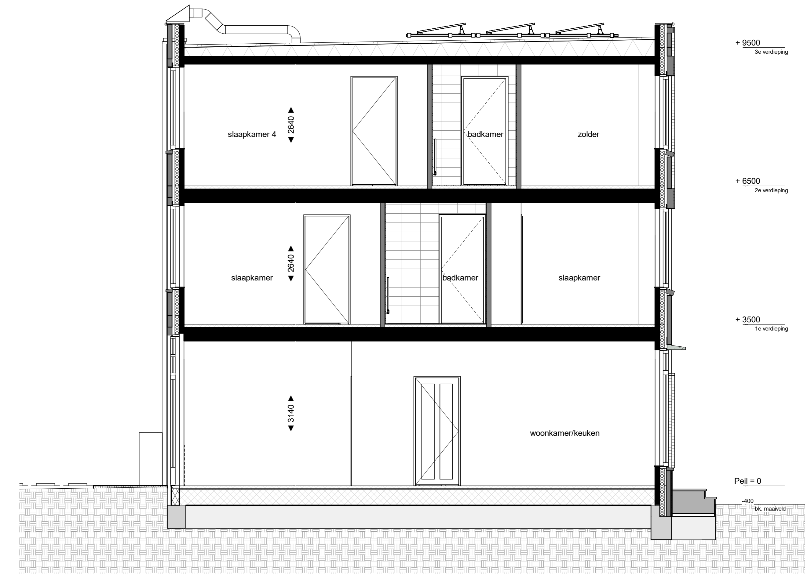
doorsnede A 1 : 50
