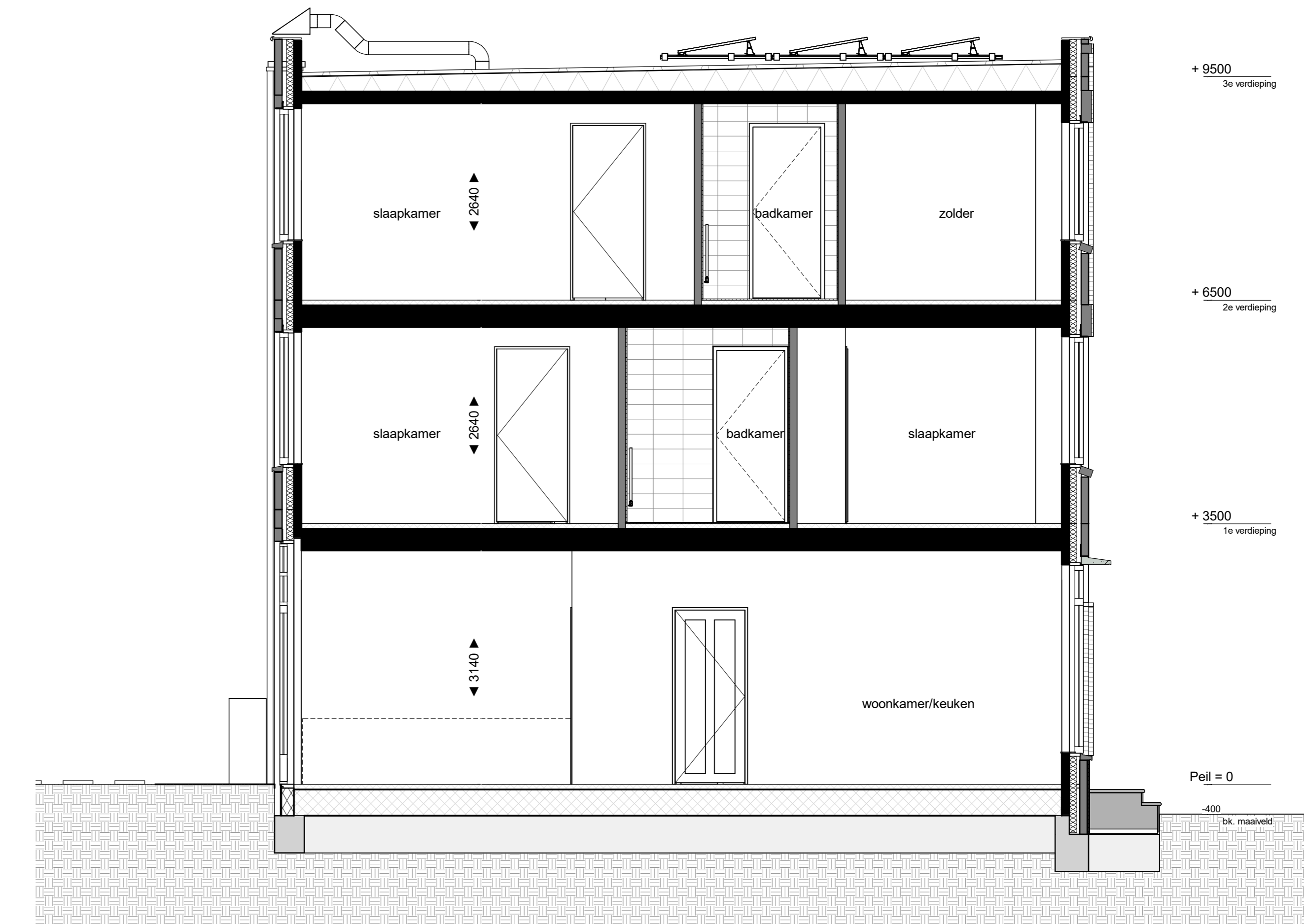
doorsnede A 1 : 50
