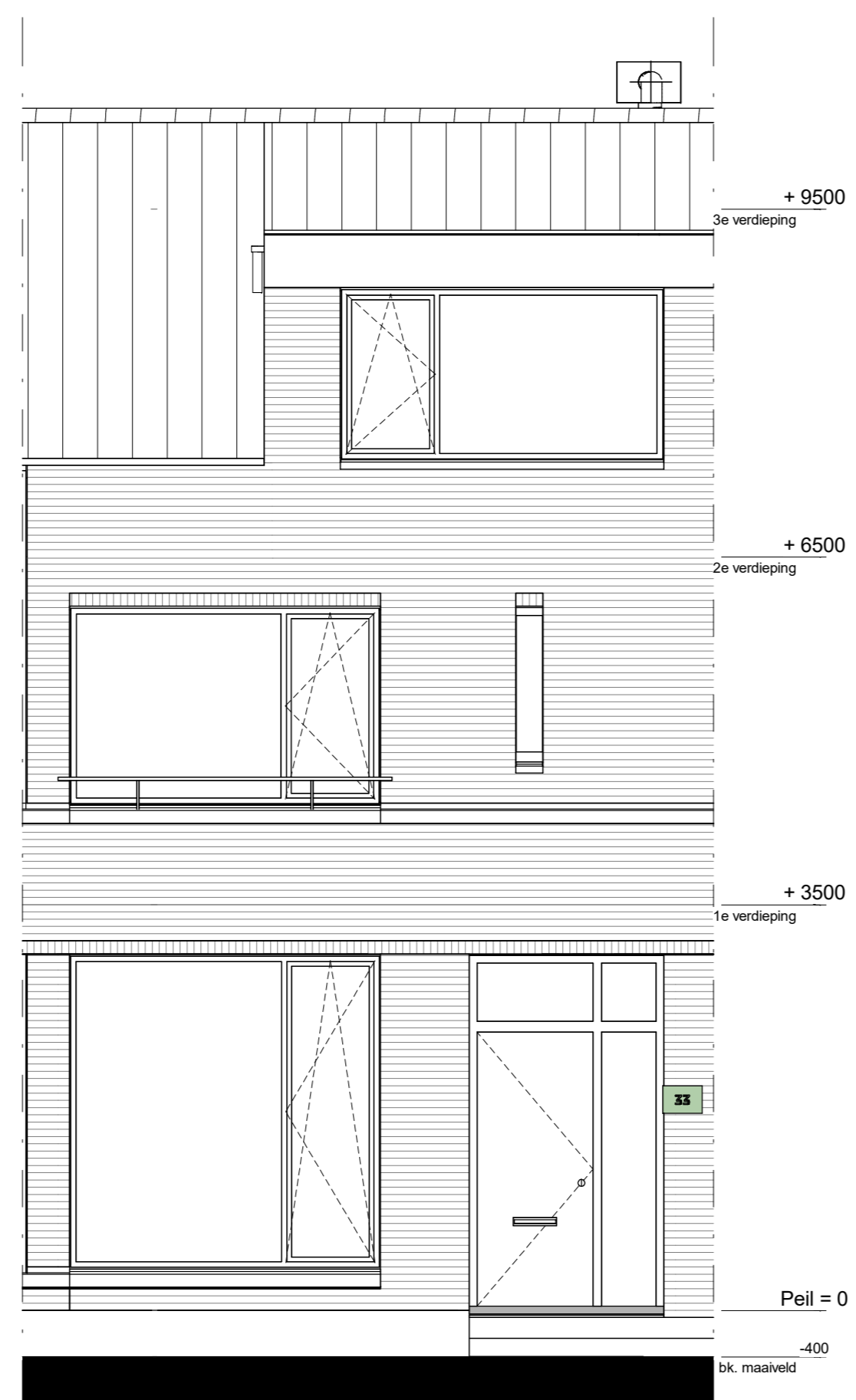
voorgevel 1 : 50
