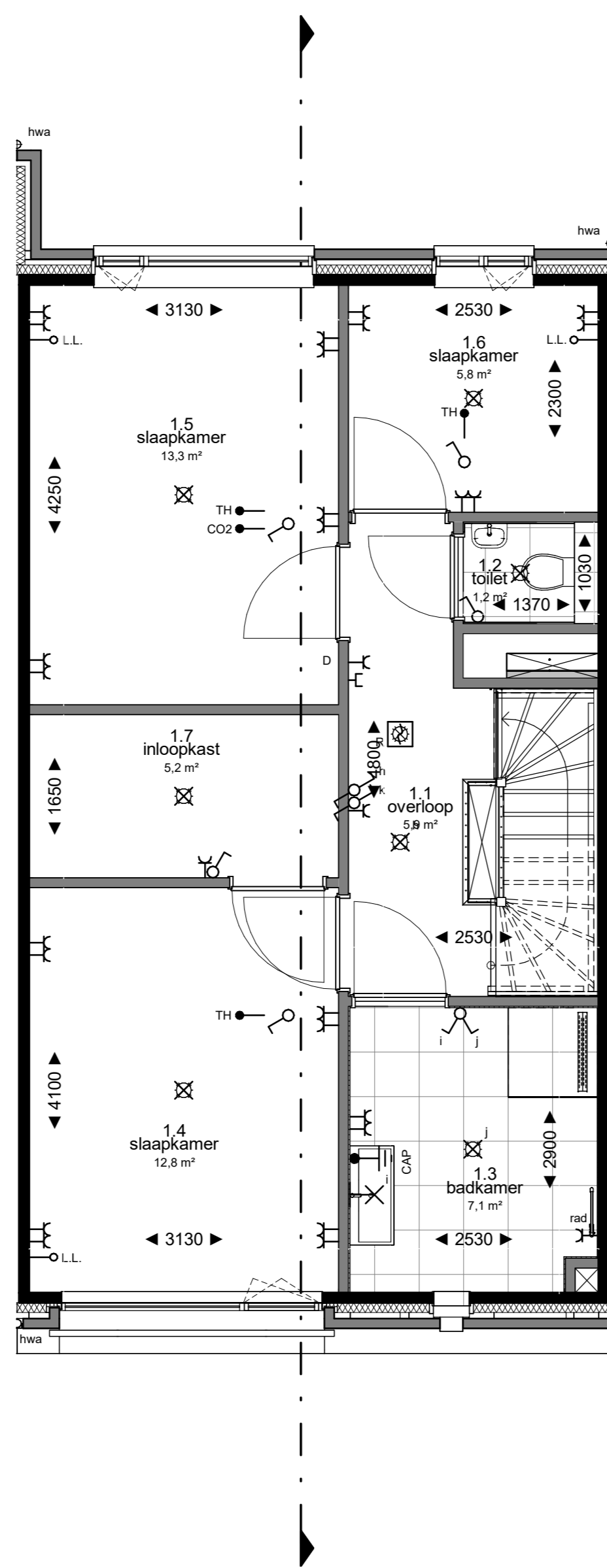
1e verdieping 1 : 50
