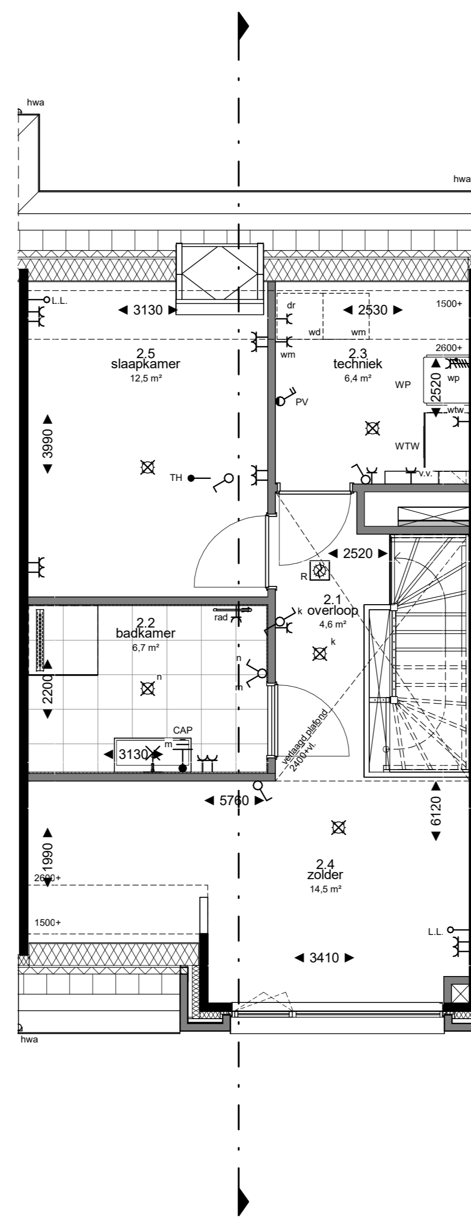
2e verdieping 1 : 50
