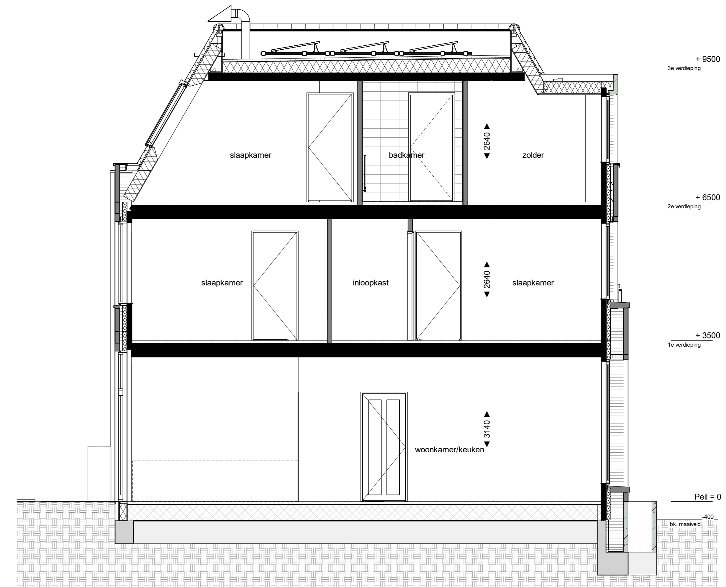
doorsnede A 1 : 50
