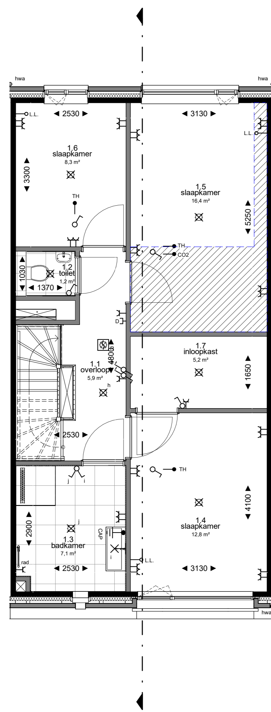
1e verdieping 1 : 50
