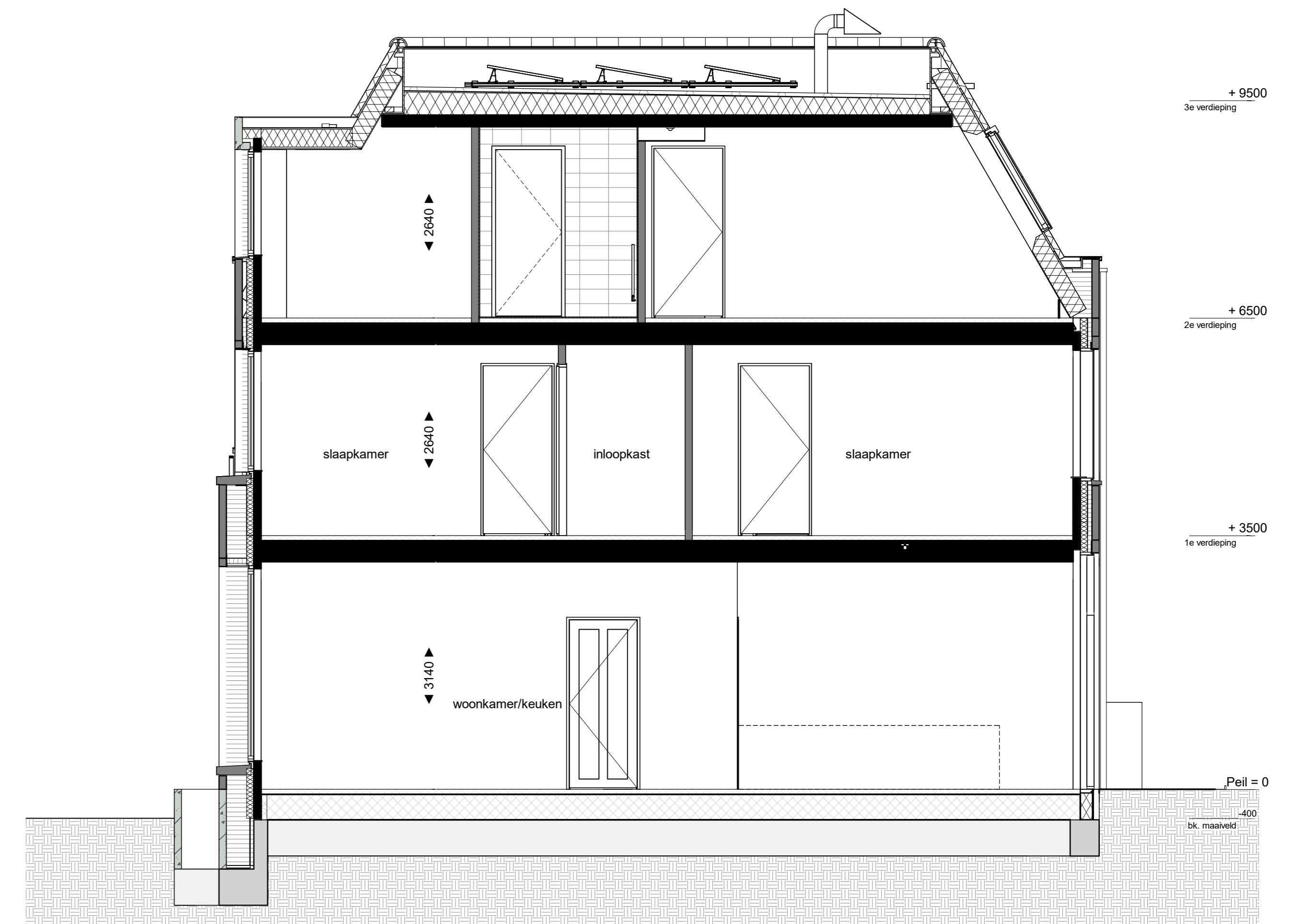
doorsnede A 1 : 50
