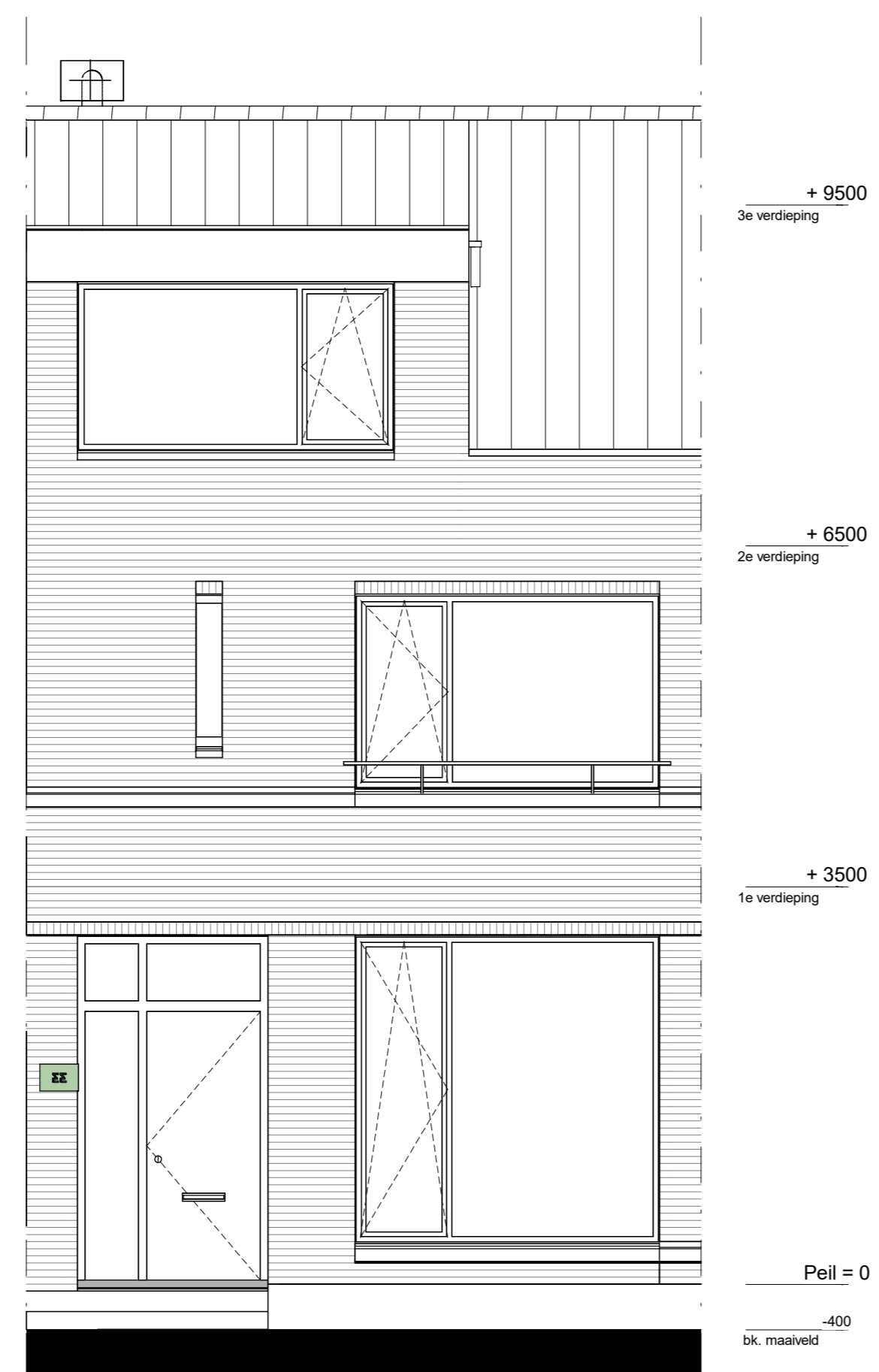
voorgevel 1 : 50
