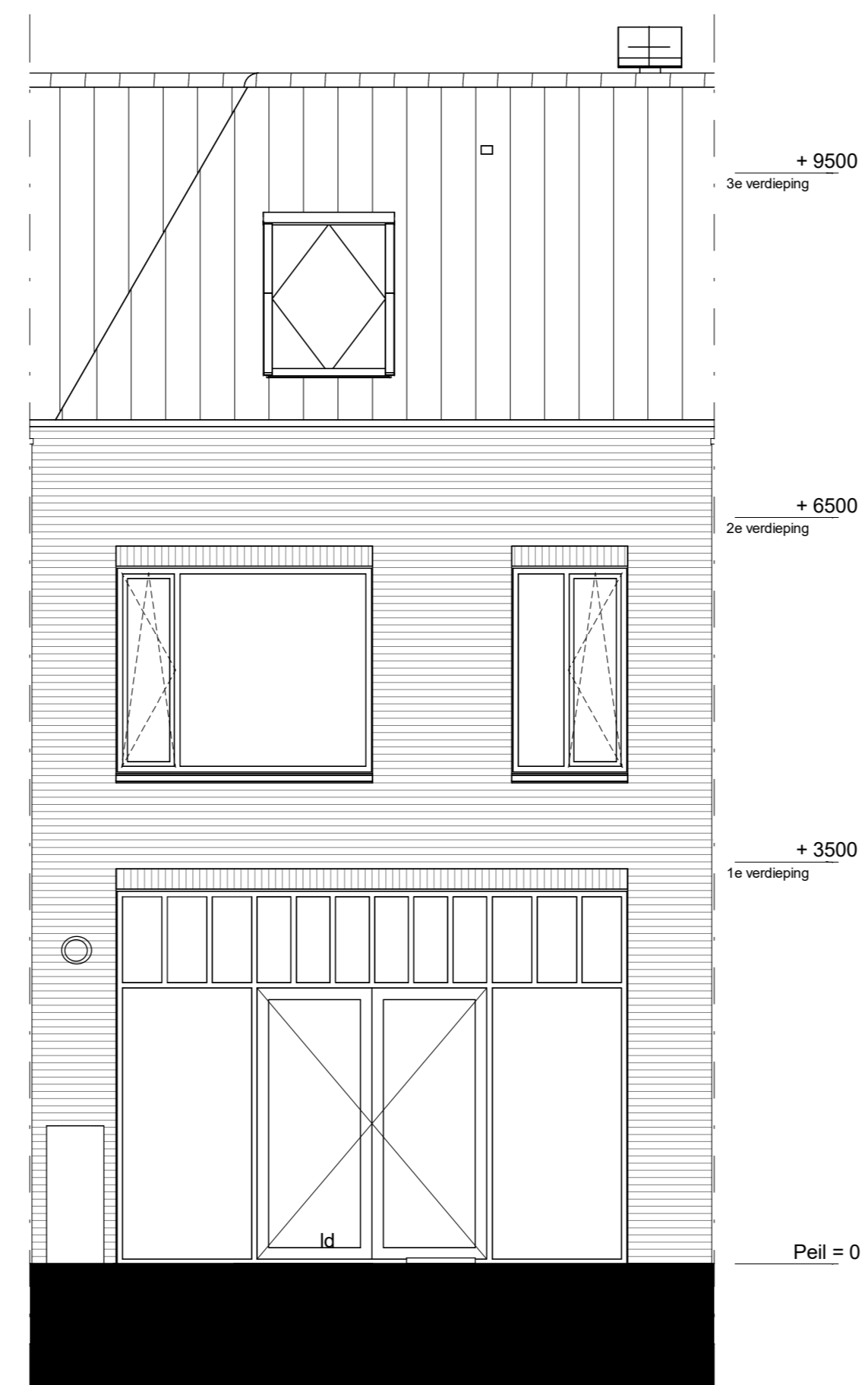
achtergevel 1 : 50
