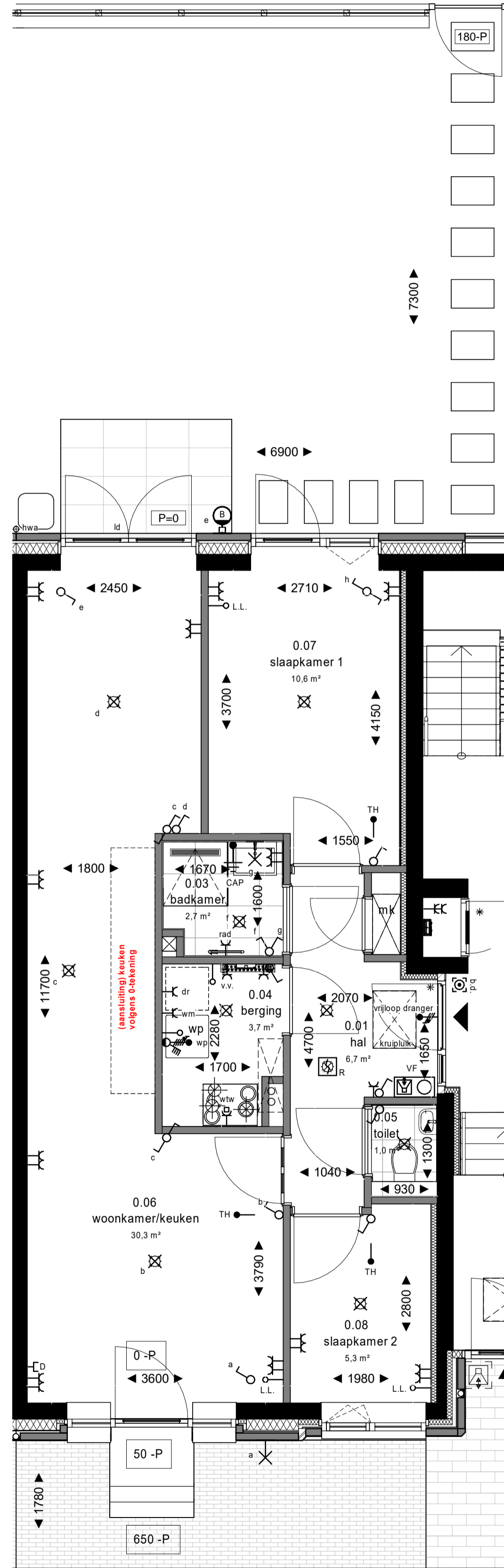
Begane grond 1 : 50
