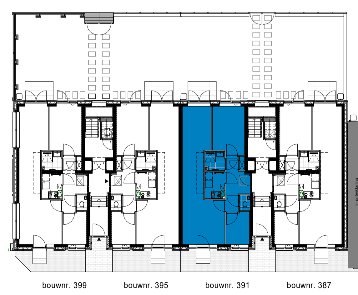
begane grond D1 Appartementen 1 : 200
