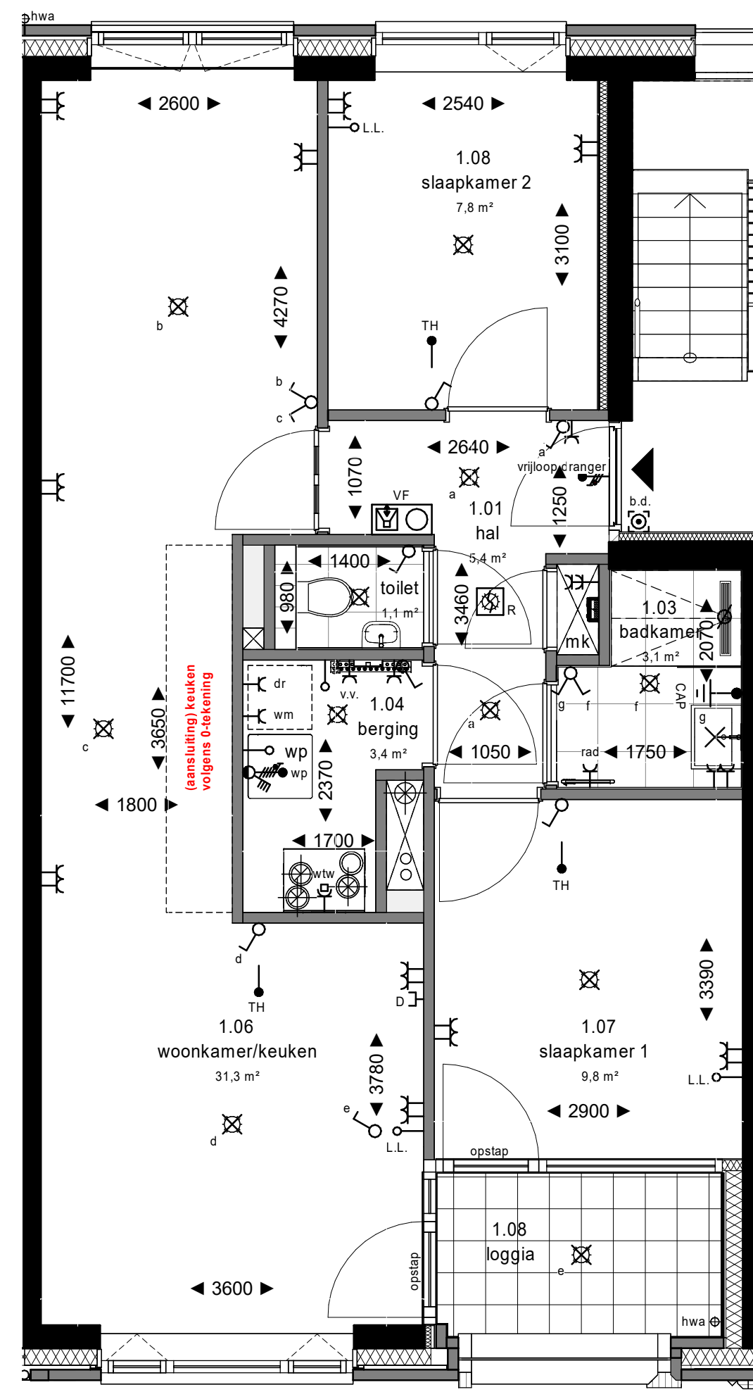
1e verdieping 1 : 50
