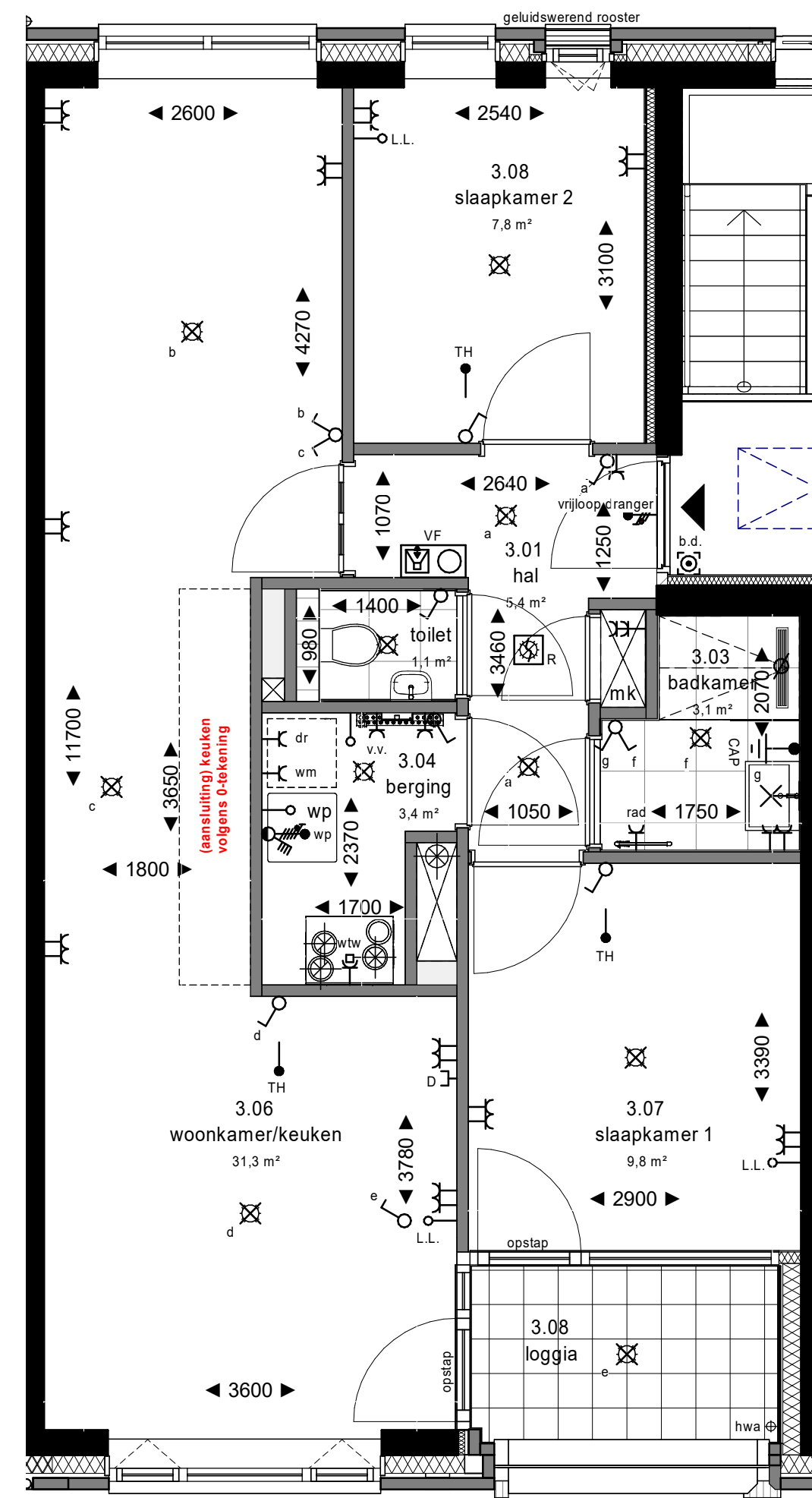
3e verdieping 1 : 50
