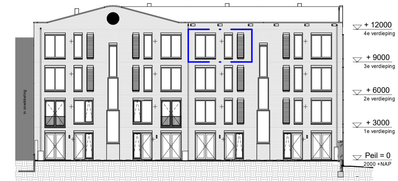
Achtergevel 1 : 200
