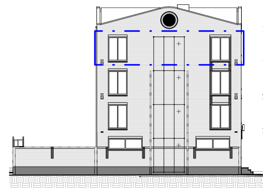
Zijgevel 1 : 200
