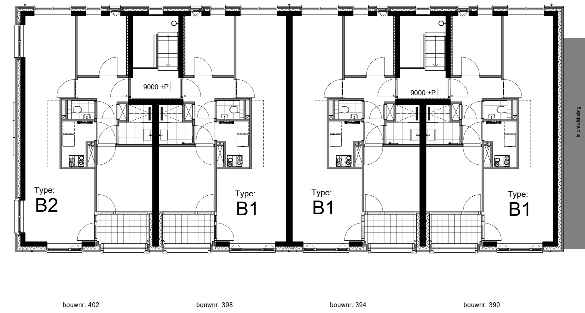
3e verdieping D1 Appartementen 1 : 100
