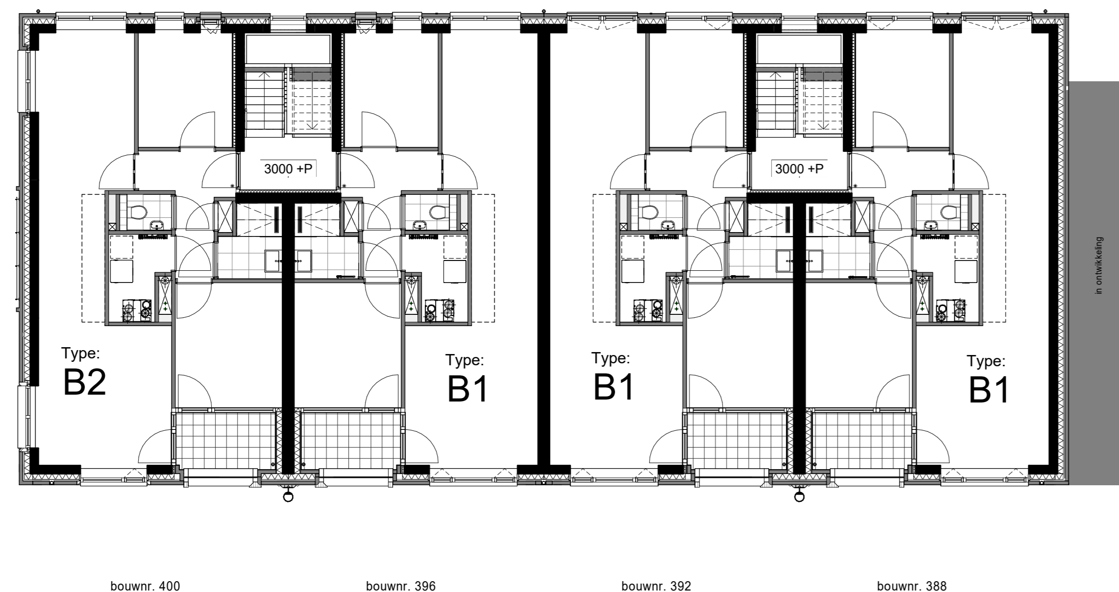
1e verdieping D1 Appartementen 1 : 100
