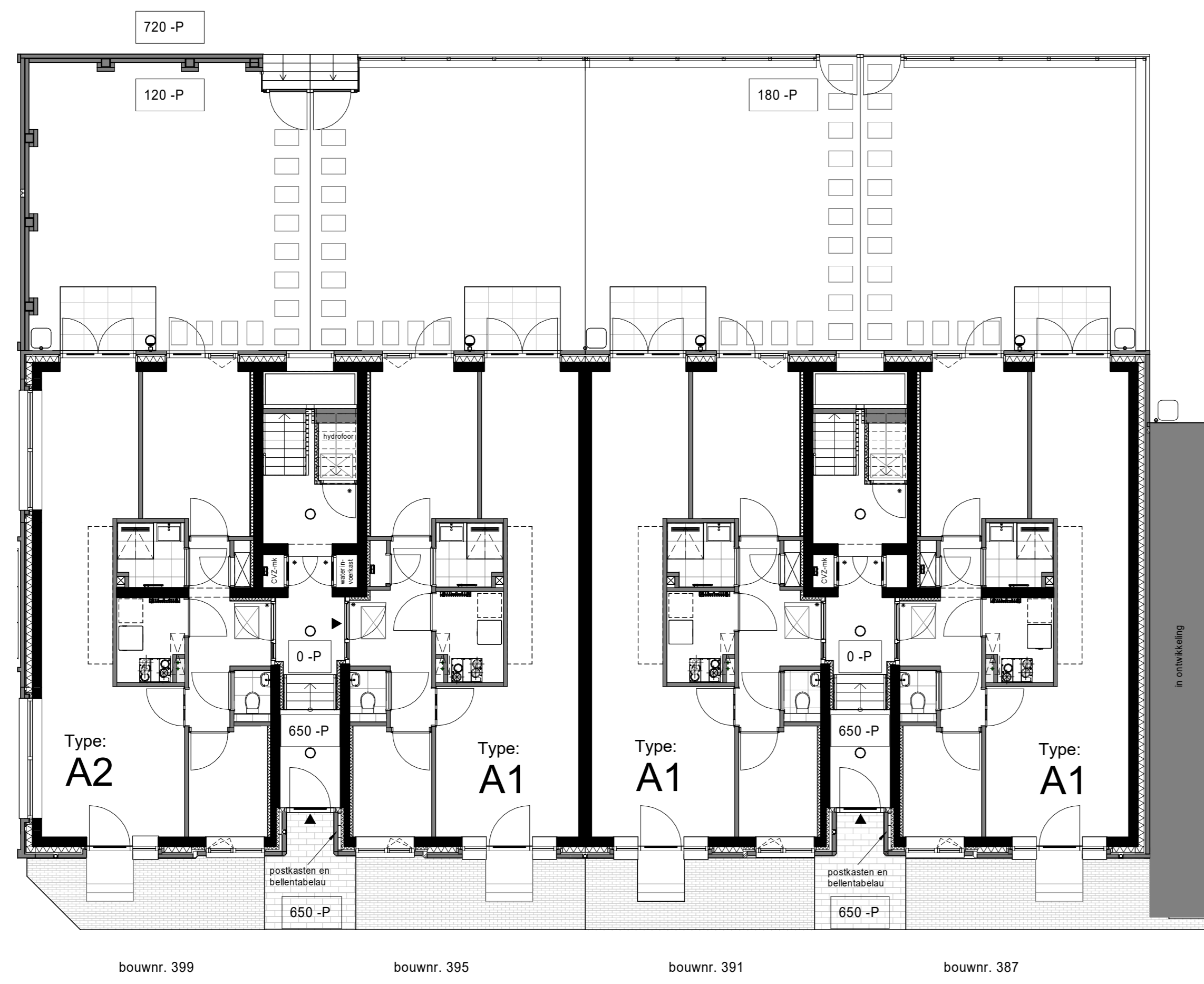
begane grond D1 Appartementen 1 : 100
