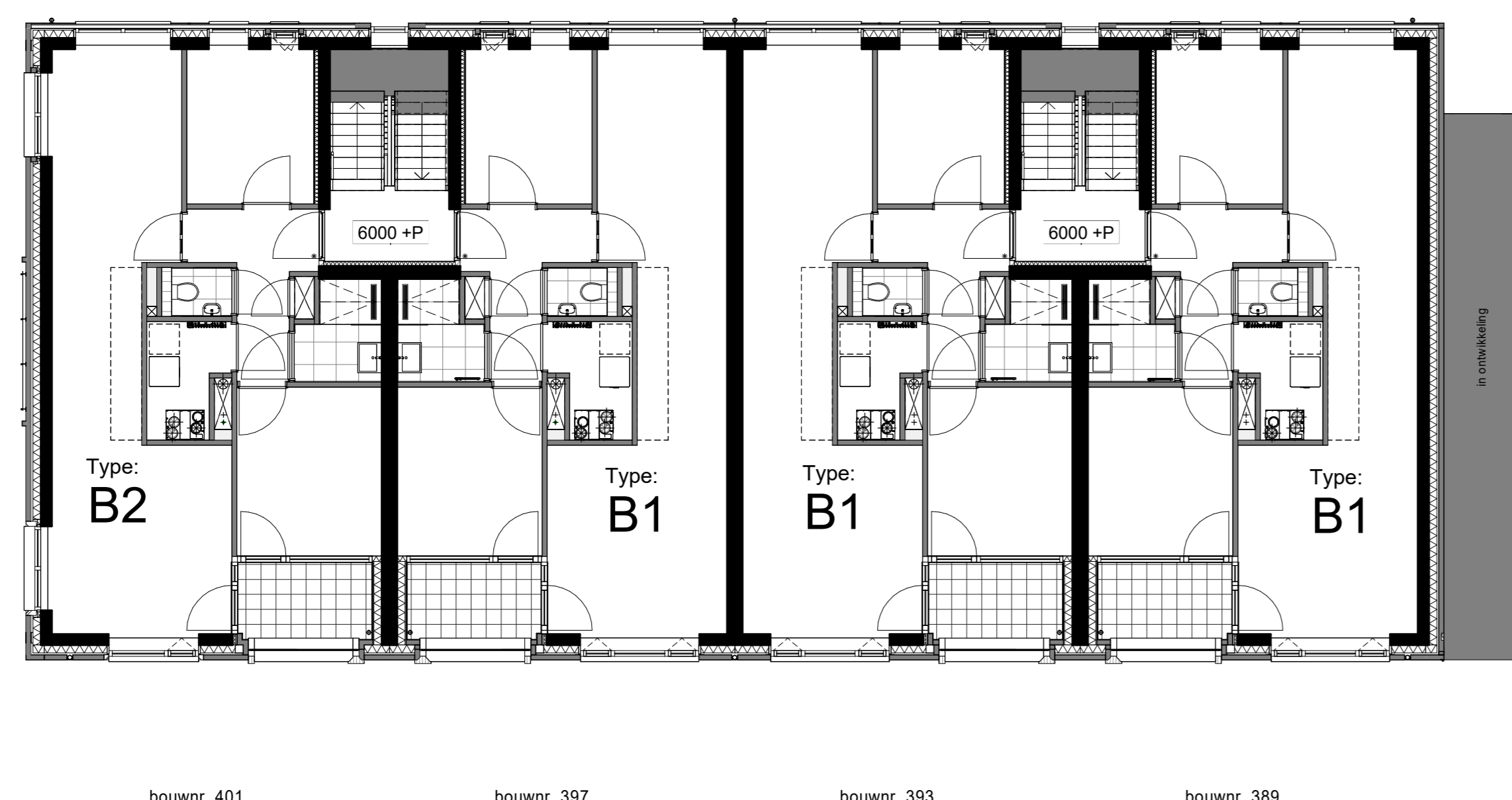
2e verdieping D1 Appartementen 1 : 100
