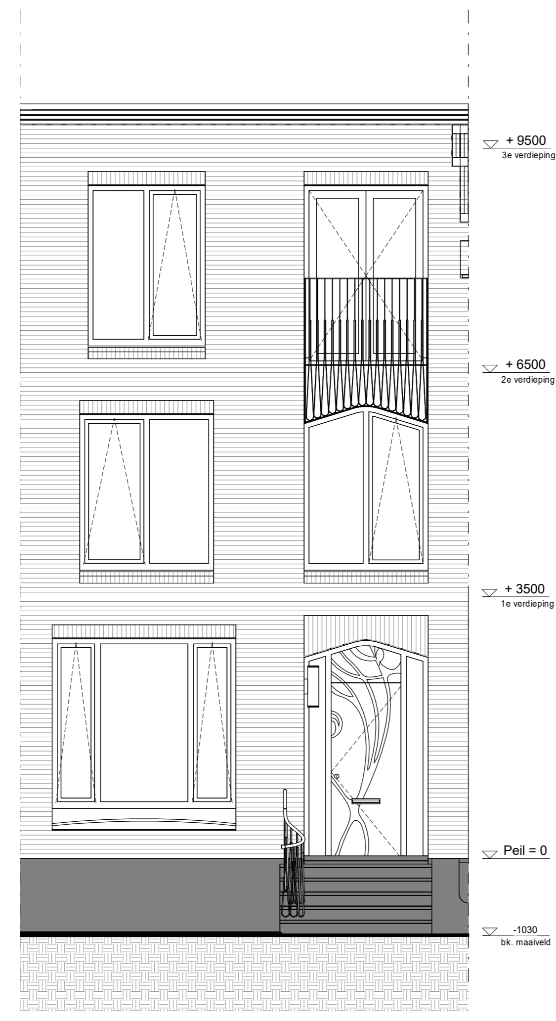
Voorgevel 1 : 50
