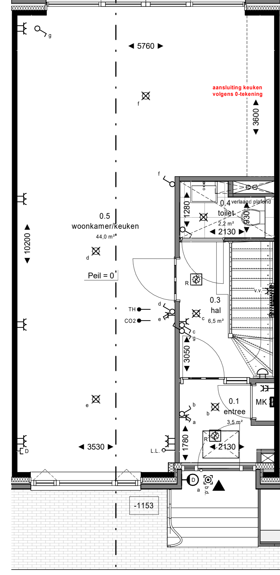
Begane grond 1 : 50
