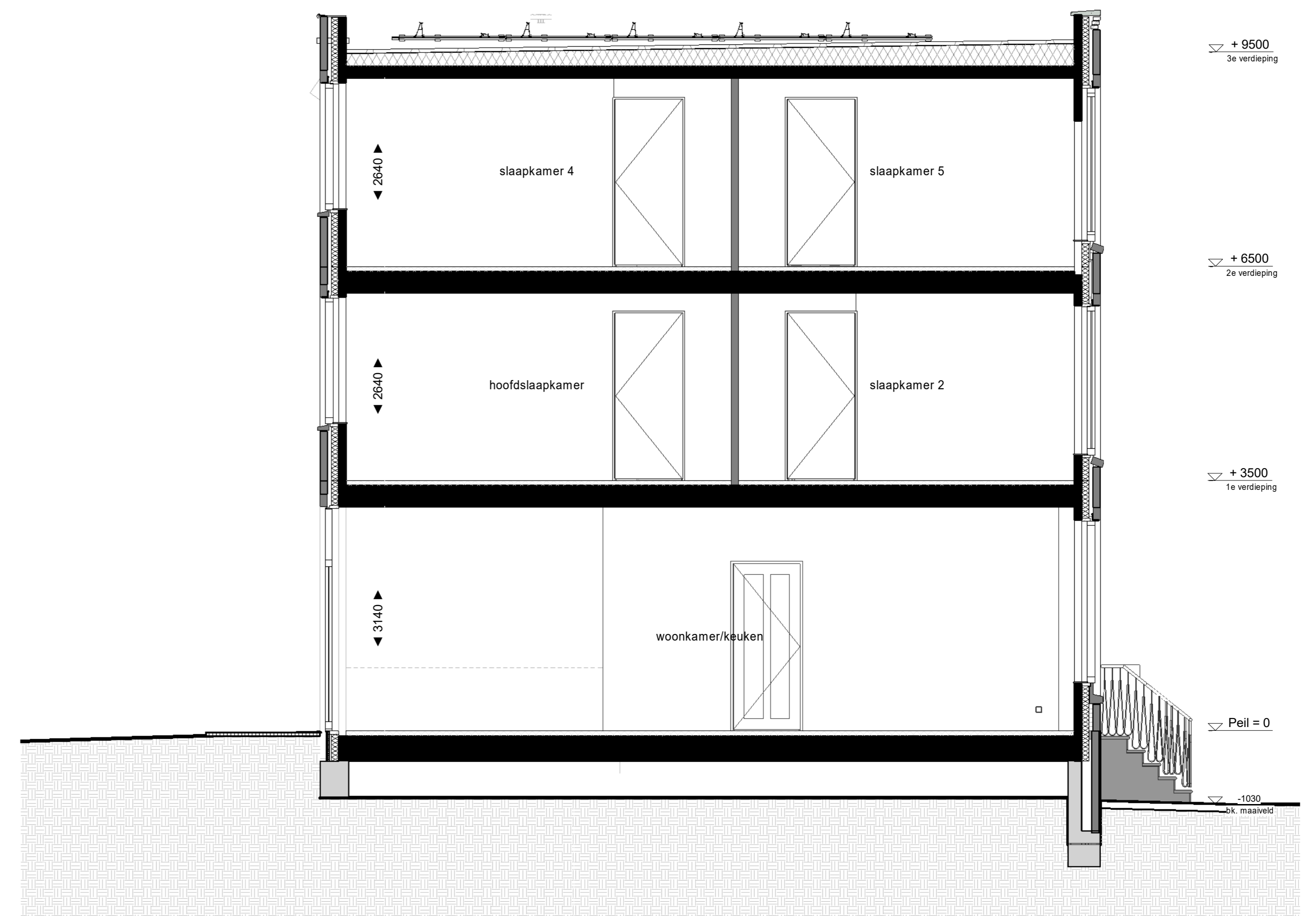
Doorsnede 1 : 50
