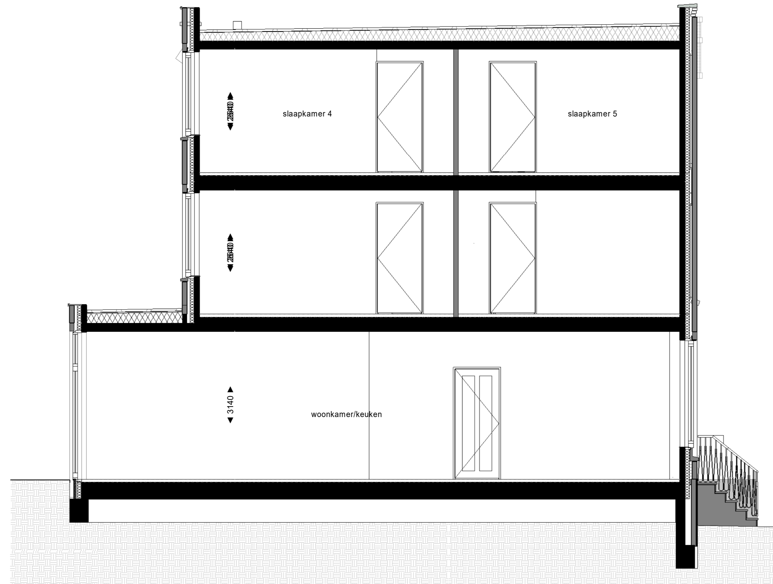
Doorsnede - Optie uitbouw begane grond verdieping (2.4m)
