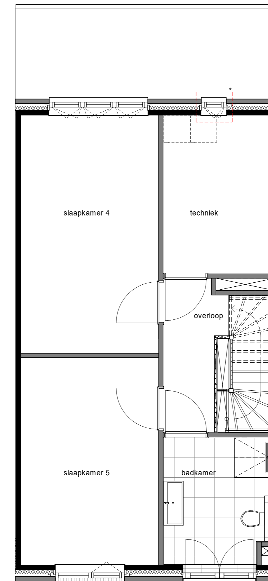
2e Verdieping - Optie raam techniek ruimte * - Optie 3e toilet bnr. 382 en 383
