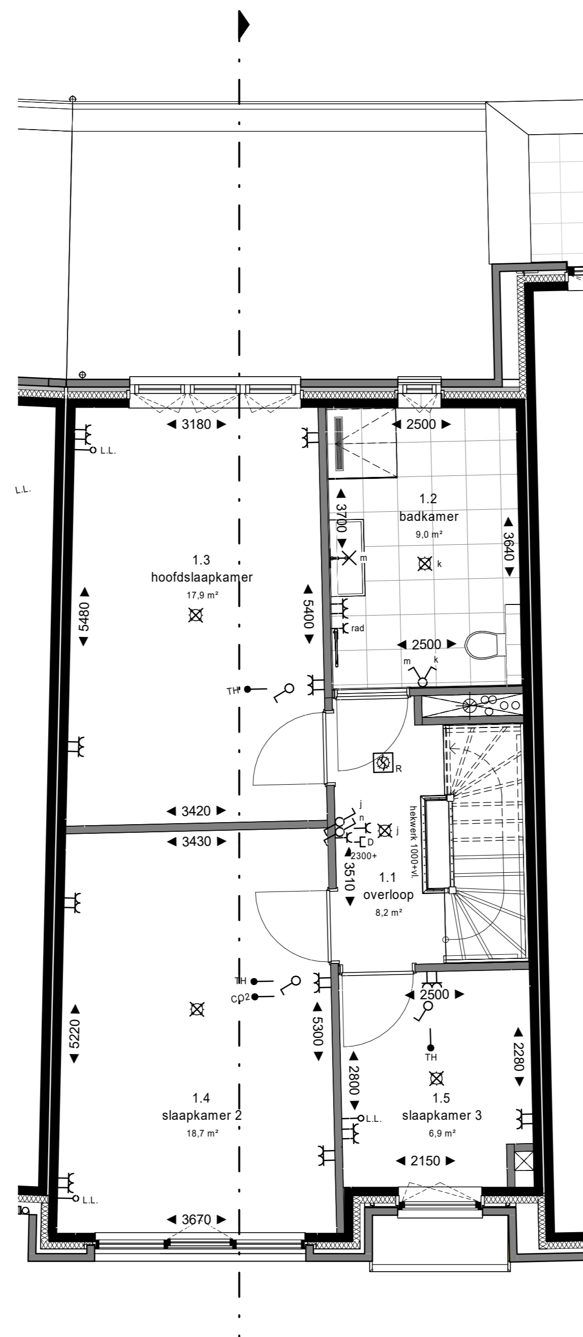
1e verdieping 1 : 50
