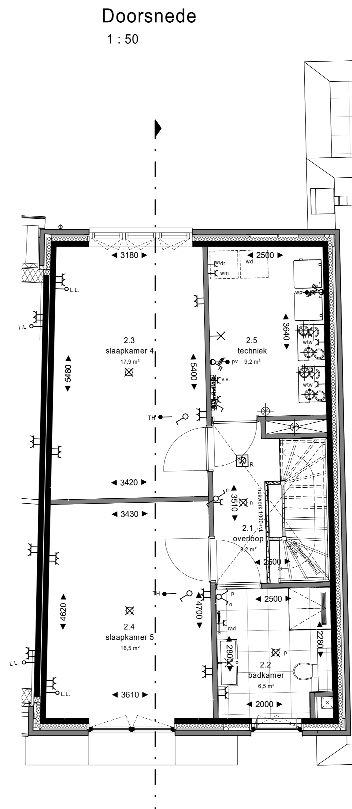
2e verdieping 1 : 50
