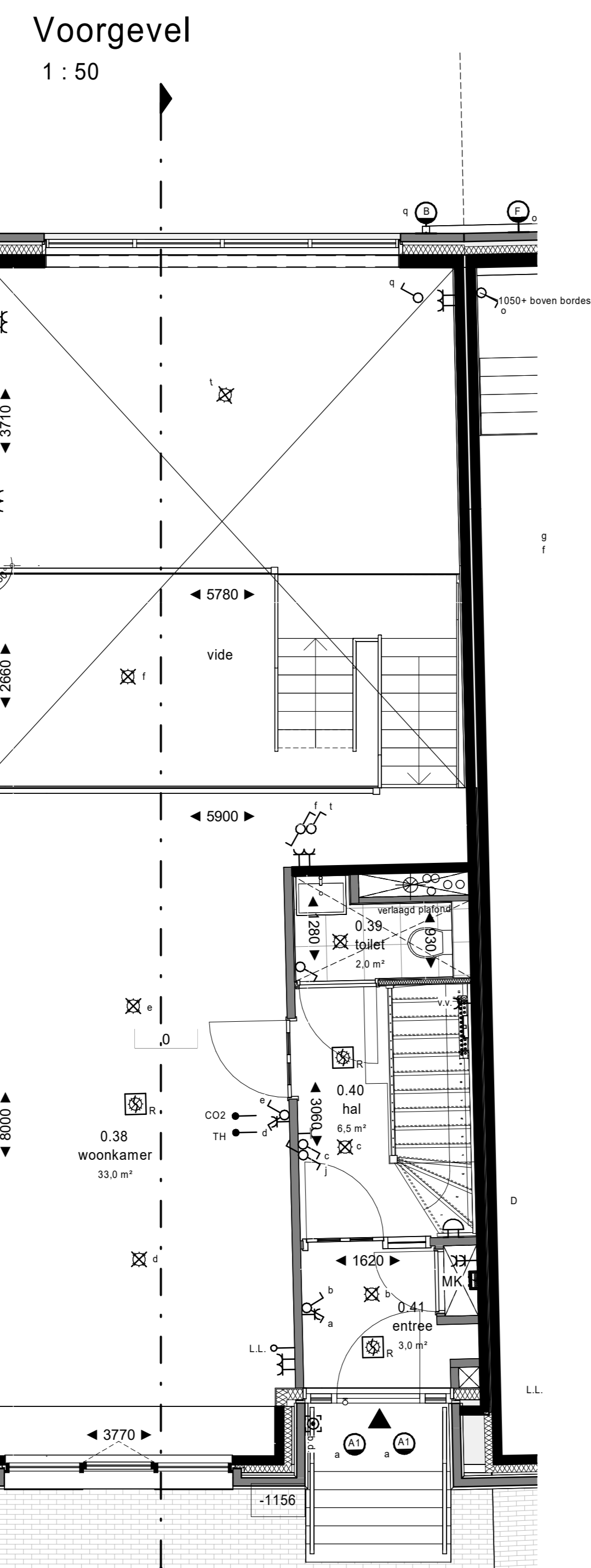
Begane grond 1 : 50
