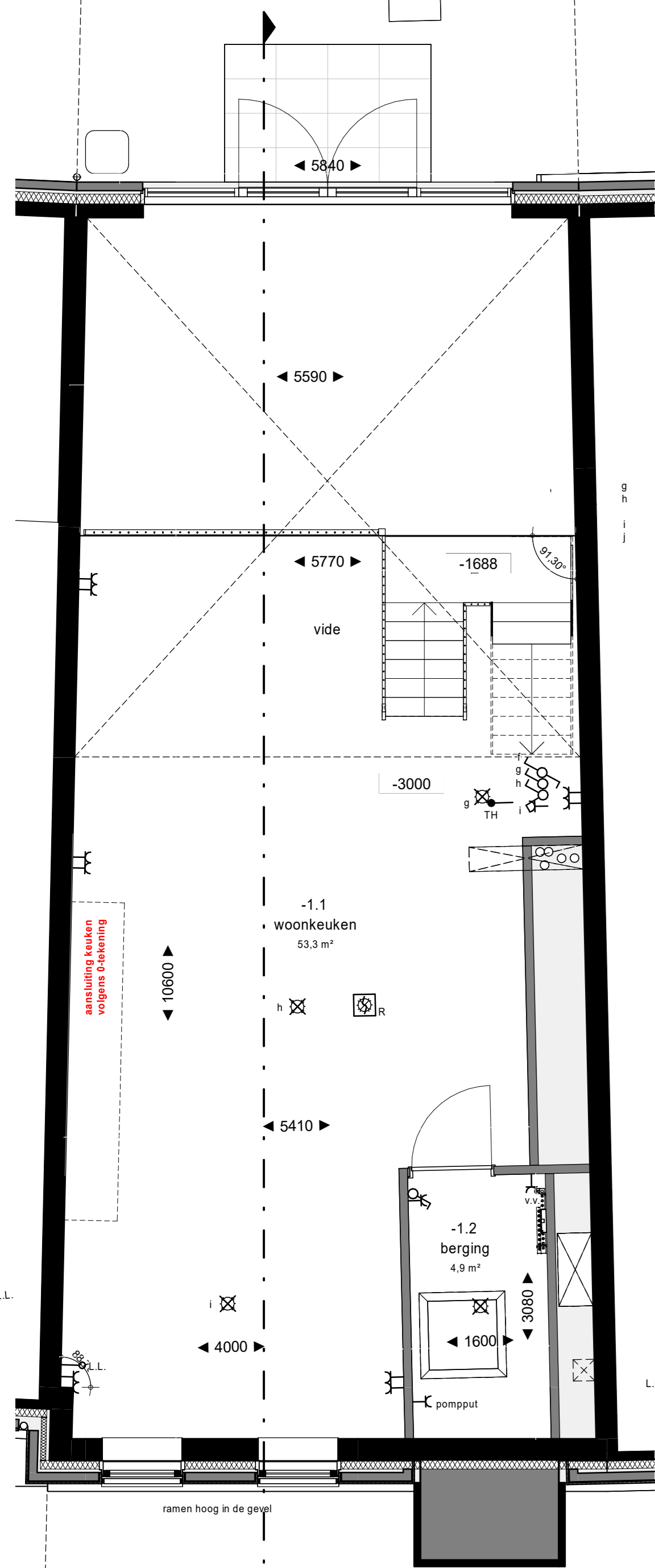
Souterrain 1 : 50
