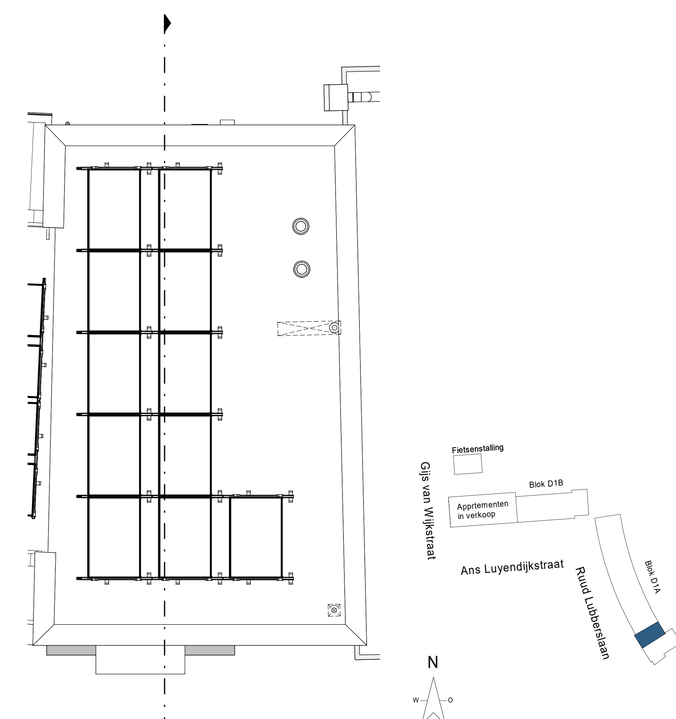
Dakplaattegrond 1 : 50
