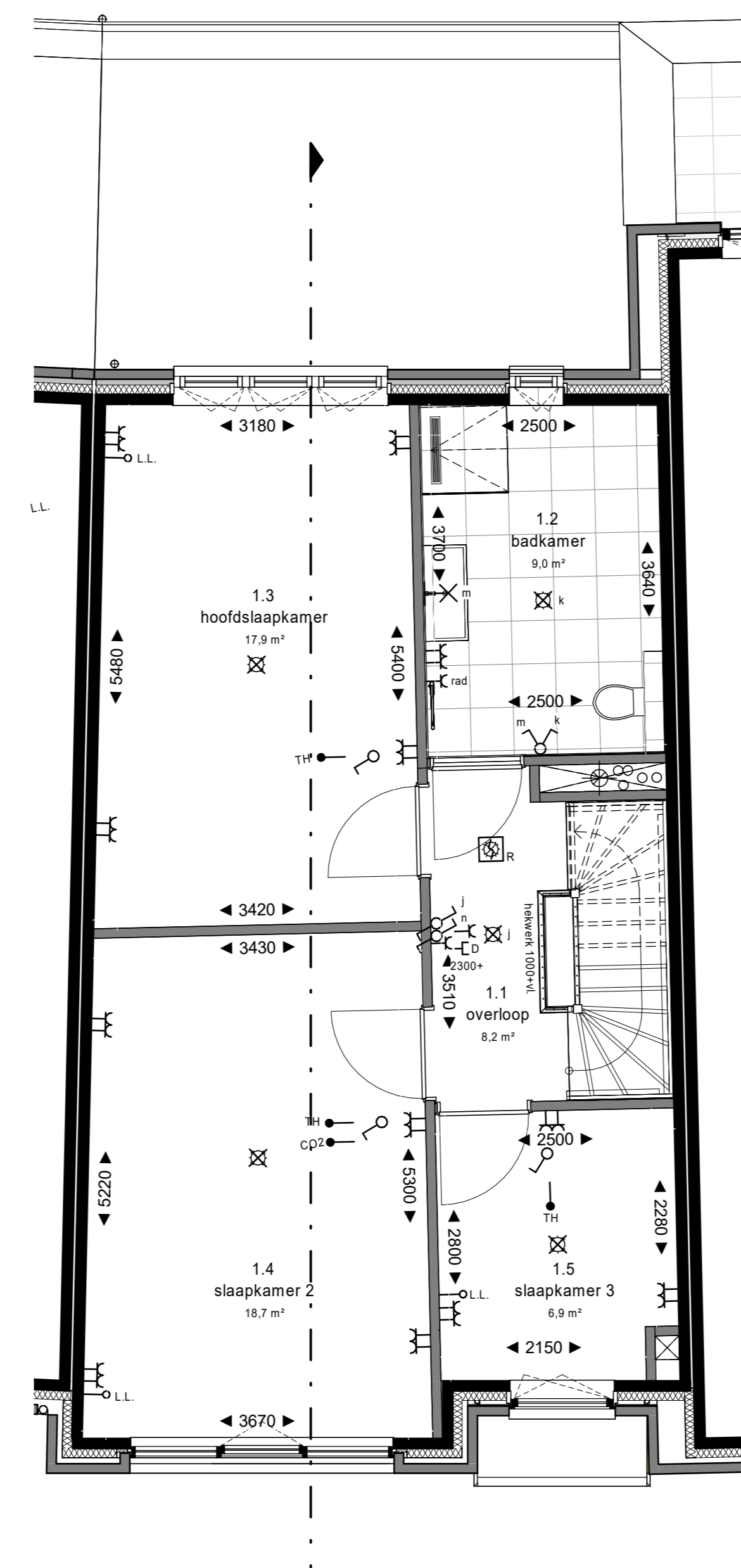
1e verdieping 1 : 50
