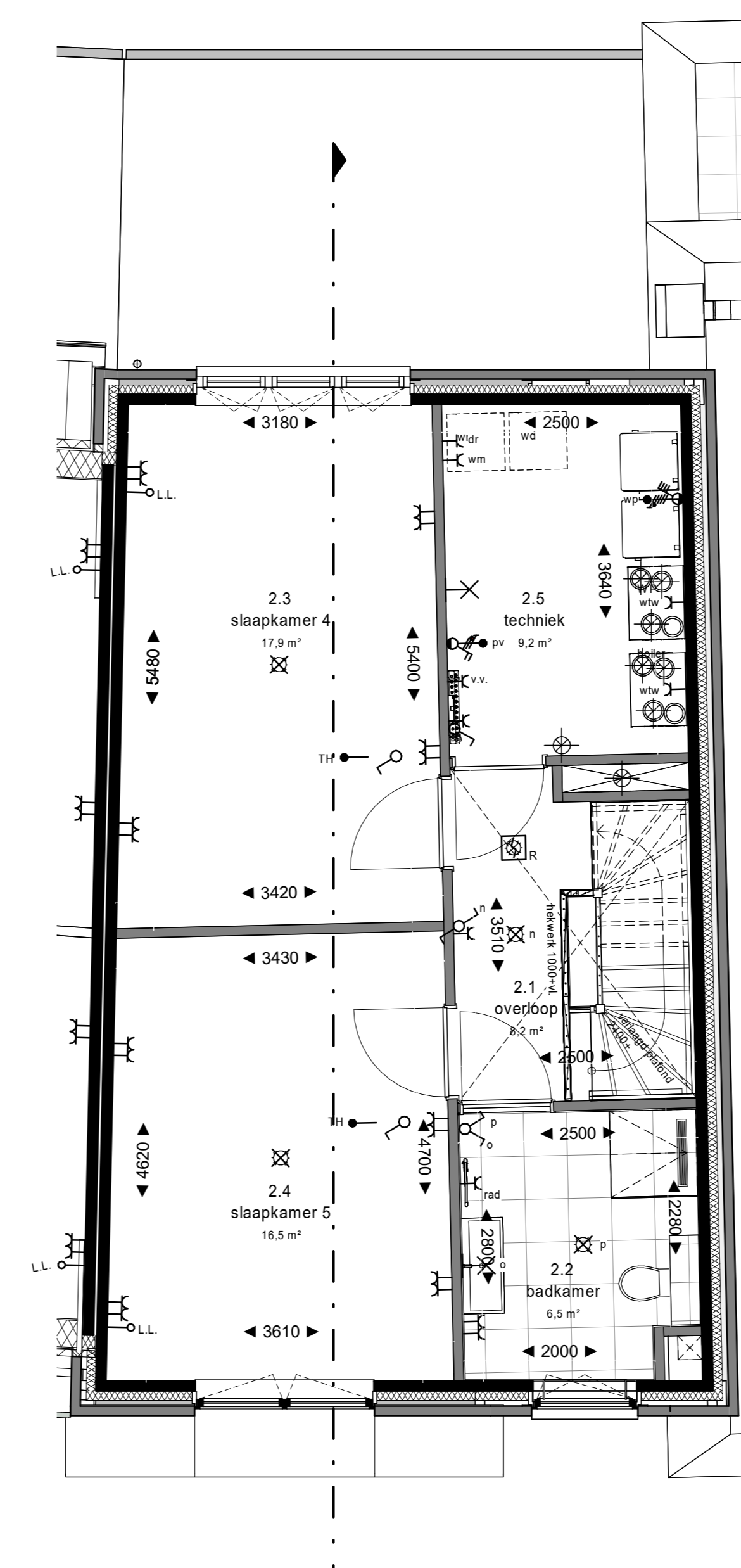
2e verdieping 1 : 50
