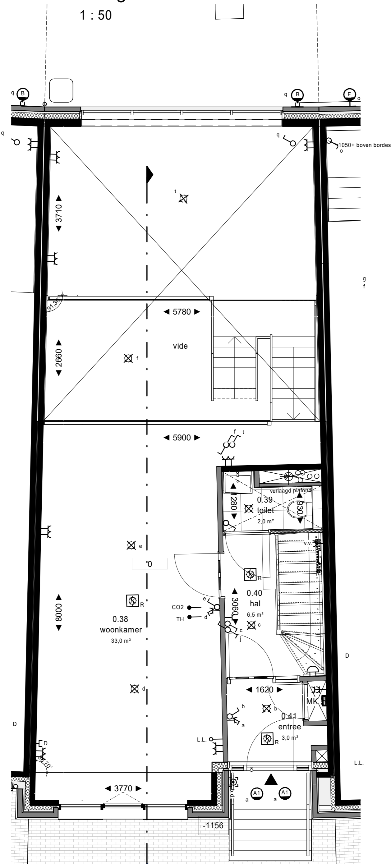
Begane grond 1 : 50
