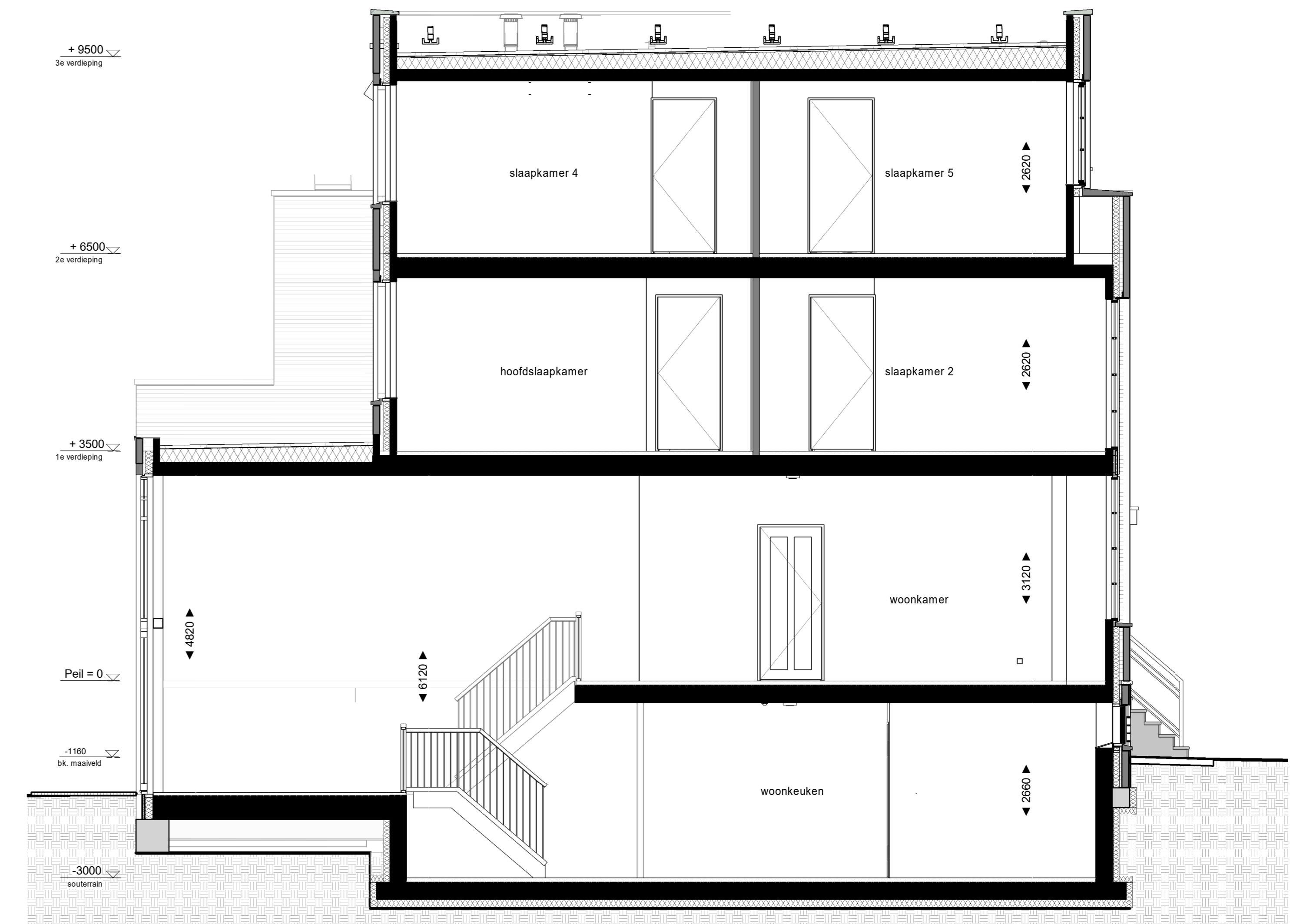
Doorsnede 1 : 50
