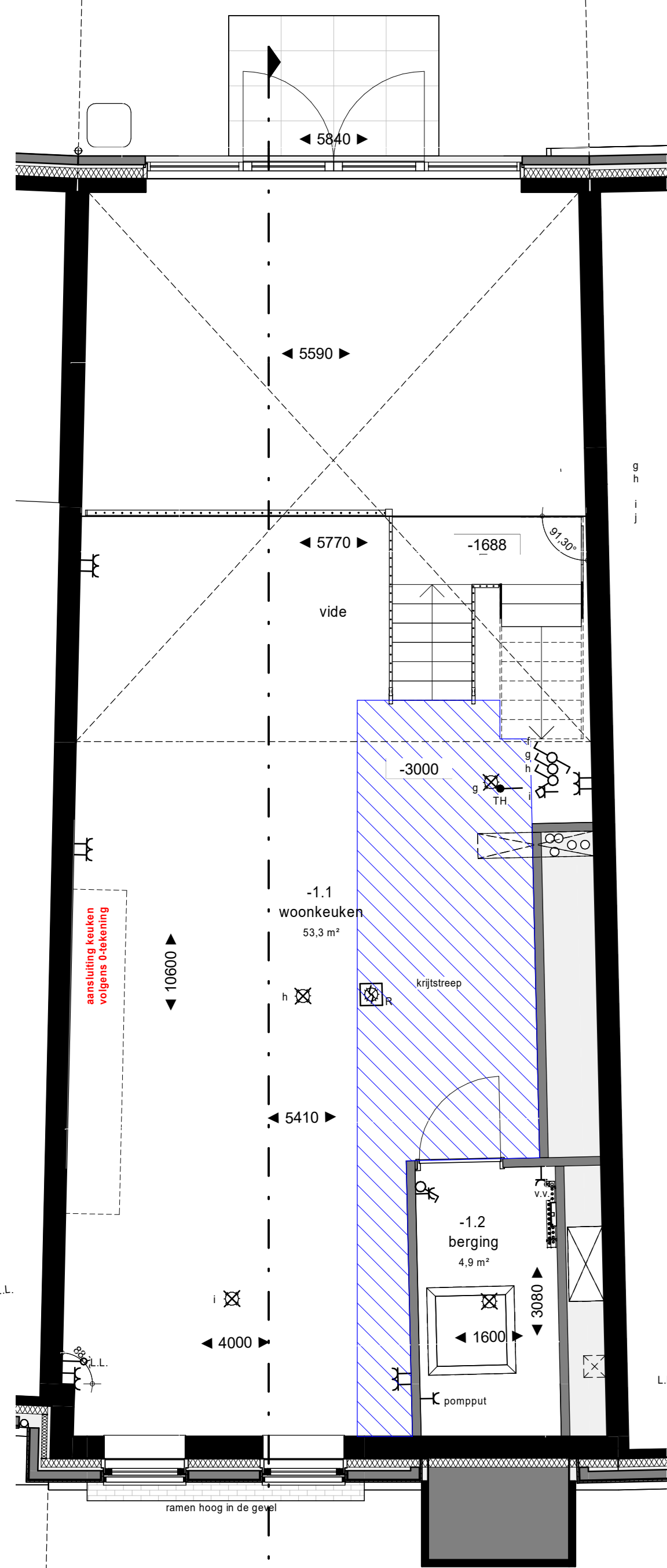
Souterrain 1 : 50
