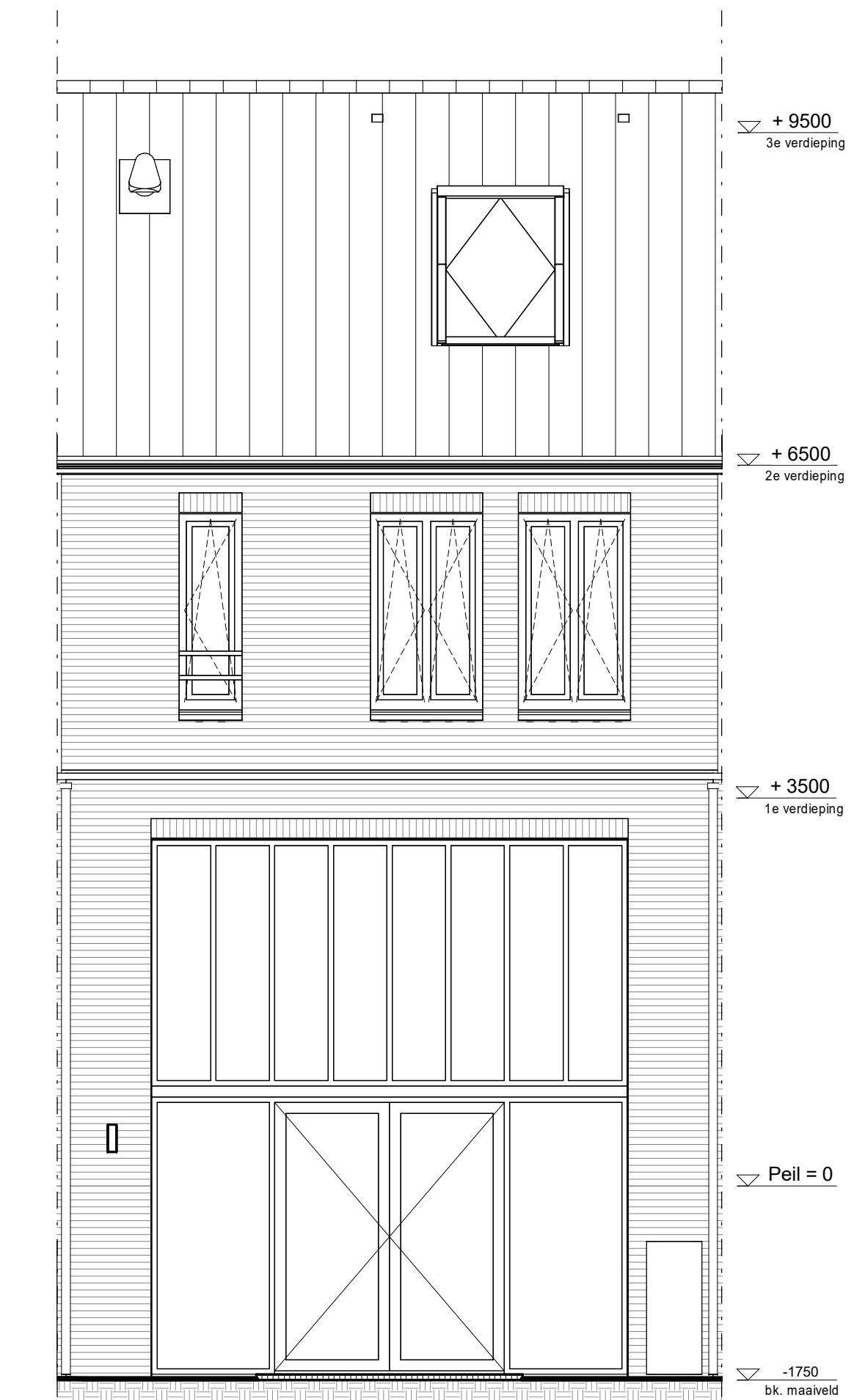
Achtergevel 1 : 50
