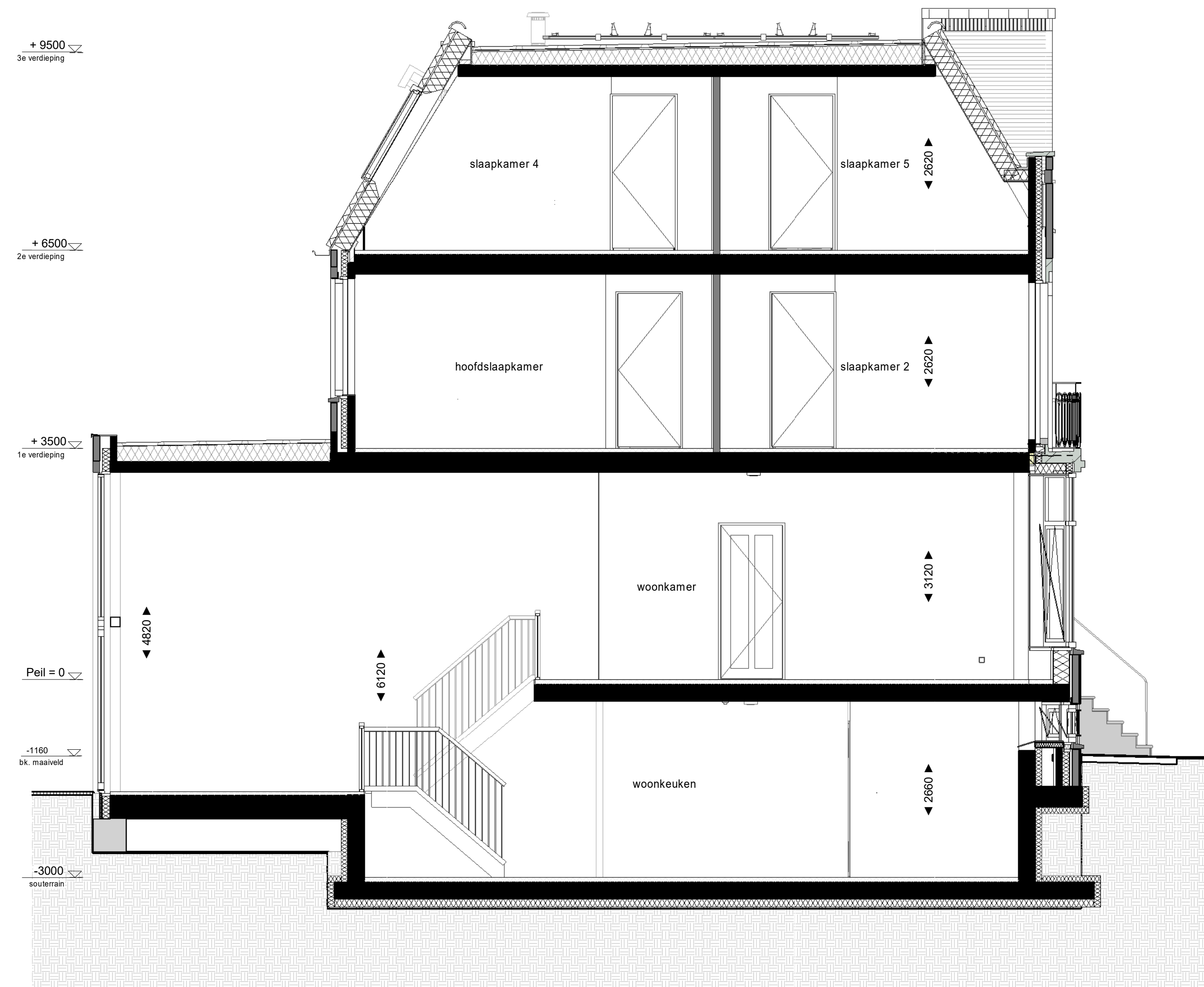
Doorsnede 1 : 50
