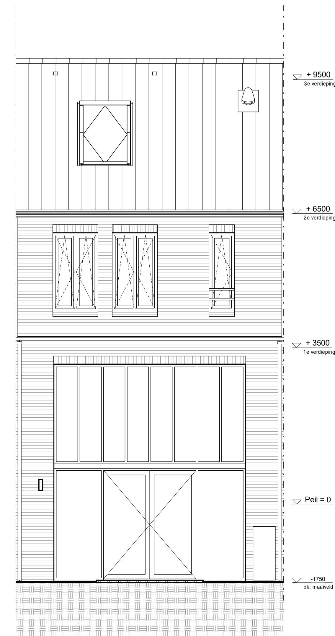
Achtergevel 1 : 50
