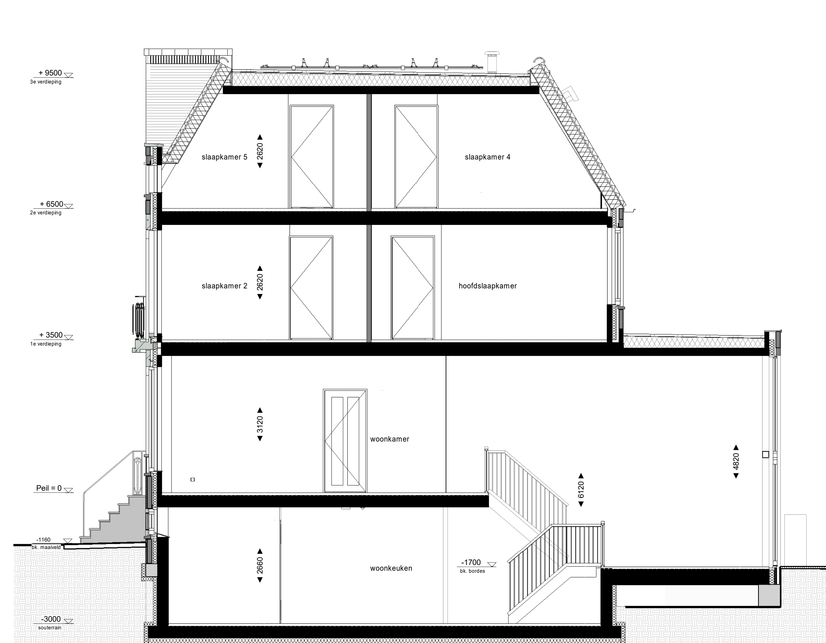
Doorsnede 1 : 50
