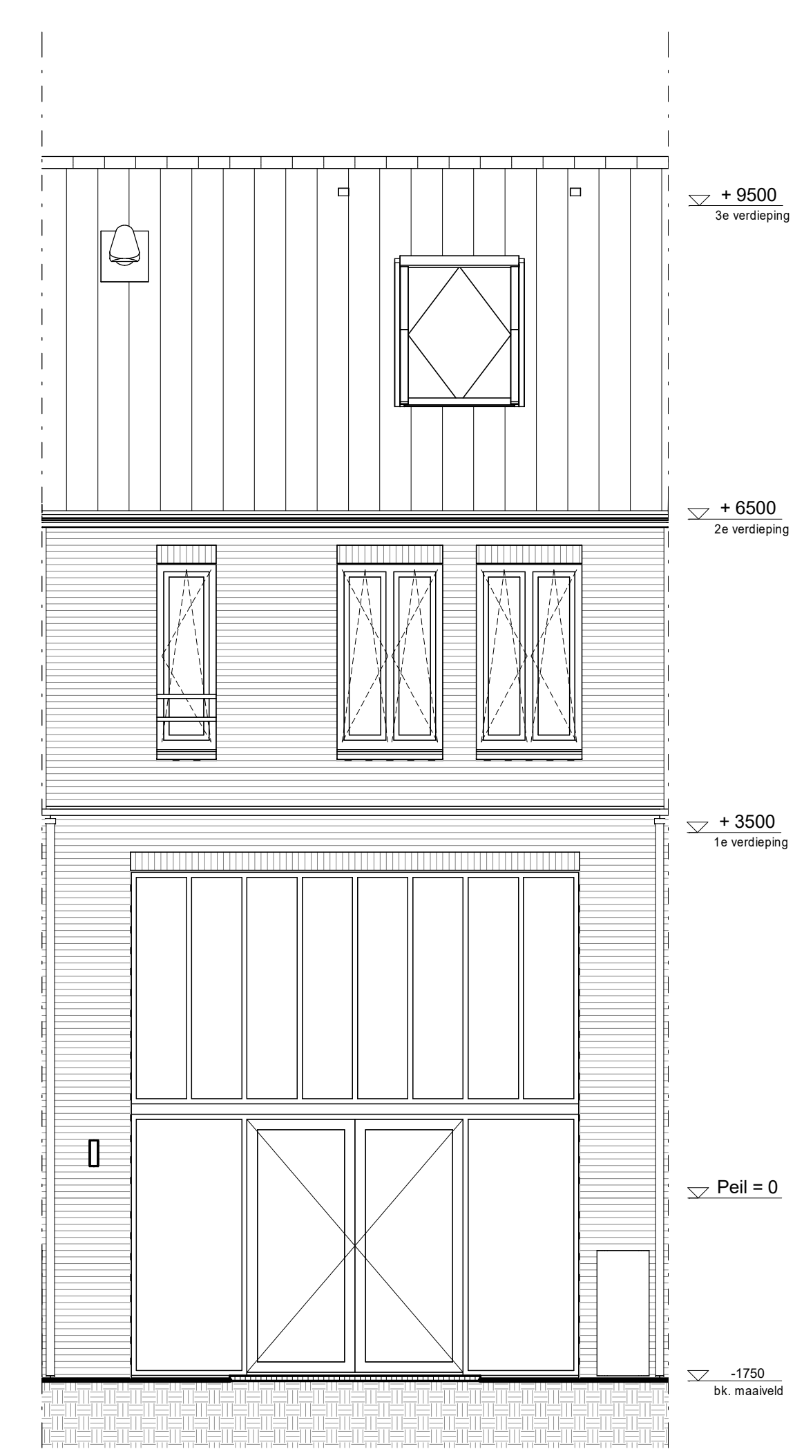
Achtergevel 1 : 50
