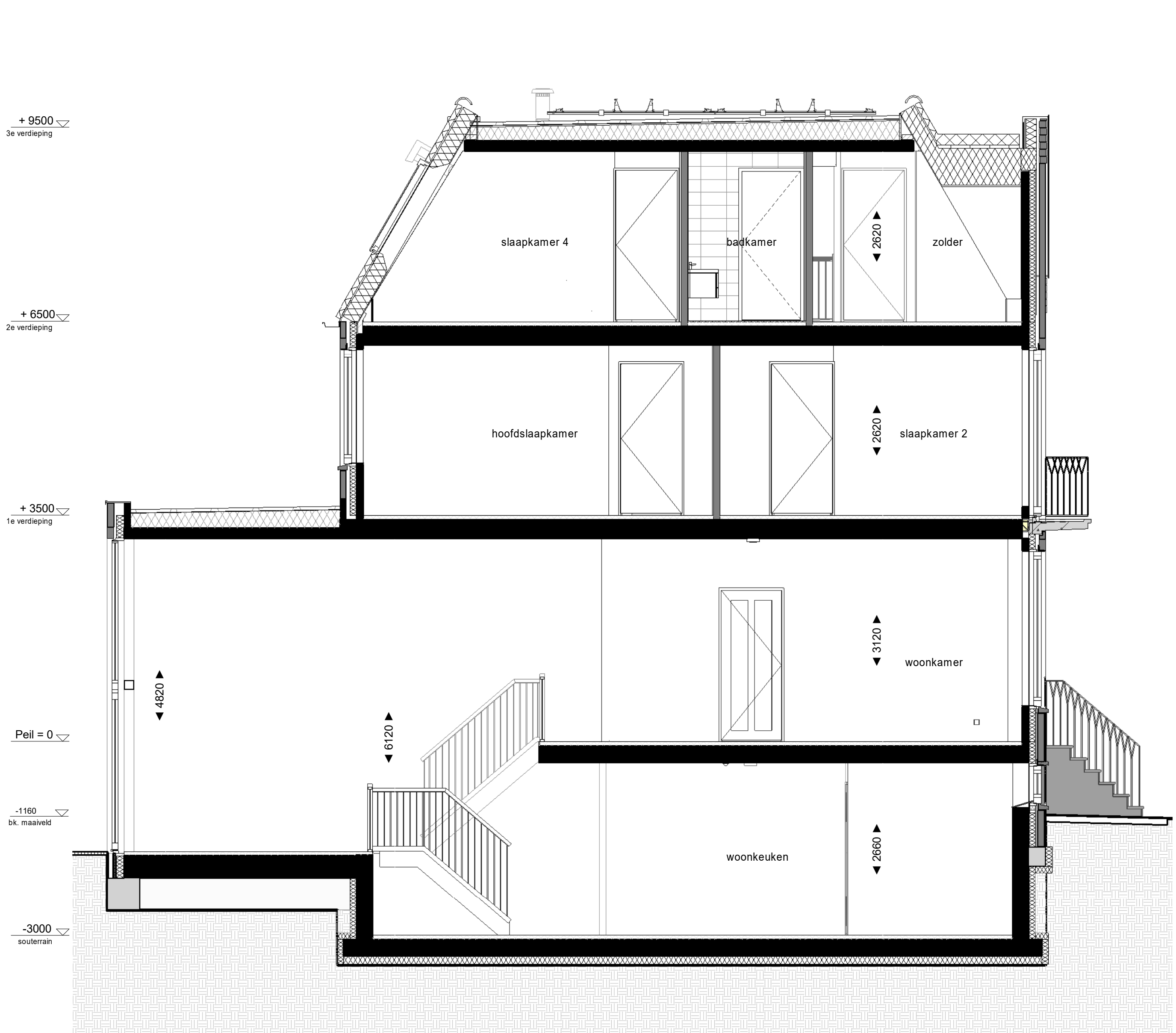
Doorsnede 1 : 50
