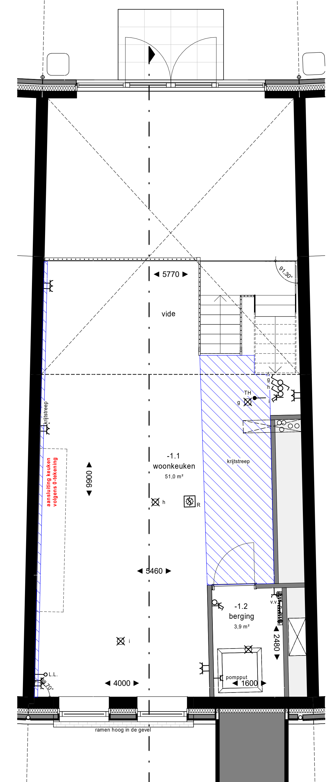
Souterrain 1 : 50
