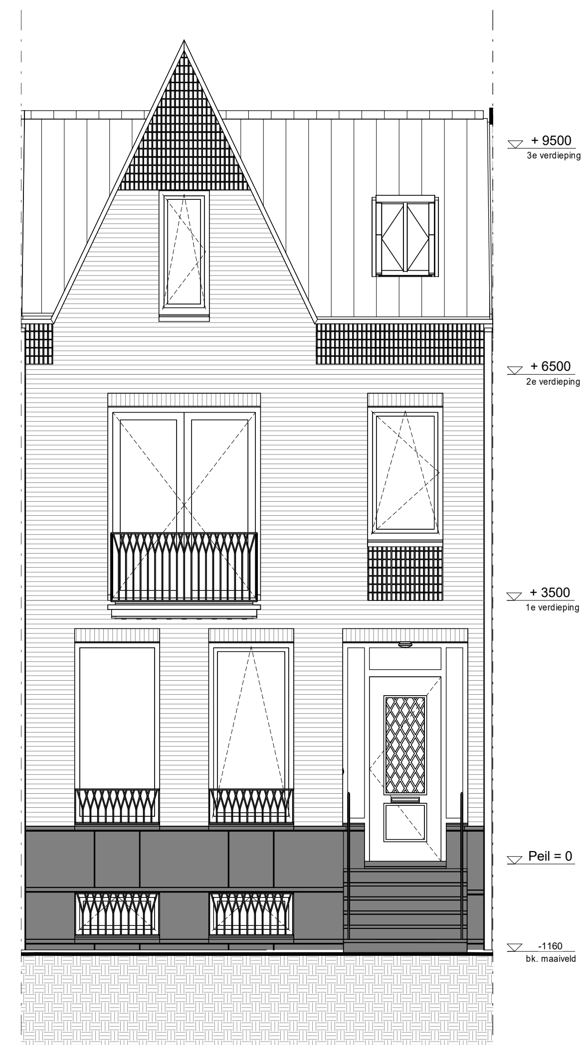
Voorgevel 1 : 50
