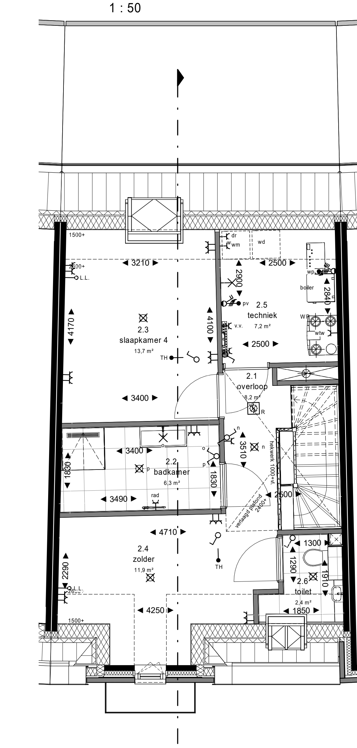
2e verdieping 1 : 50
