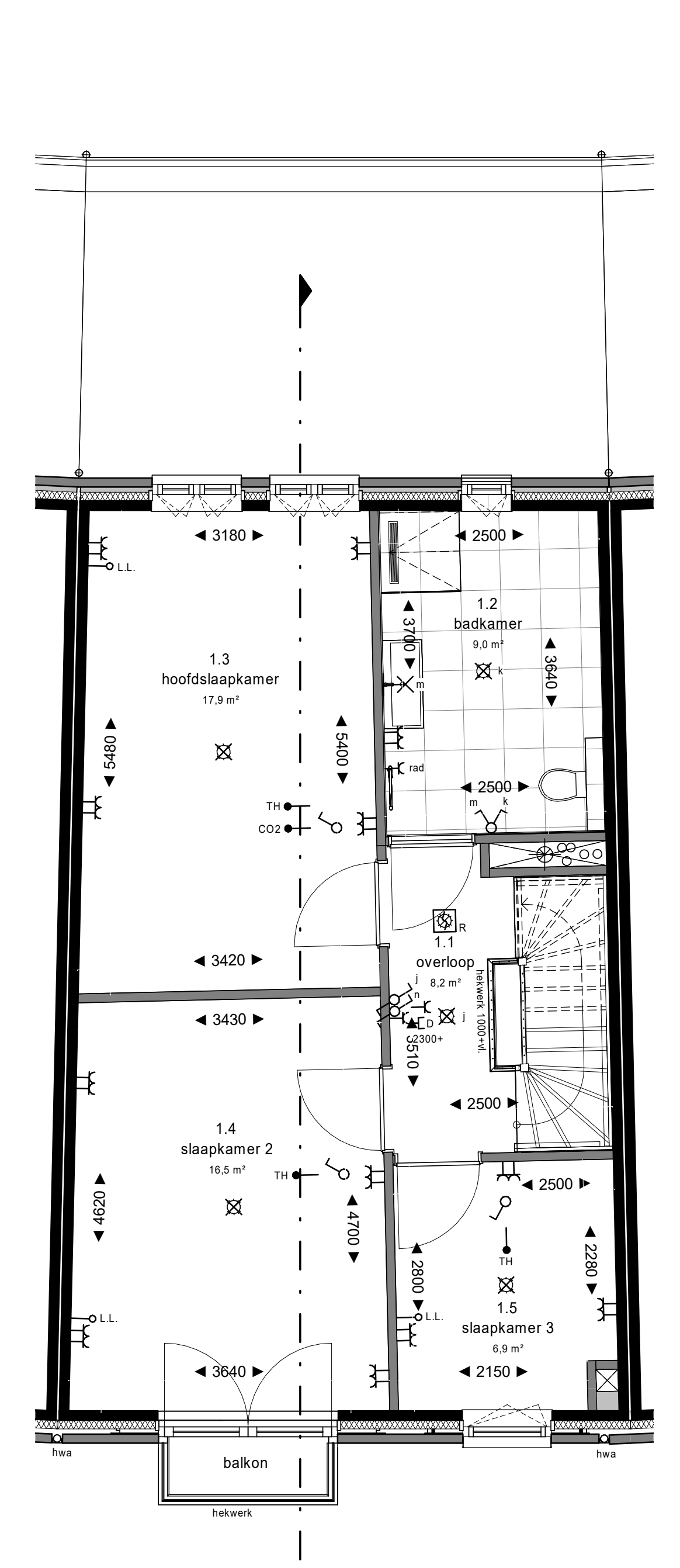
1e verdieping 1 : 50
