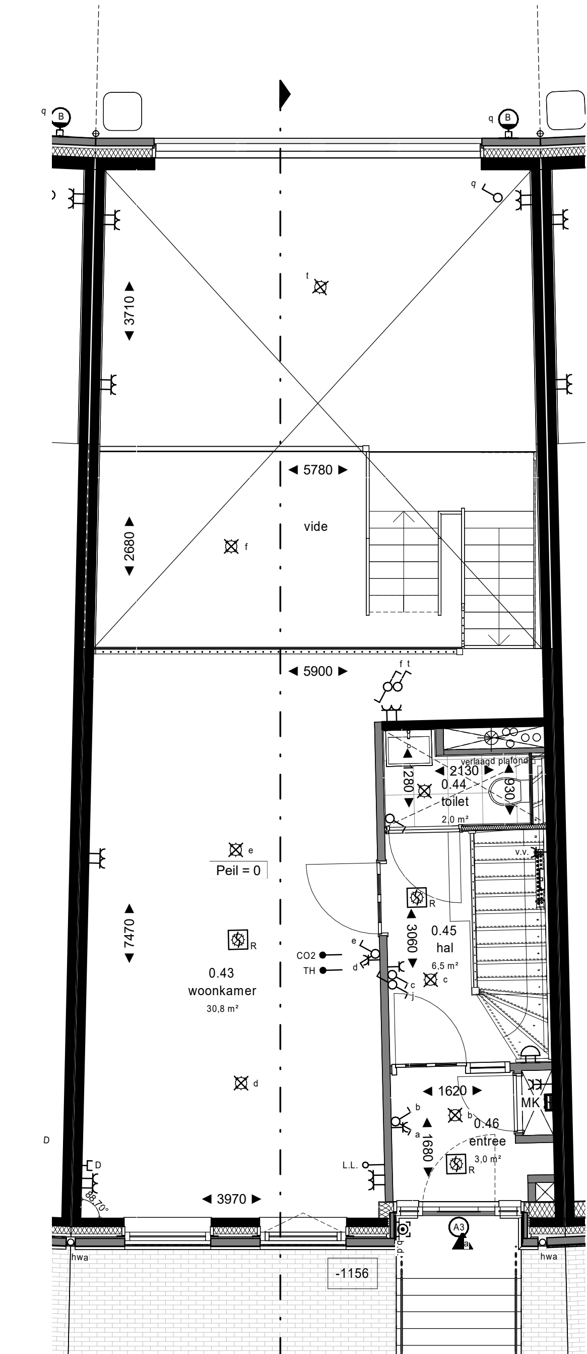
Begane grond 1 : 50
