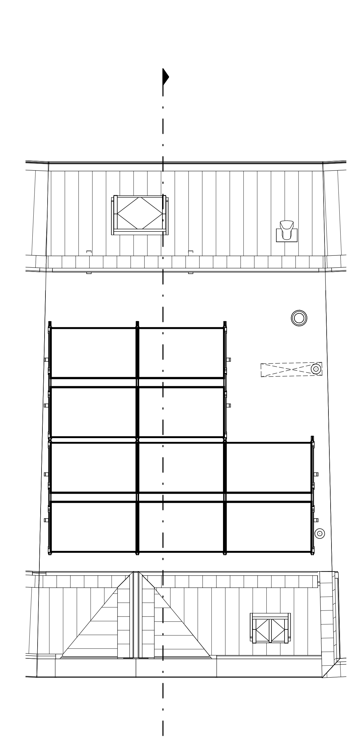
Dakplattegrond 1 : 50
