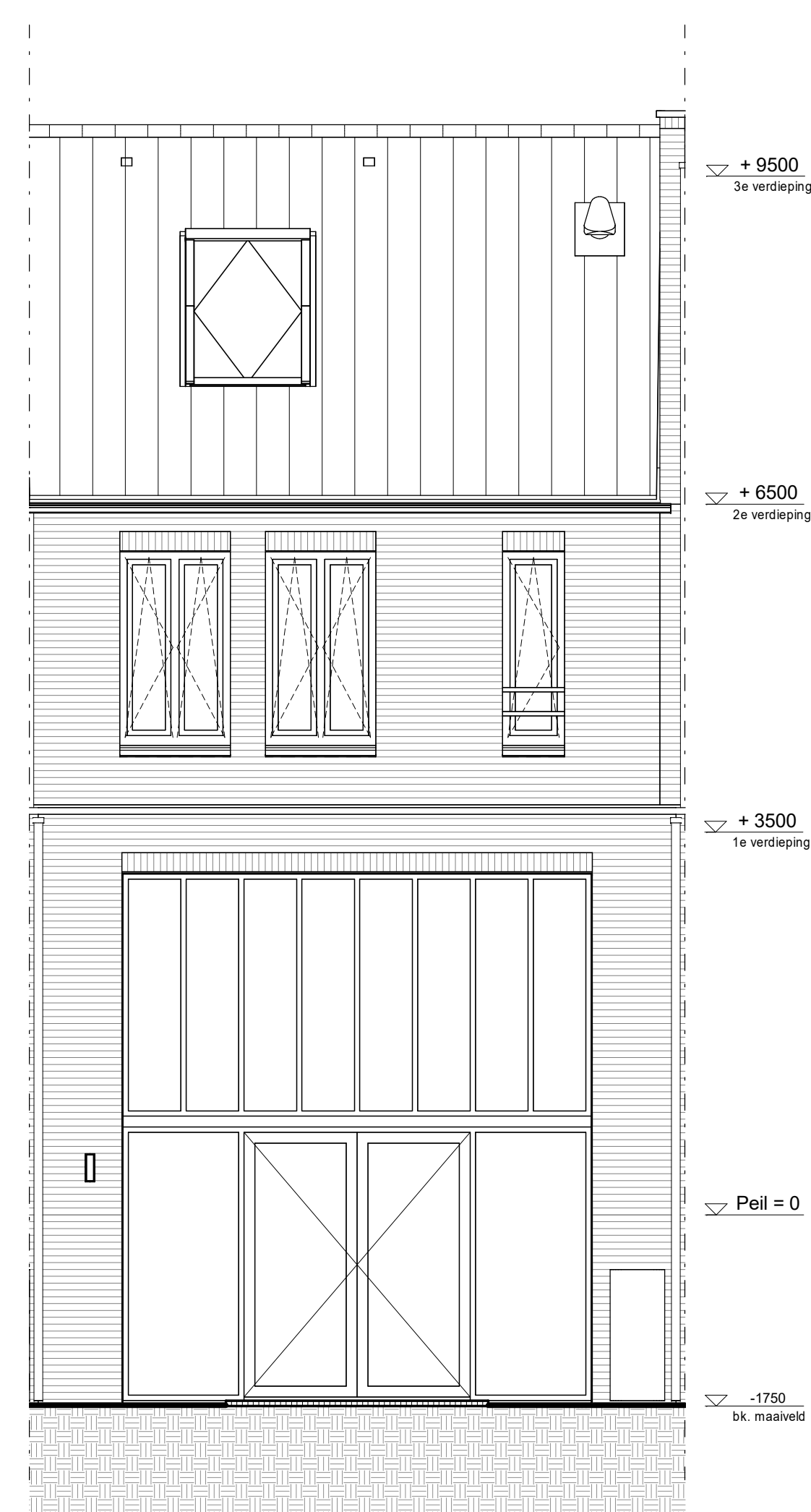
Achtergevel 1 : 50
