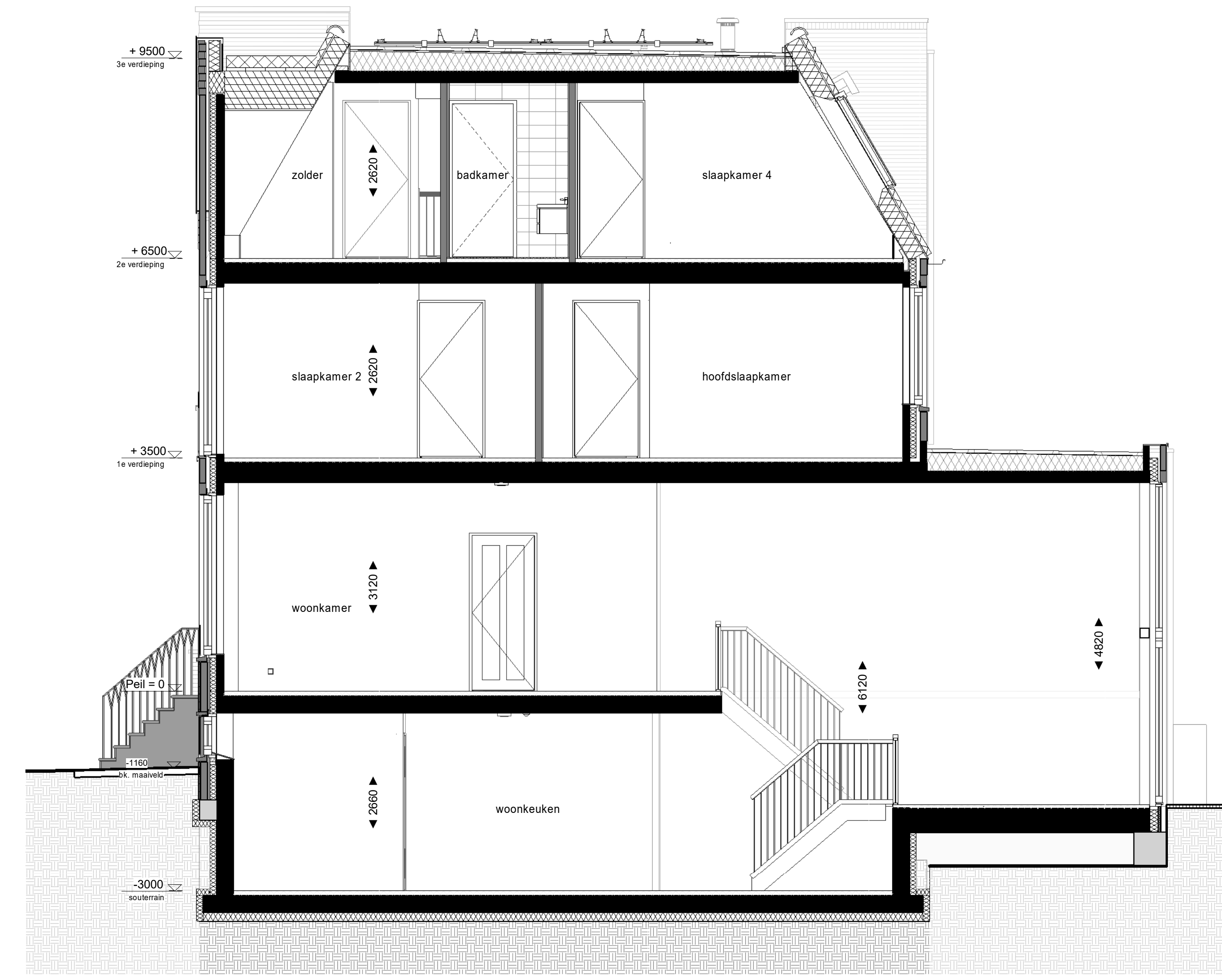
Doorsnede 1 : 50
