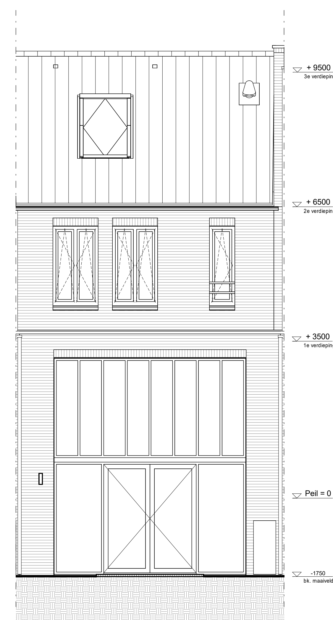
Achtergevel 1 : 50
