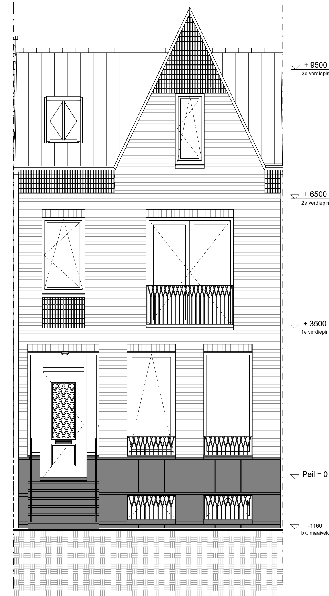
Voorgevel 1 : 50
