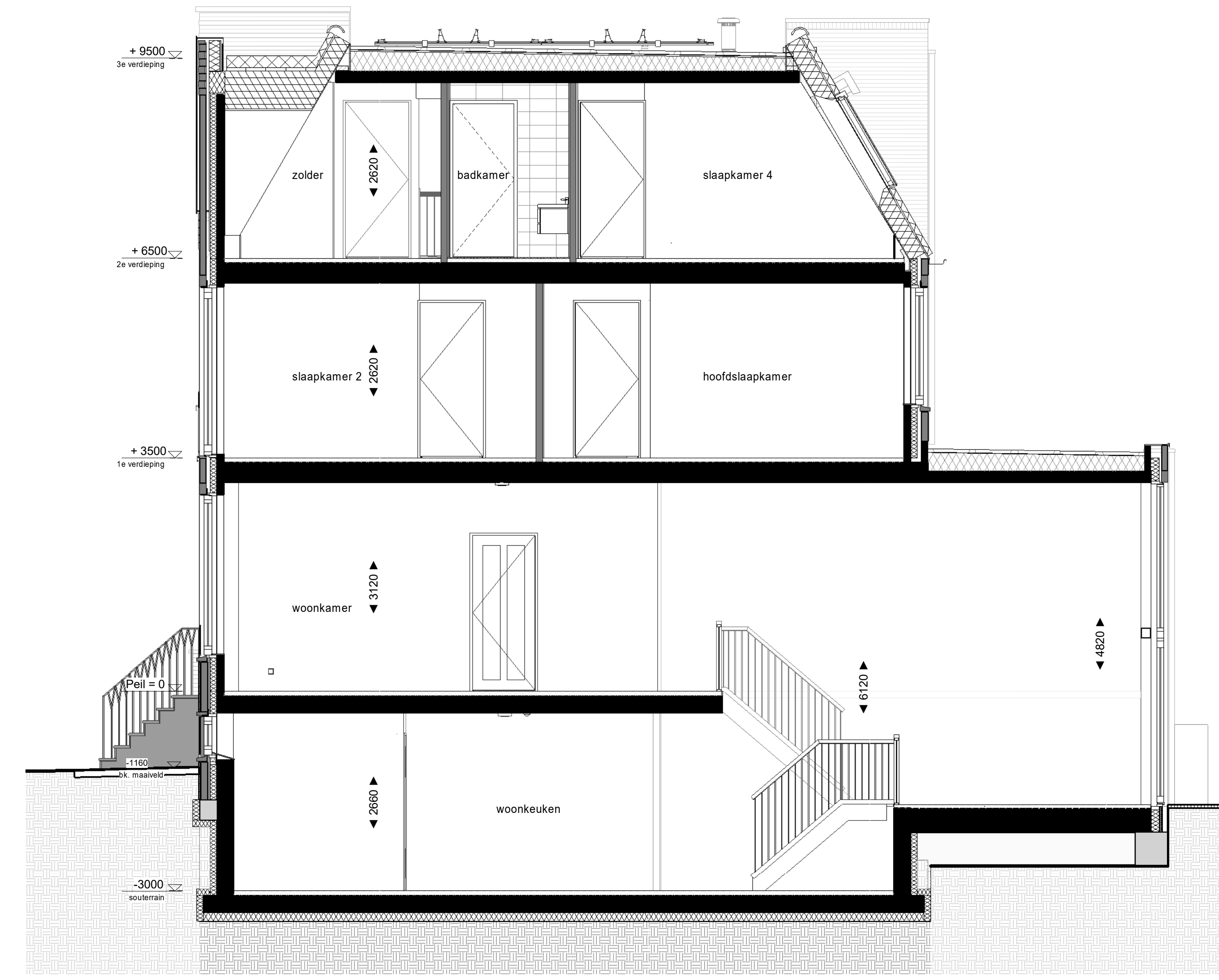
Doorsnede 1 : 50
