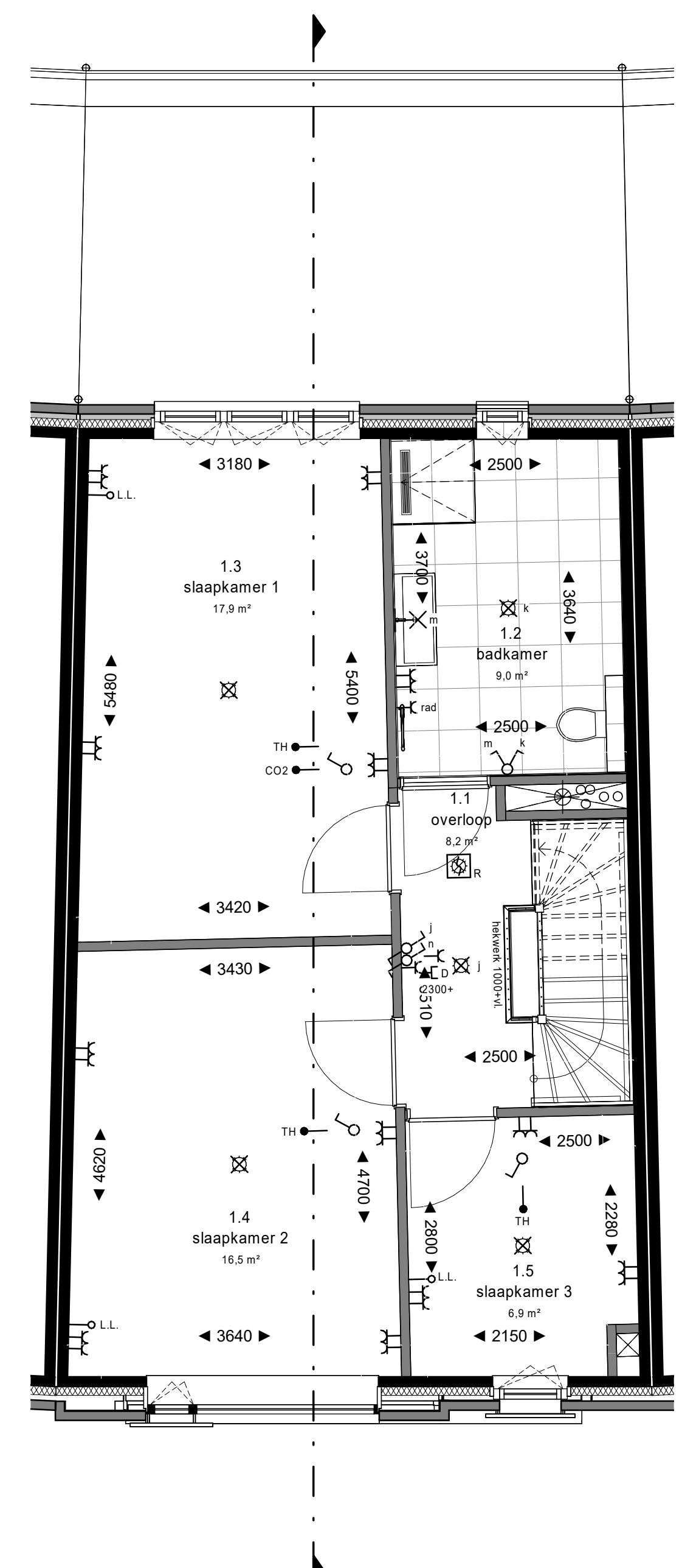
1e verdieping 1 : 50
