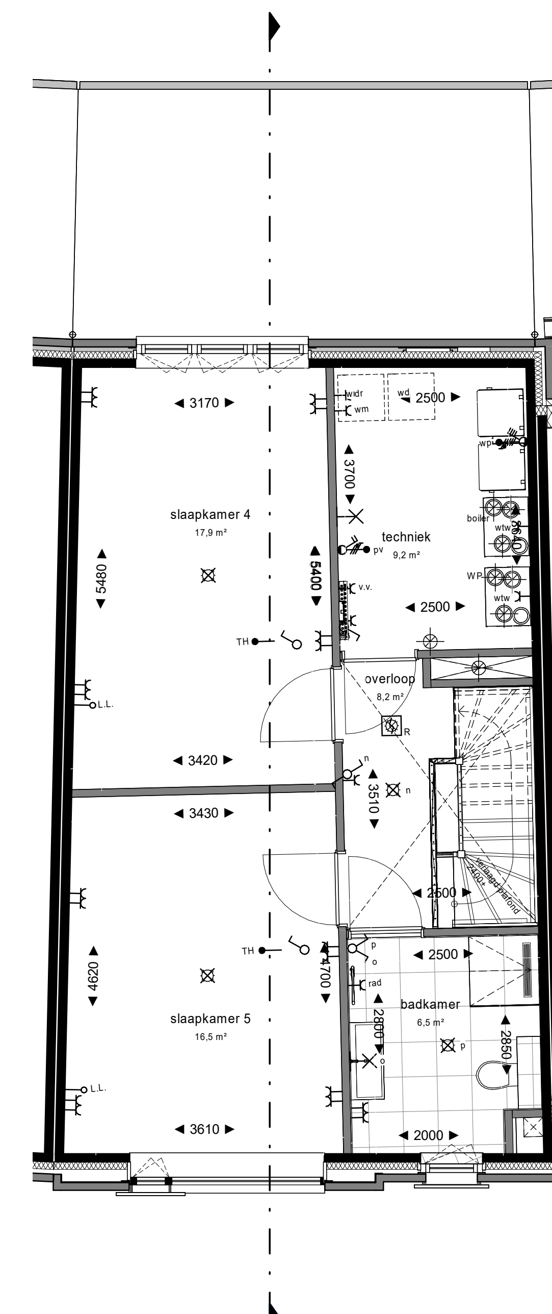
2e verdieping 1 : 50
