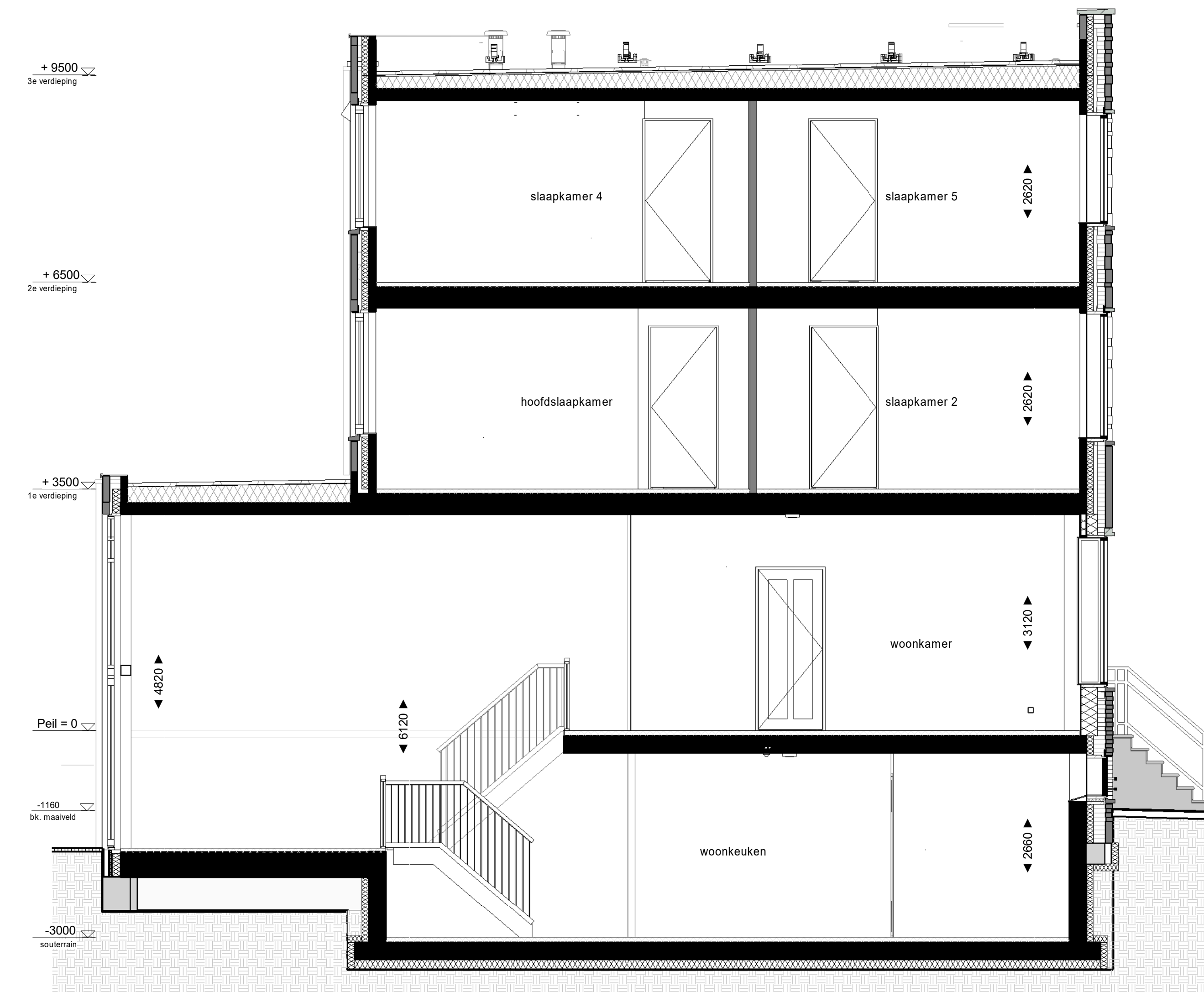
Doorsnede 1 : 50
