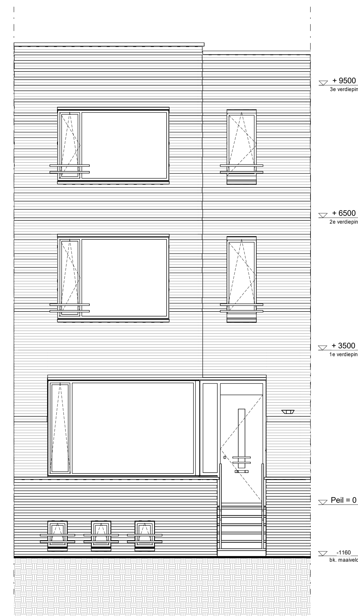
Voorgevel 1 : 50
