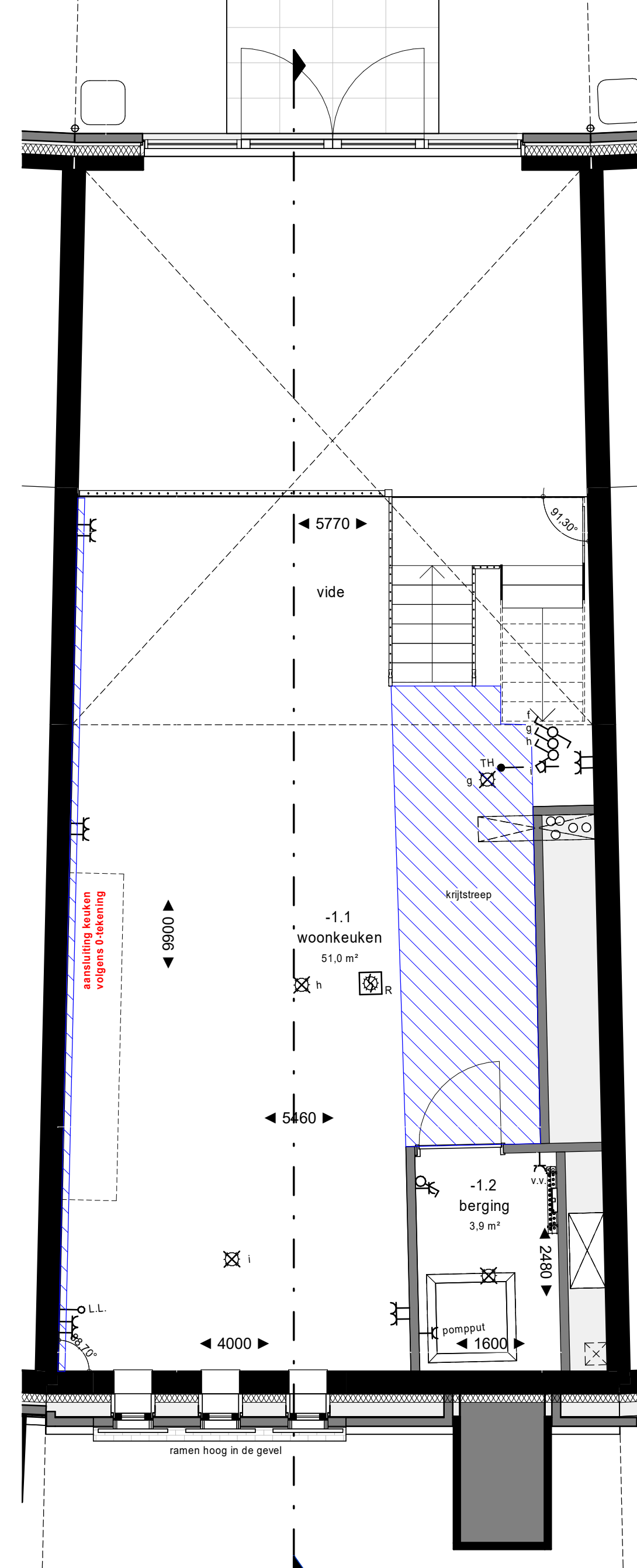
Souterrain 1 : 50
