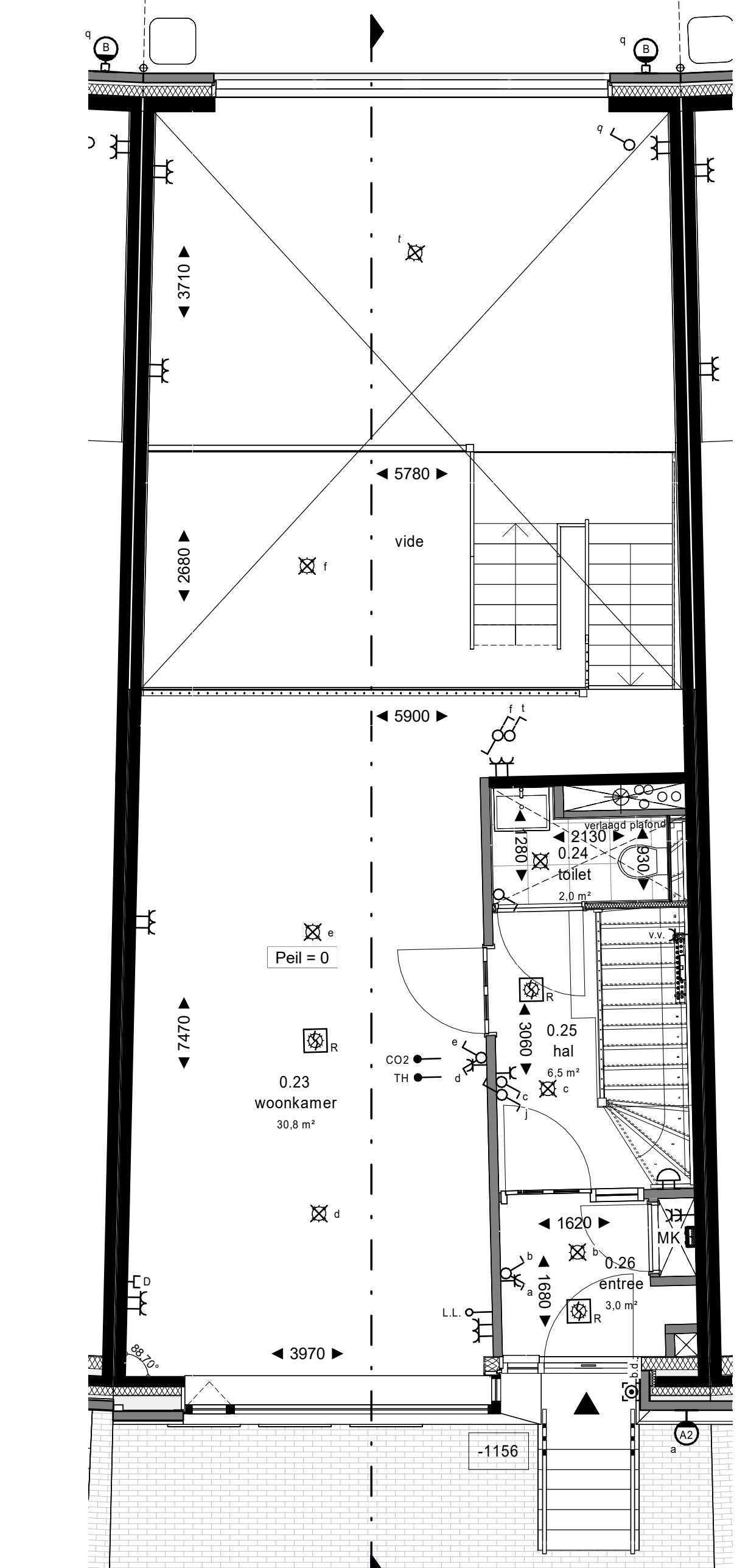
Begane grond 1 : 50
