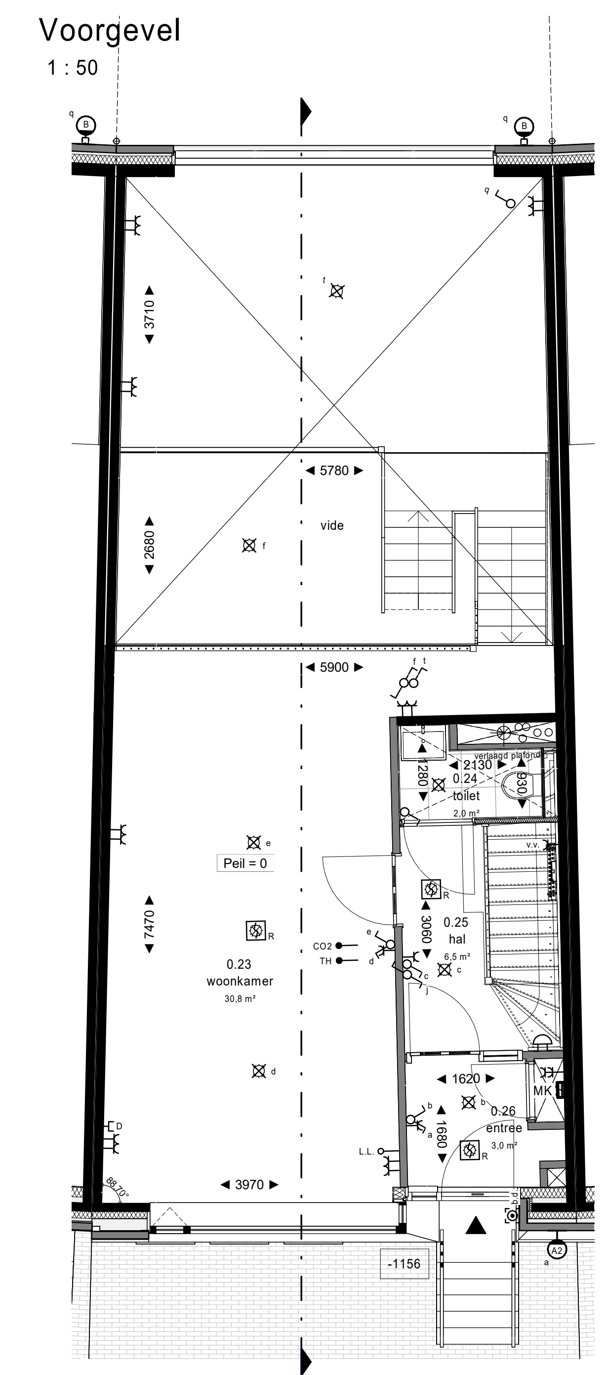
Begane grond 1 : 50
