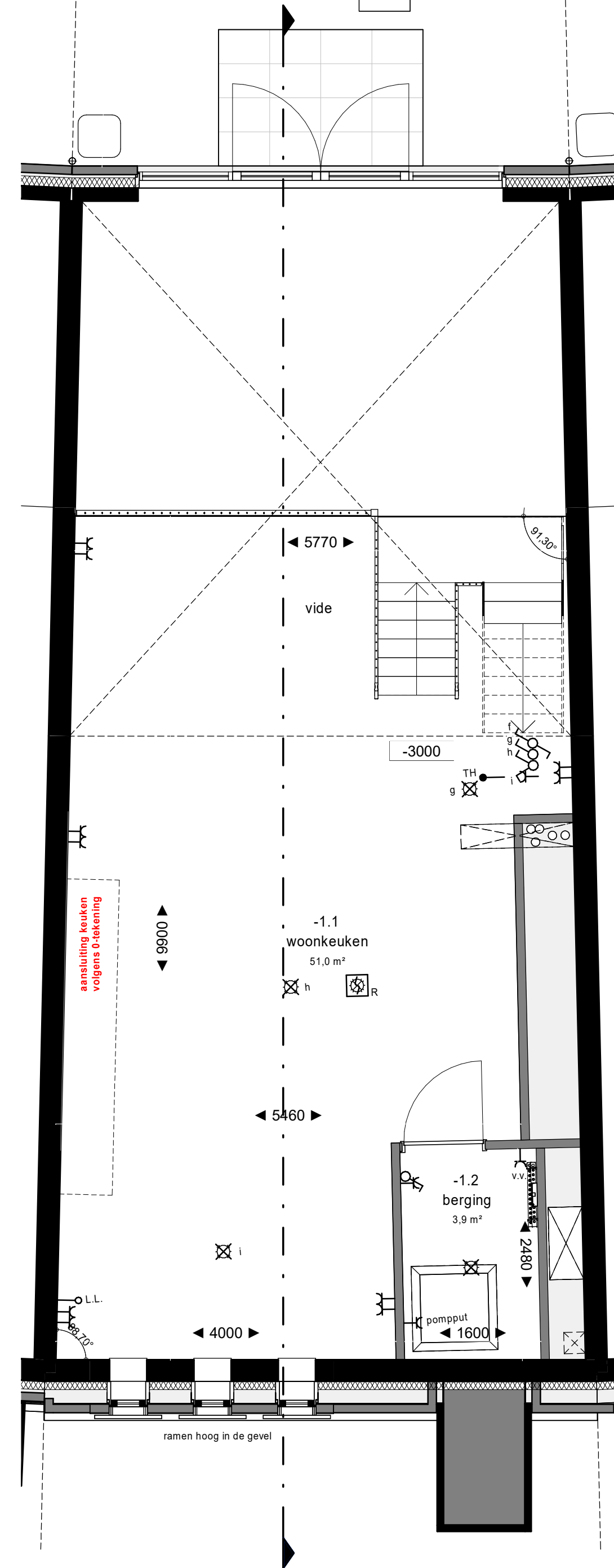
Souterrain 1 : 50
