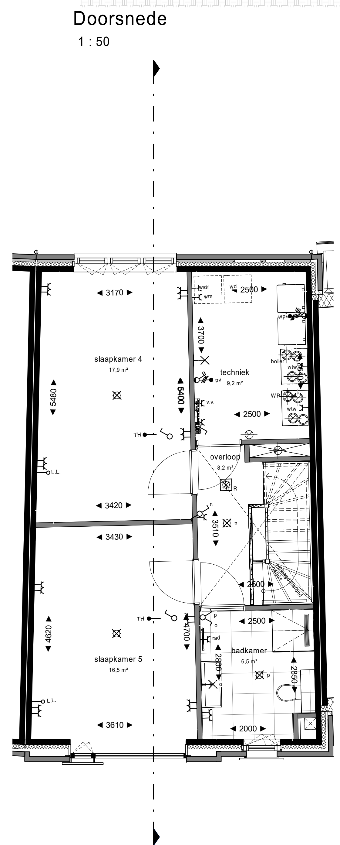
2e verdieping 1 : 50
