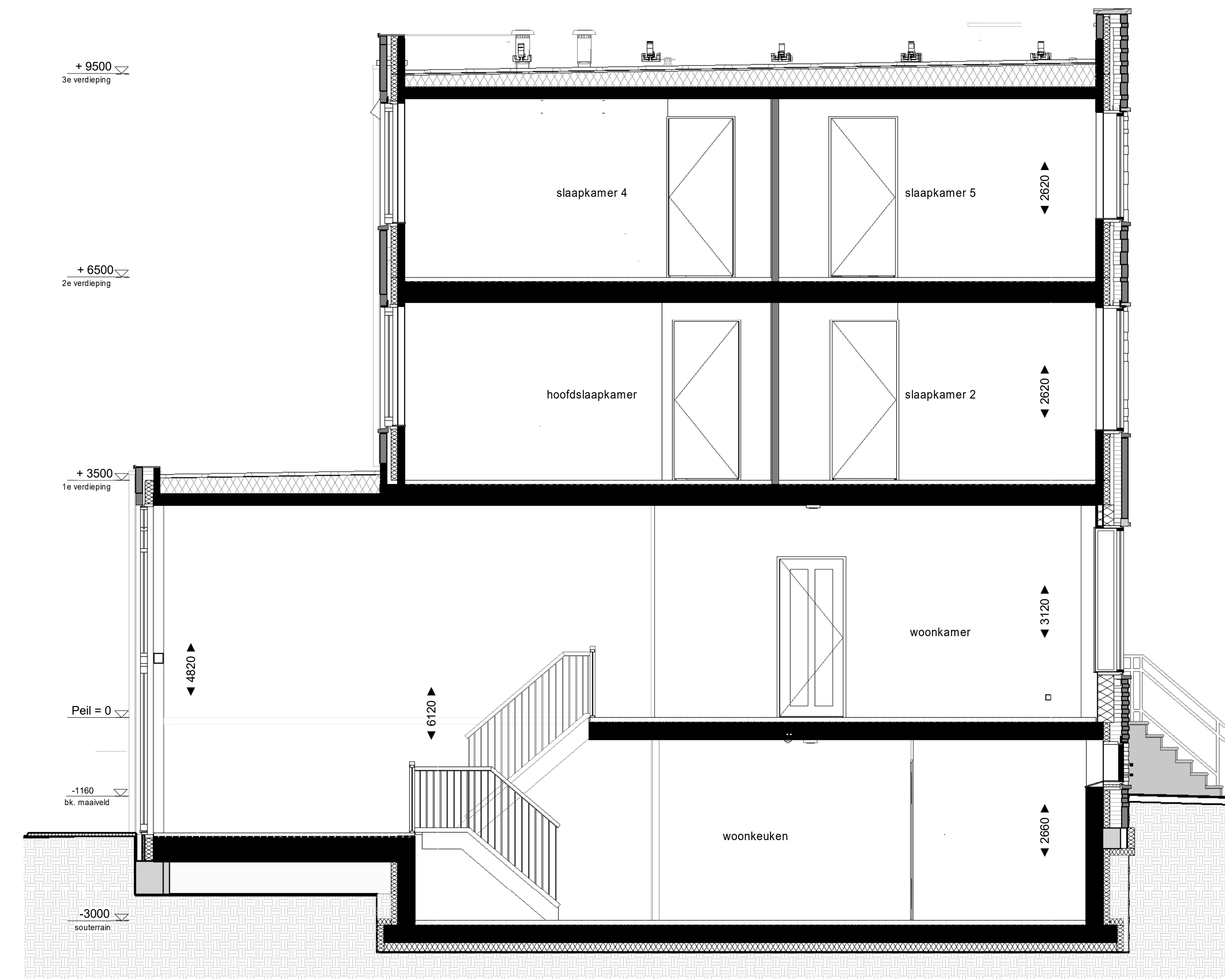
Doorsnede 1 : 50
