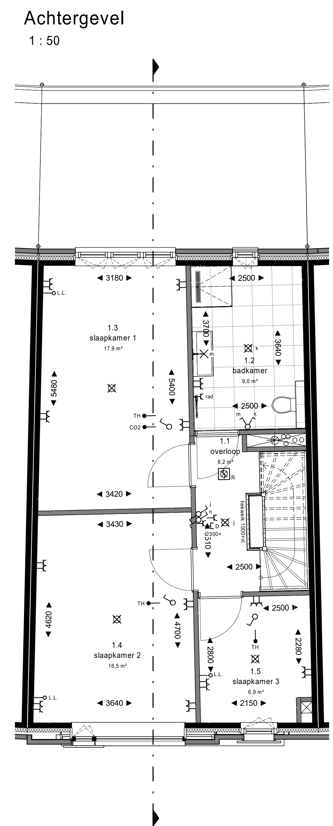
1e verdieping 1 : 50
