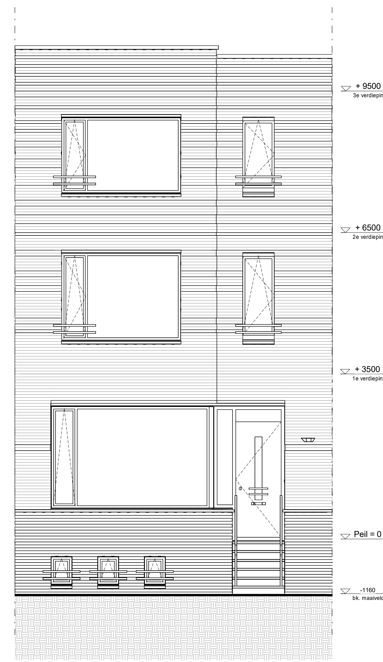
Voorgevel 1 : 50
