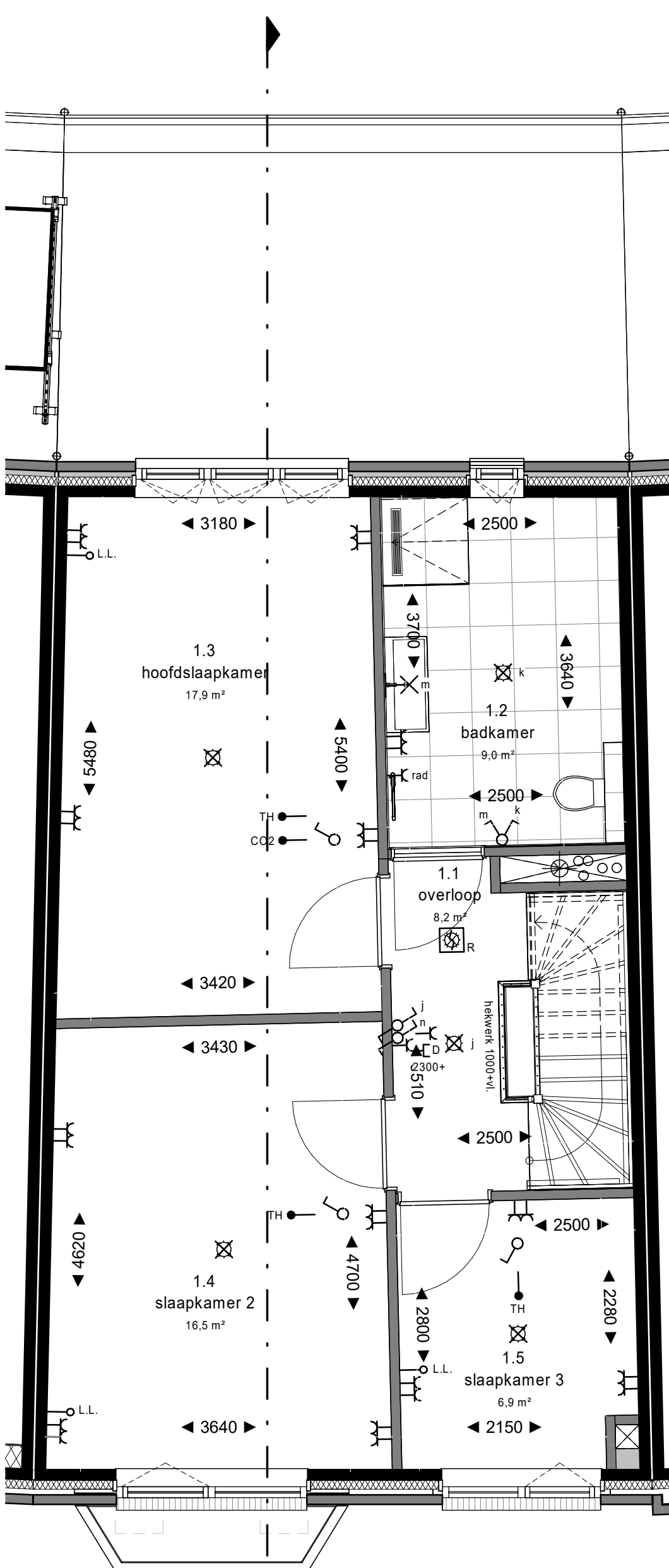
1e verdieping 1 : 50
