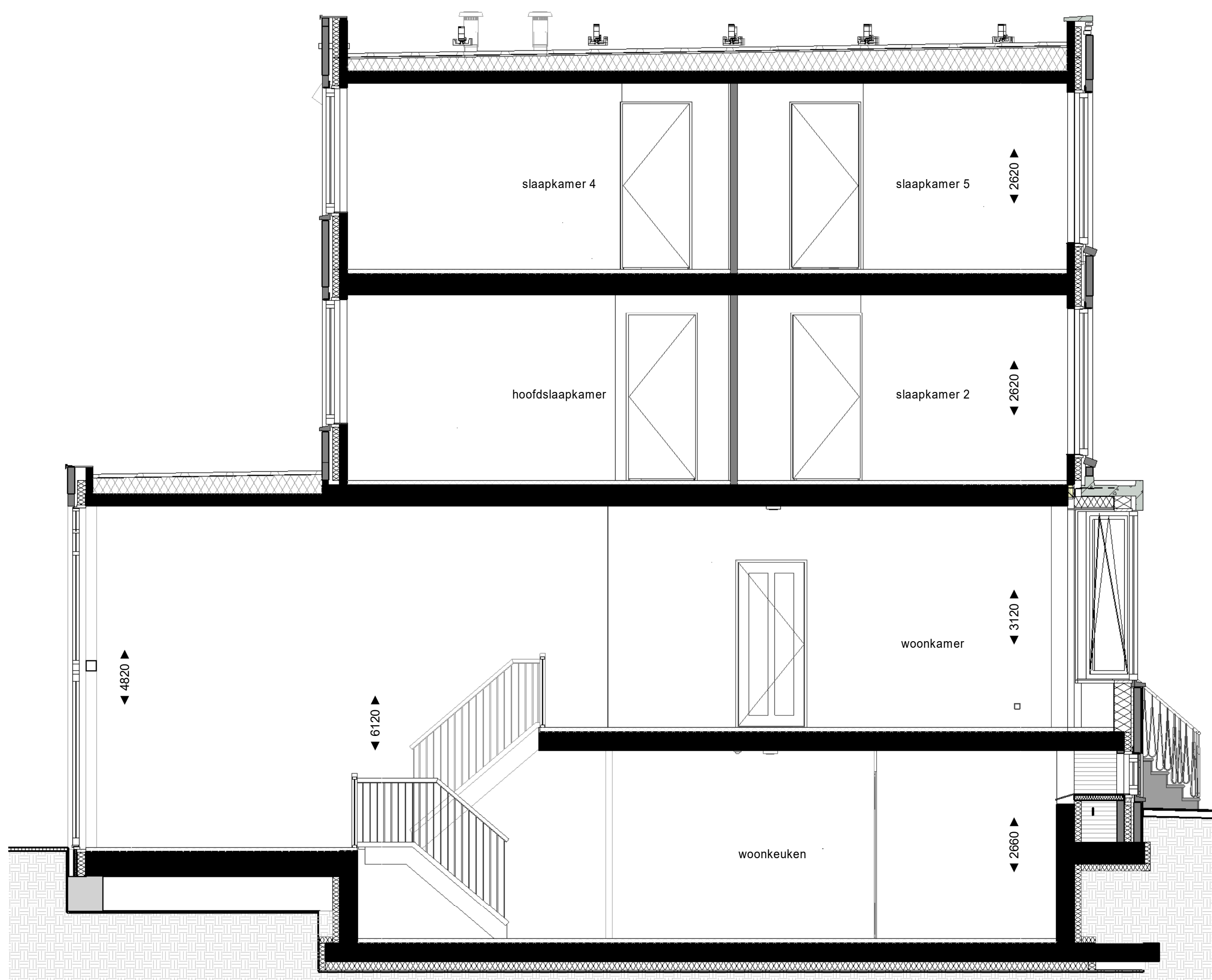
Doorsnede 1 : 50
