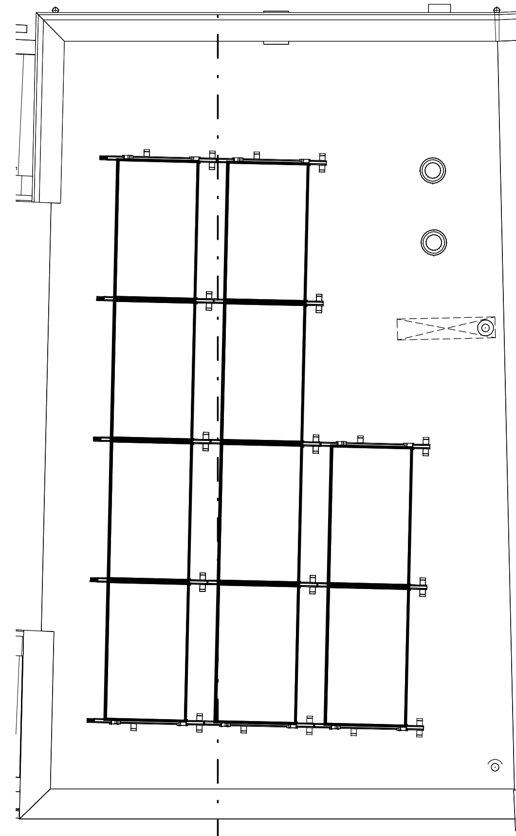
Dakplattegrond 1 : 50
