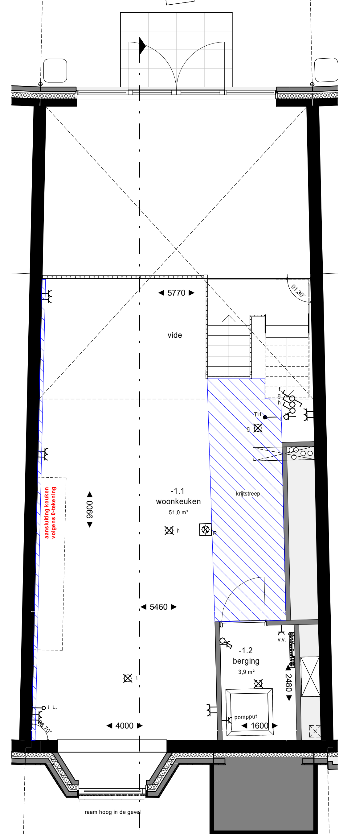
Souterrain 1 : 50
