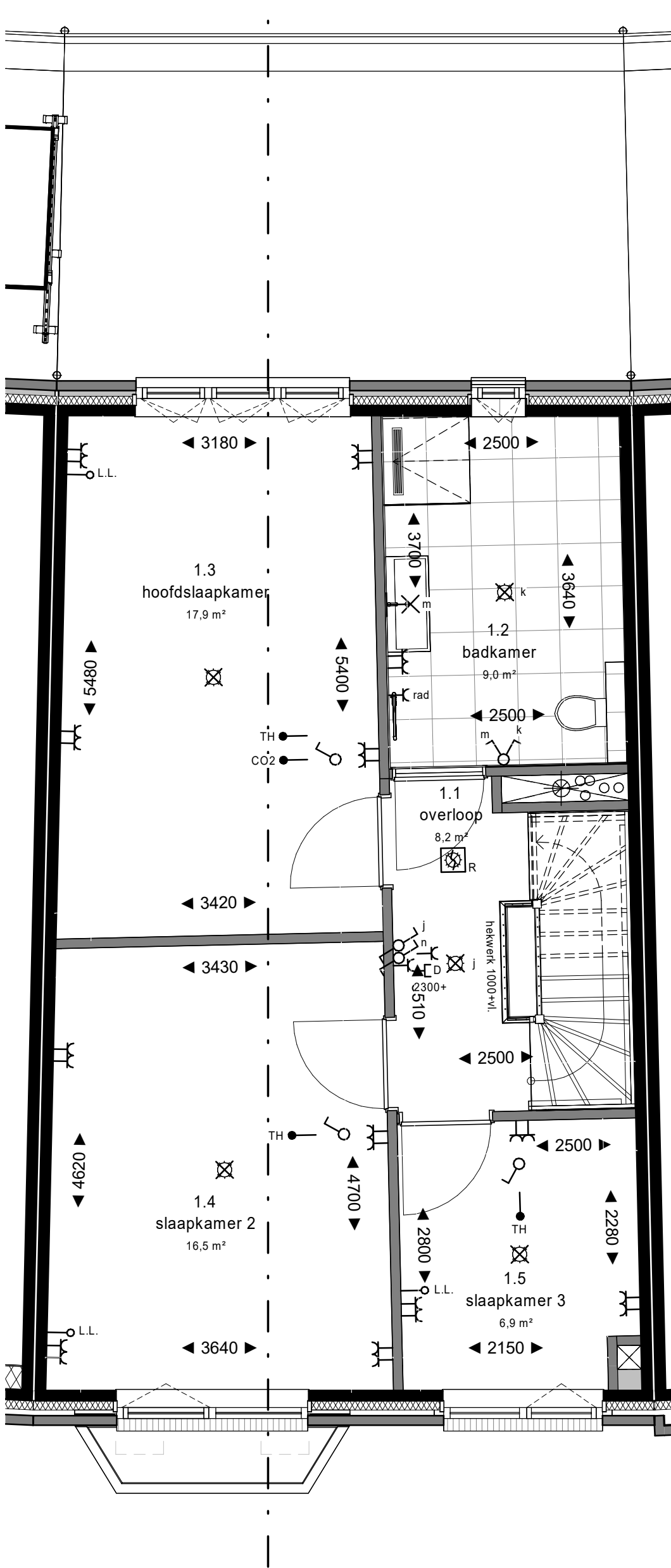
1e verdieping 1 : 50
