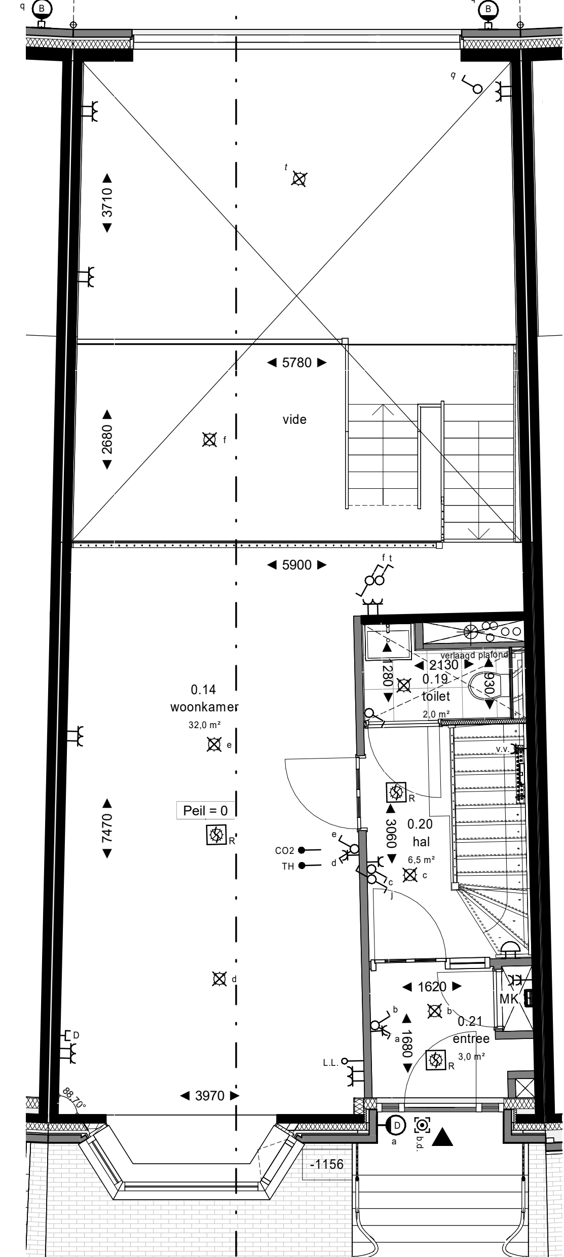
Begane grond 1 : 50
