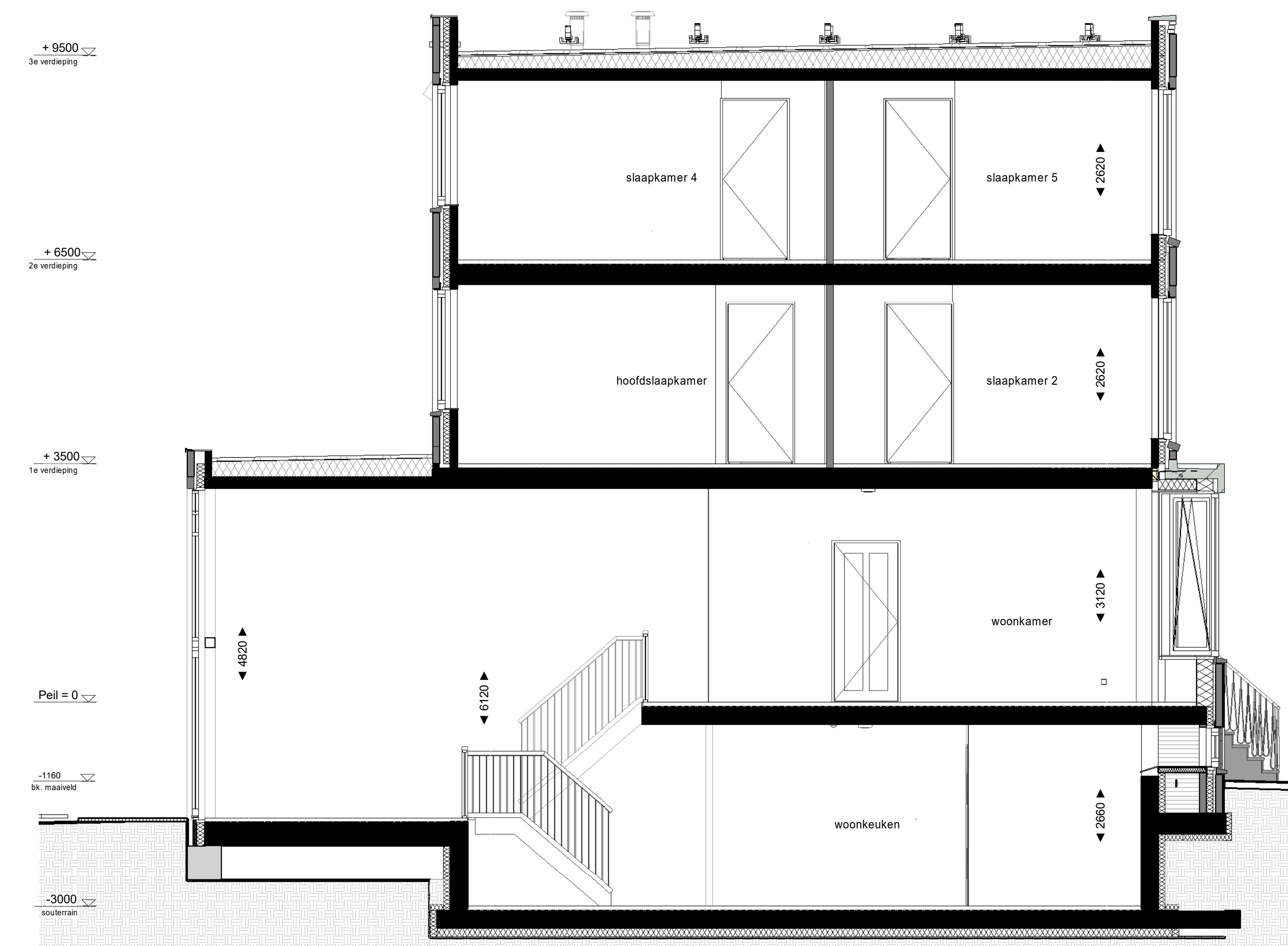
Doorsnede 1 : 50
