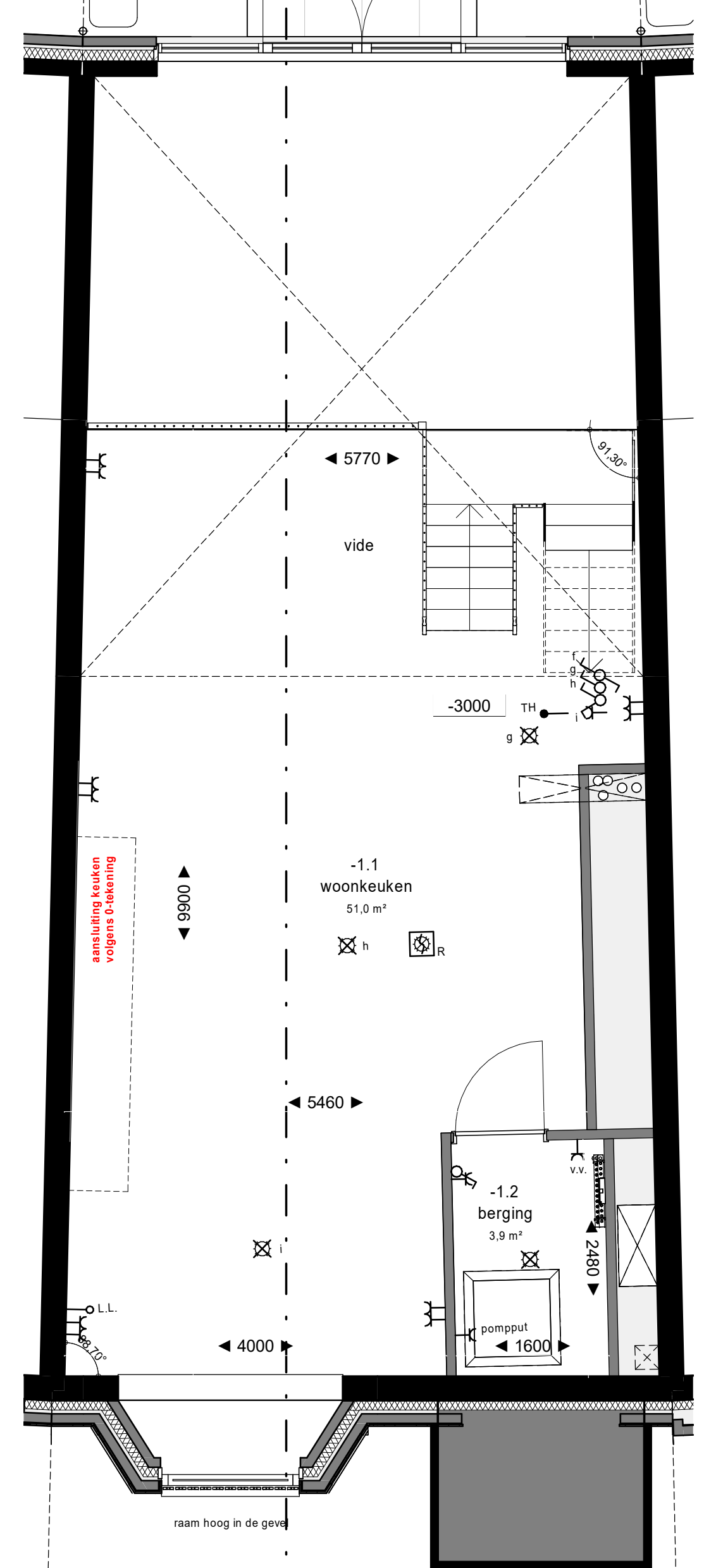
Souterrain 1 : 50
