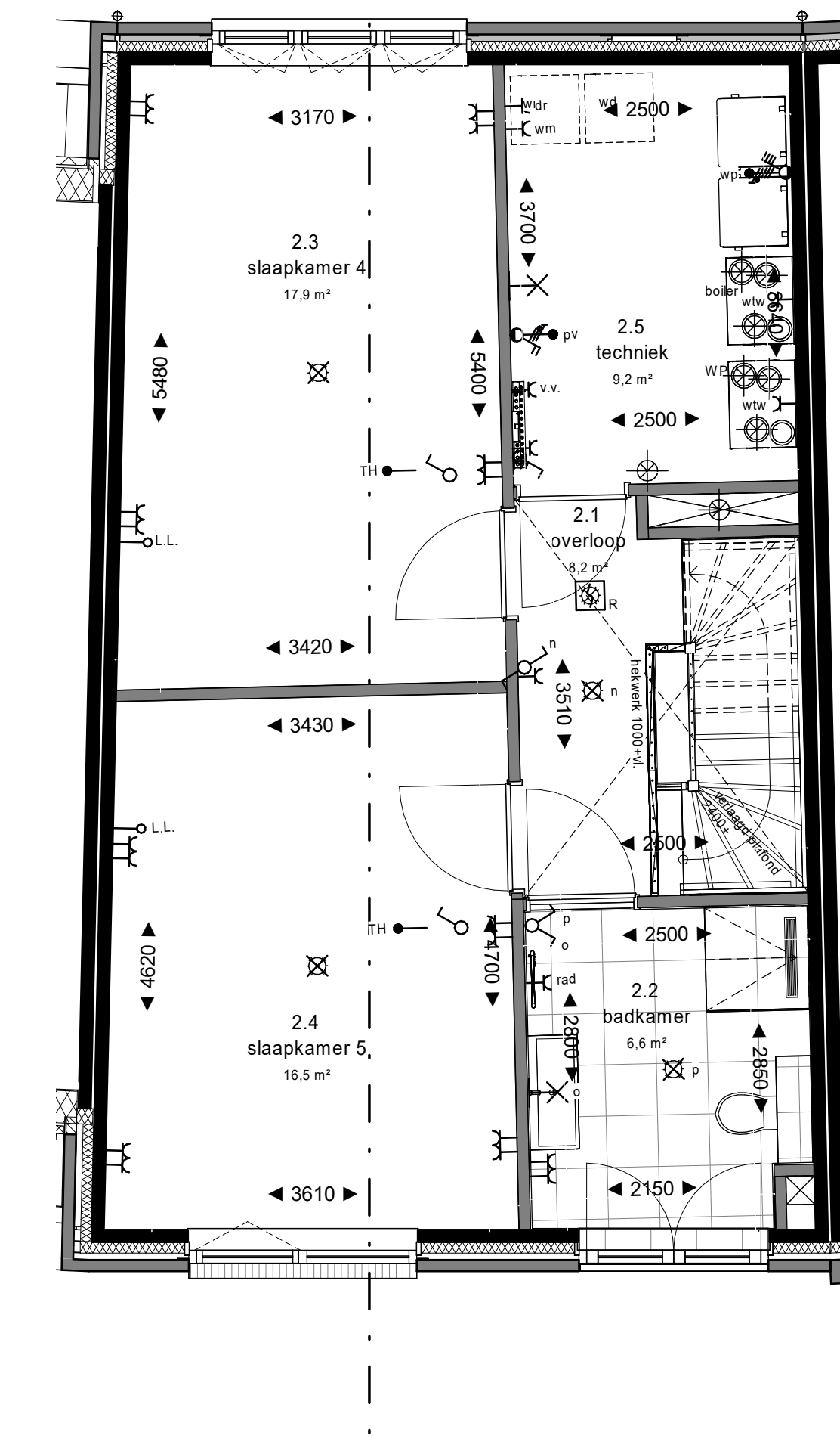
2e verdieping 1 : 50
