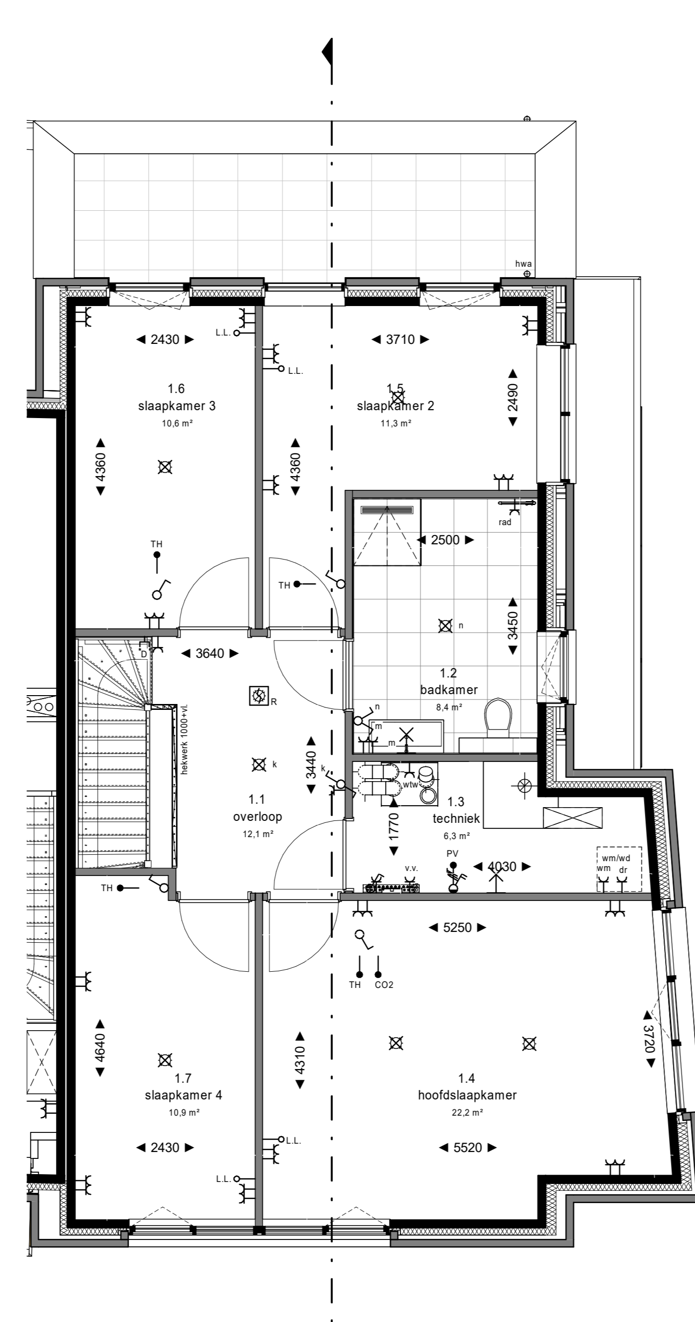
1e verdieping 1 : 50
