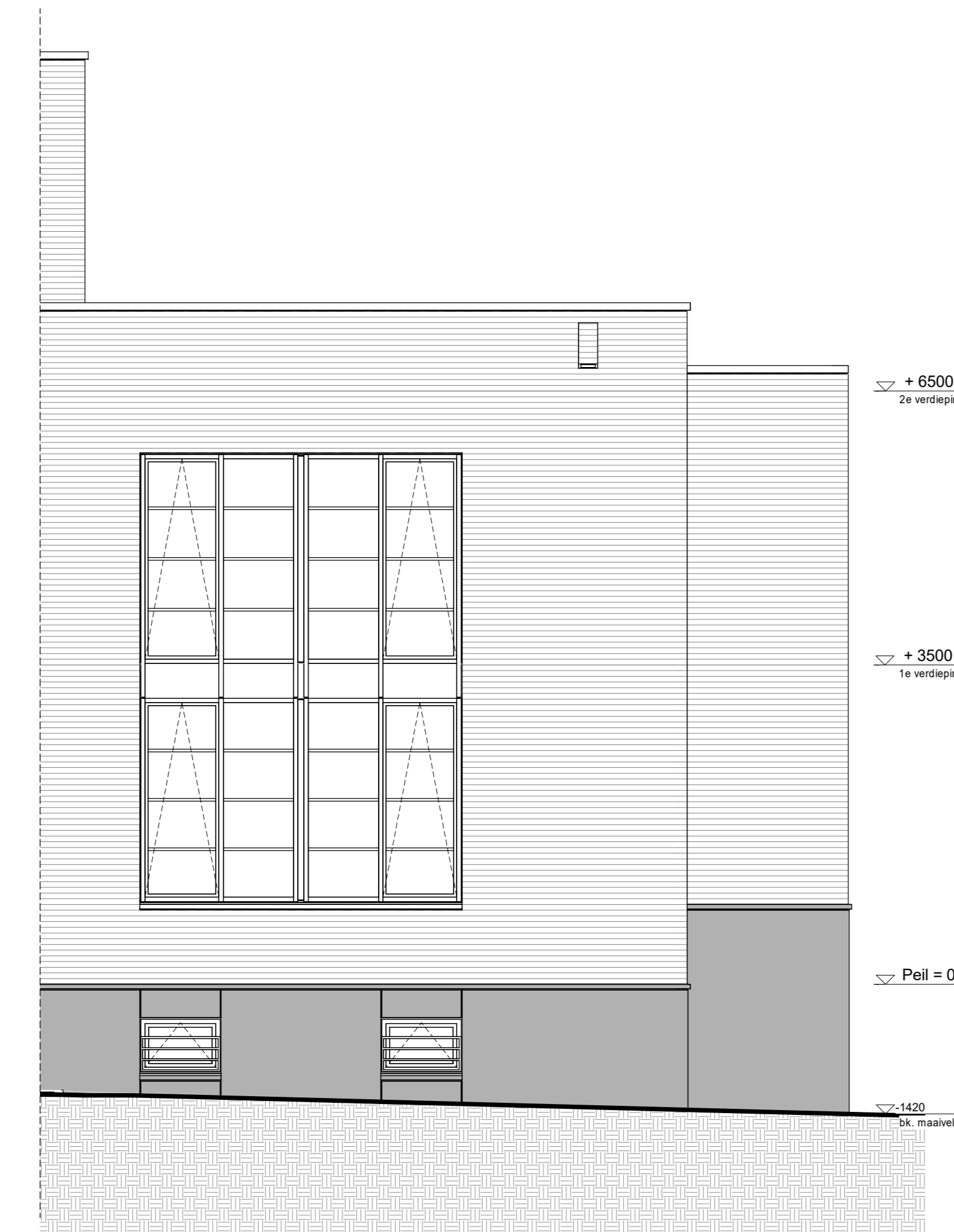
Voorgevel 1 : 50
