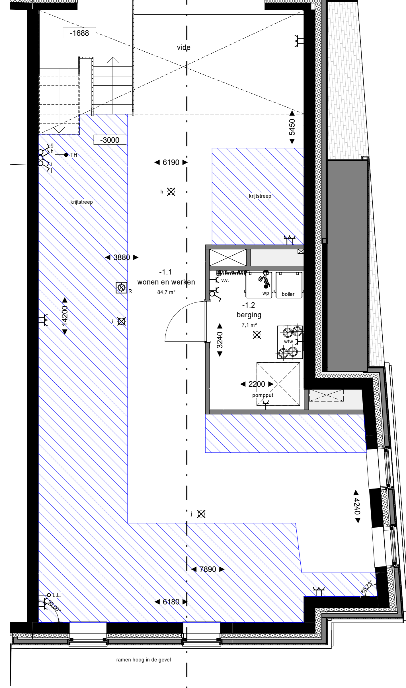
Souterrain 1 : 50
