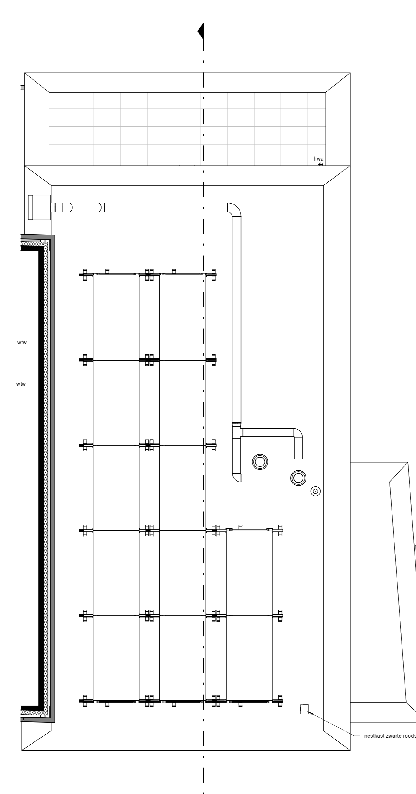
Dakplaattegrond 1 : 50
