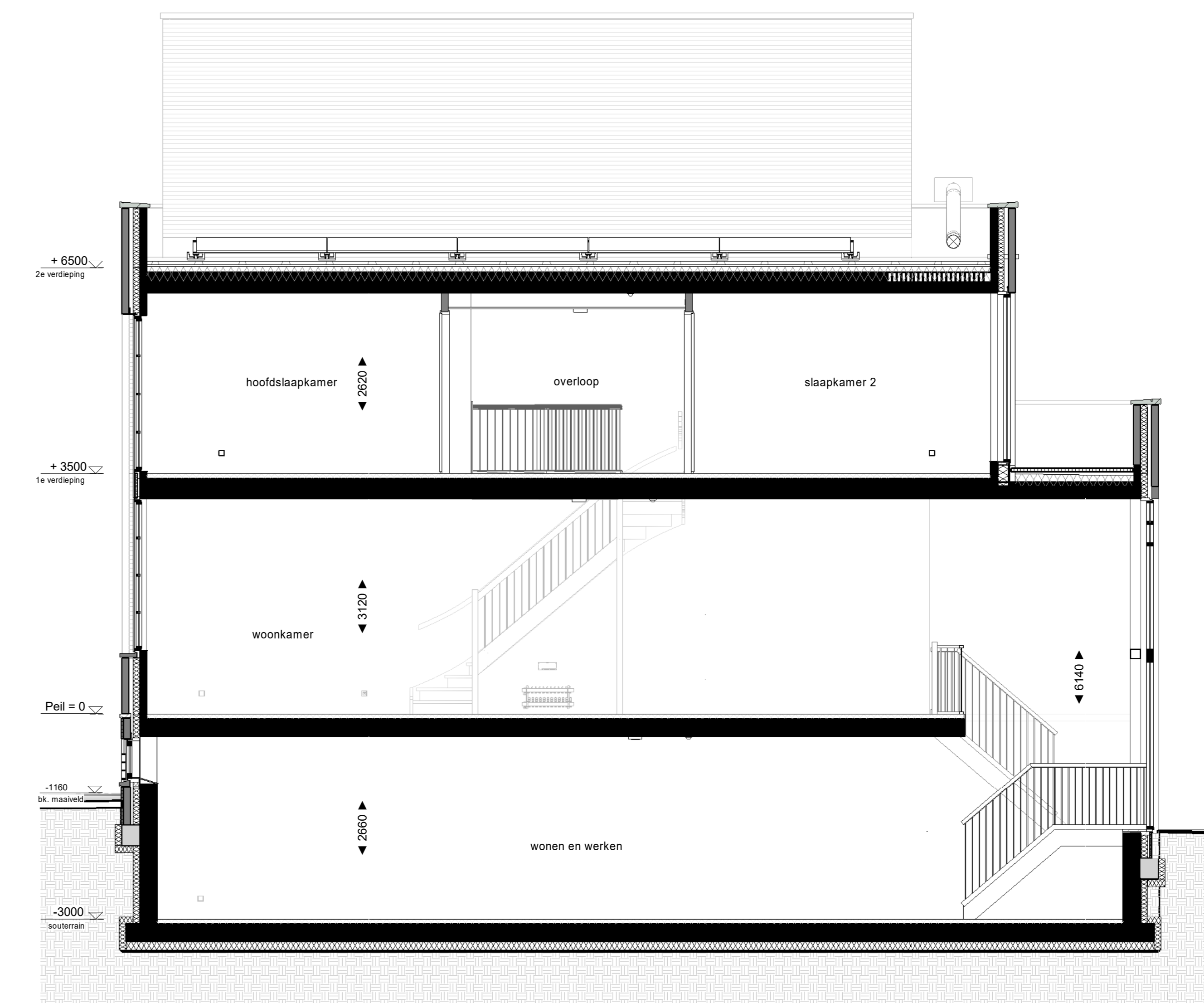
Doorsnede 1 : 50
