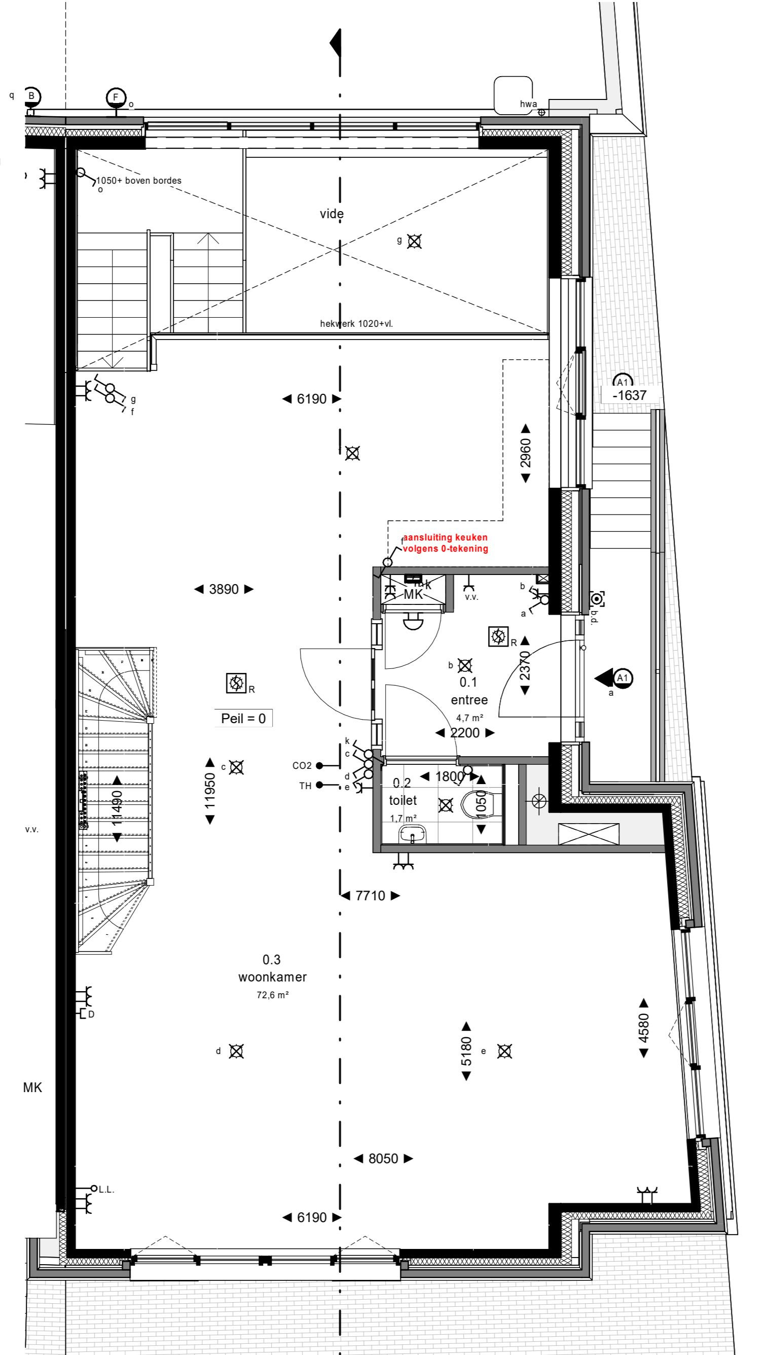
Begane grond 1 : 50
