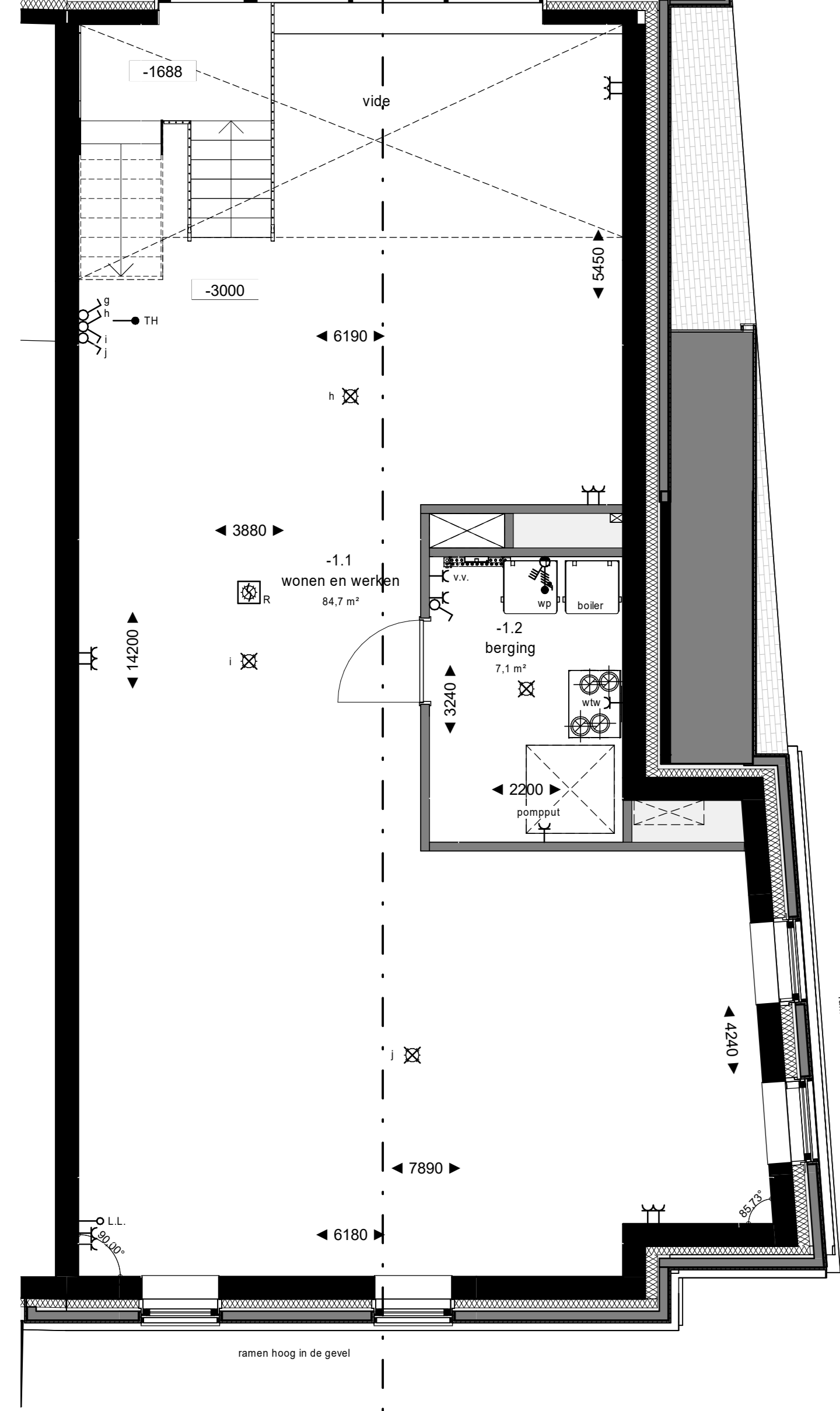
Souterrain 1 : 50
