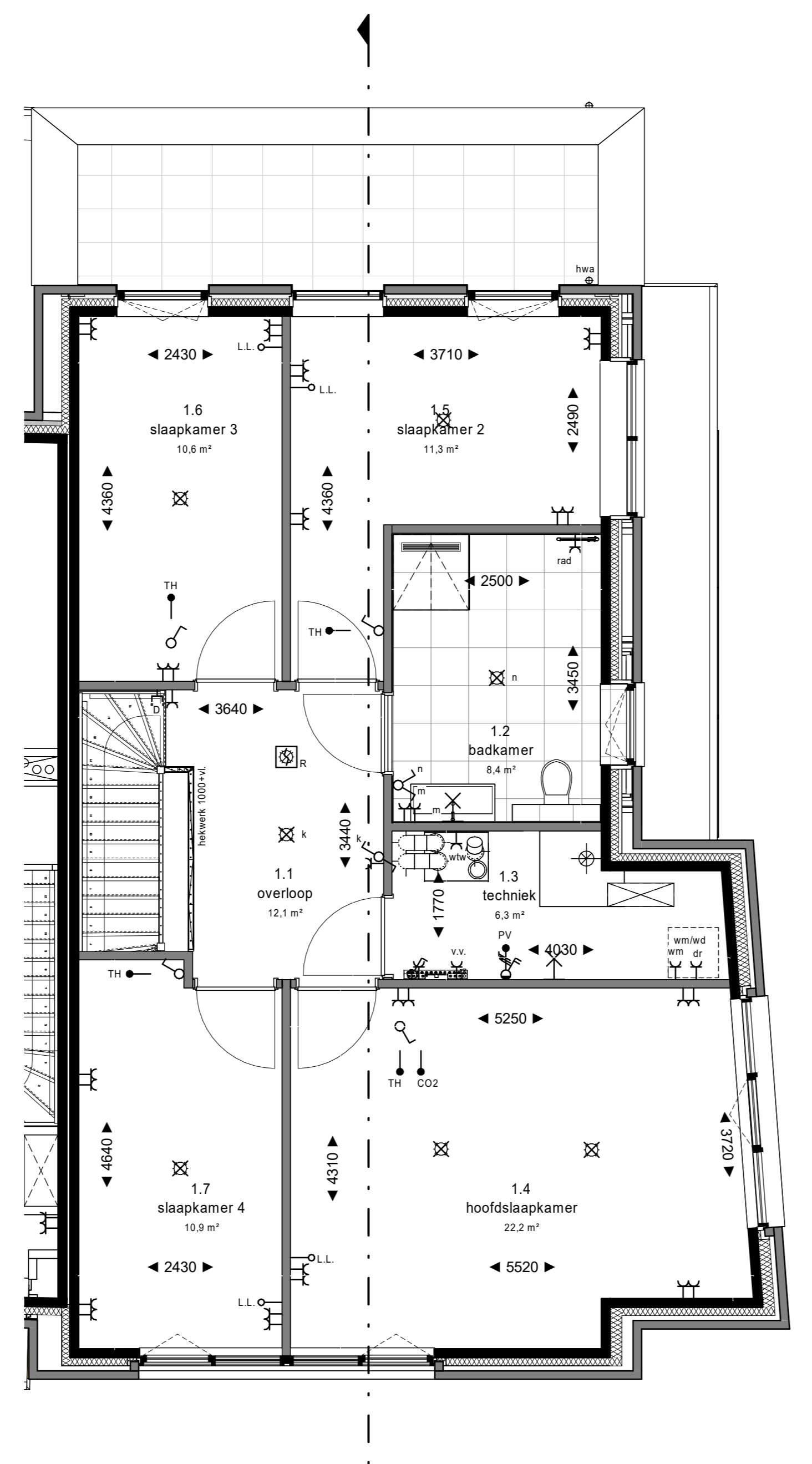
1e verdieping 1 : 50
