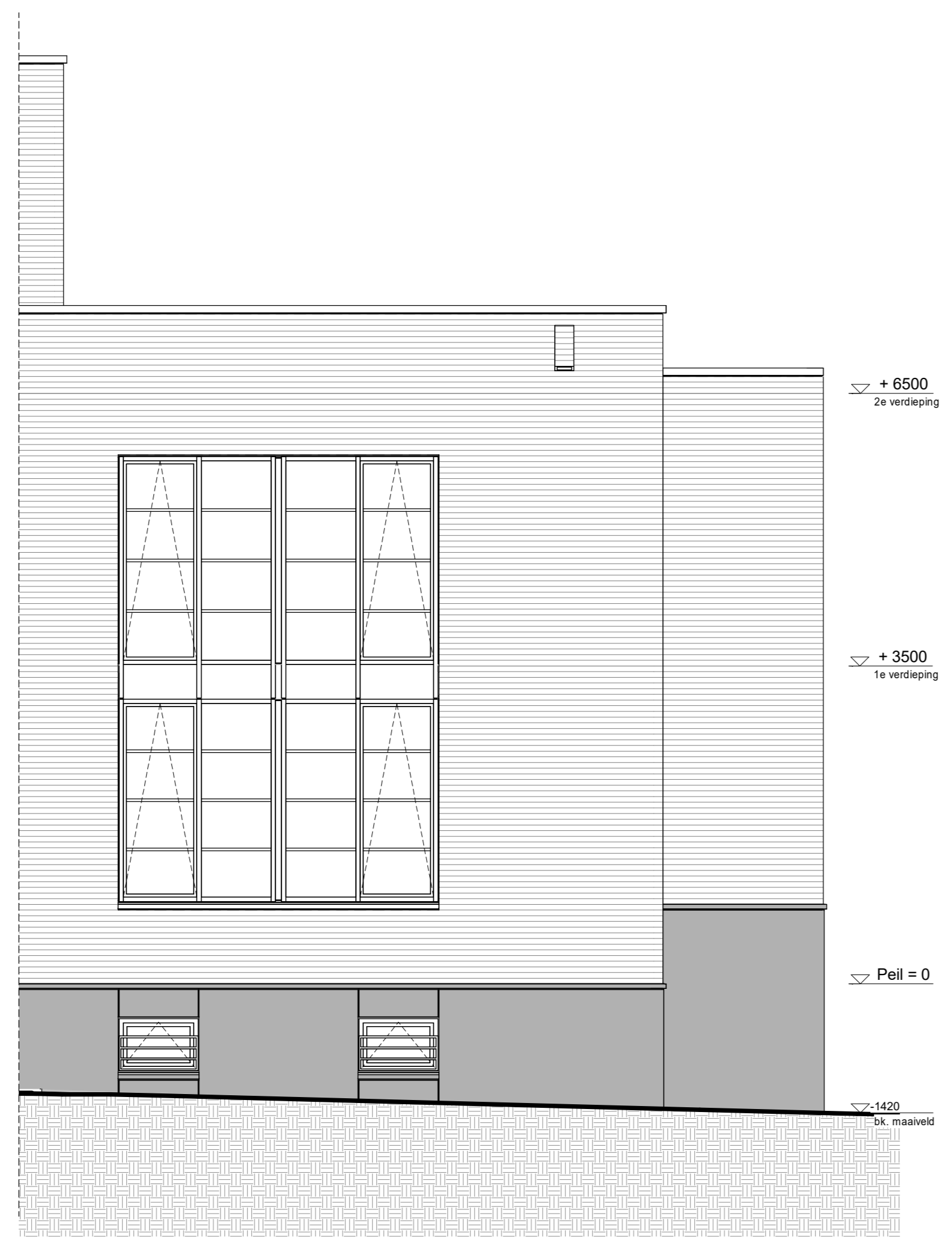
Voorgevel 1 : 50
