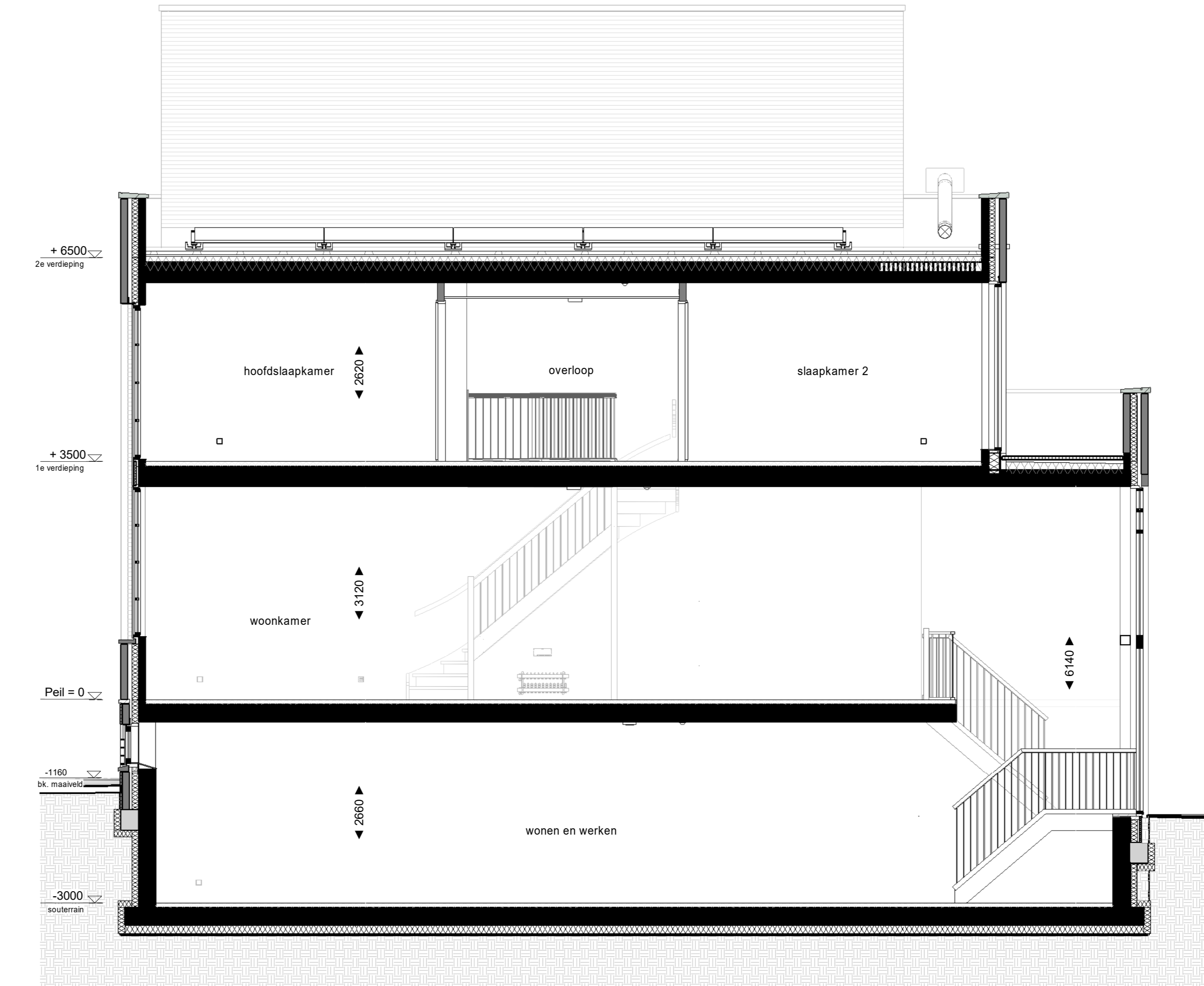
Doorsnede 1 : 50
