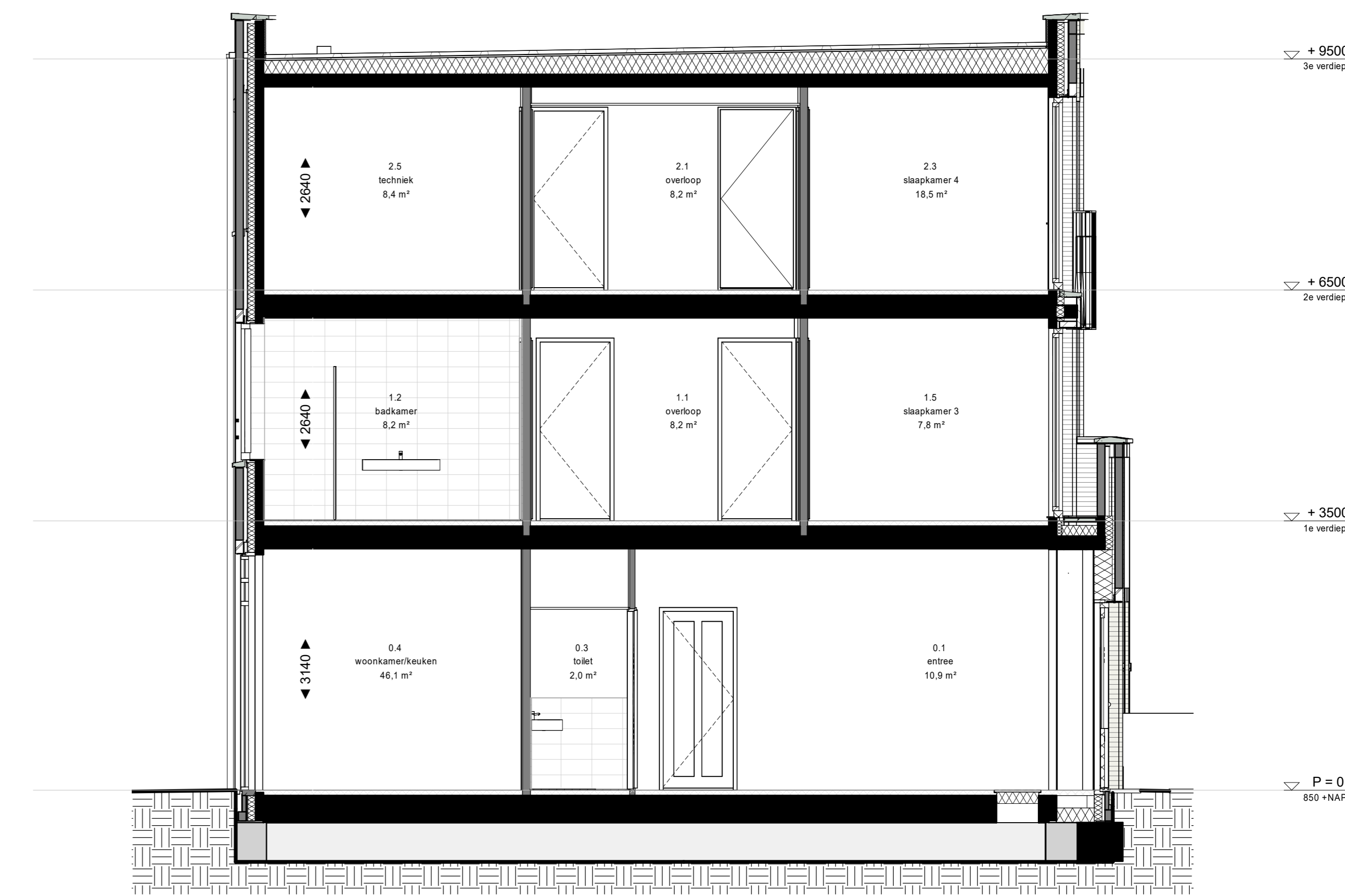
doorsnede
