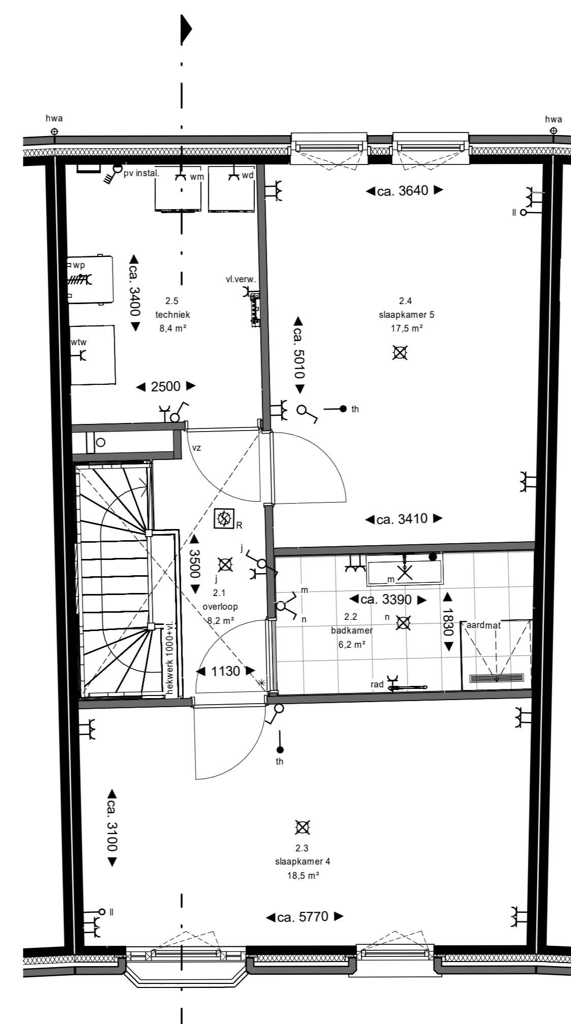
2e verdieping
