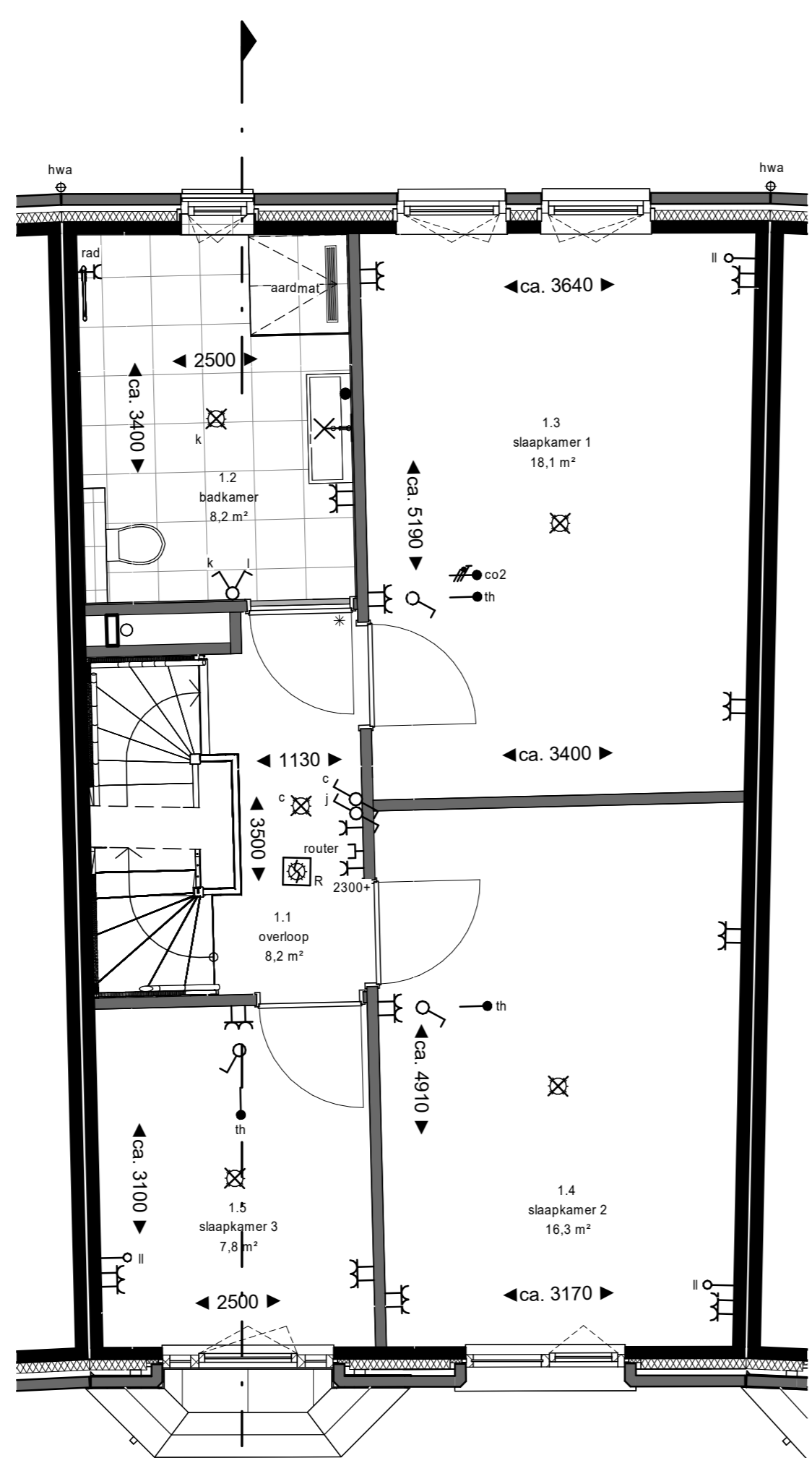
1e verdieping
