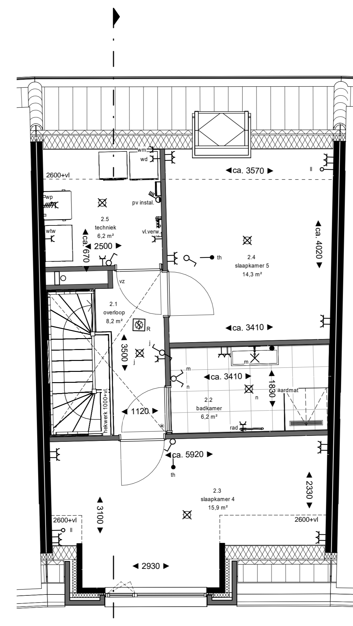
2e verdieping
