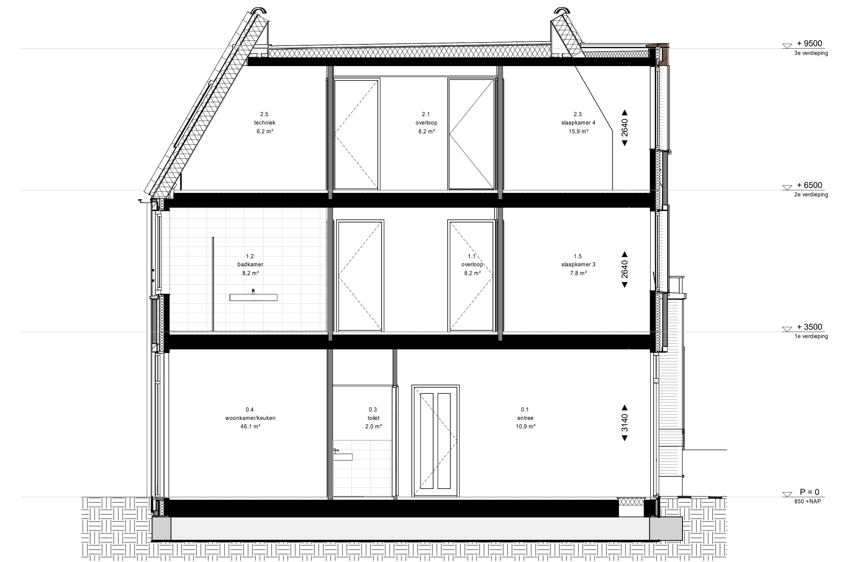
doorsnede
