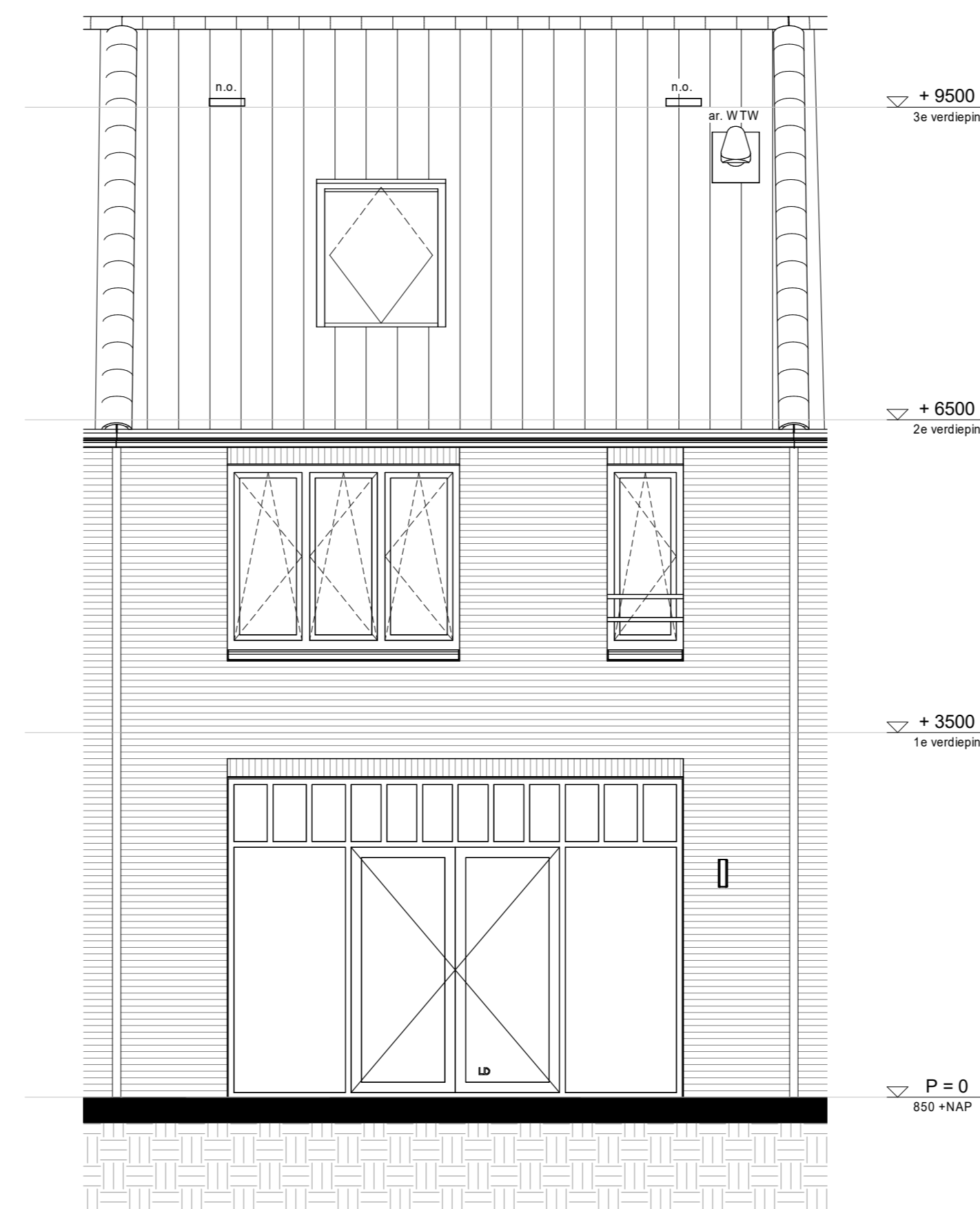
achtergevel
