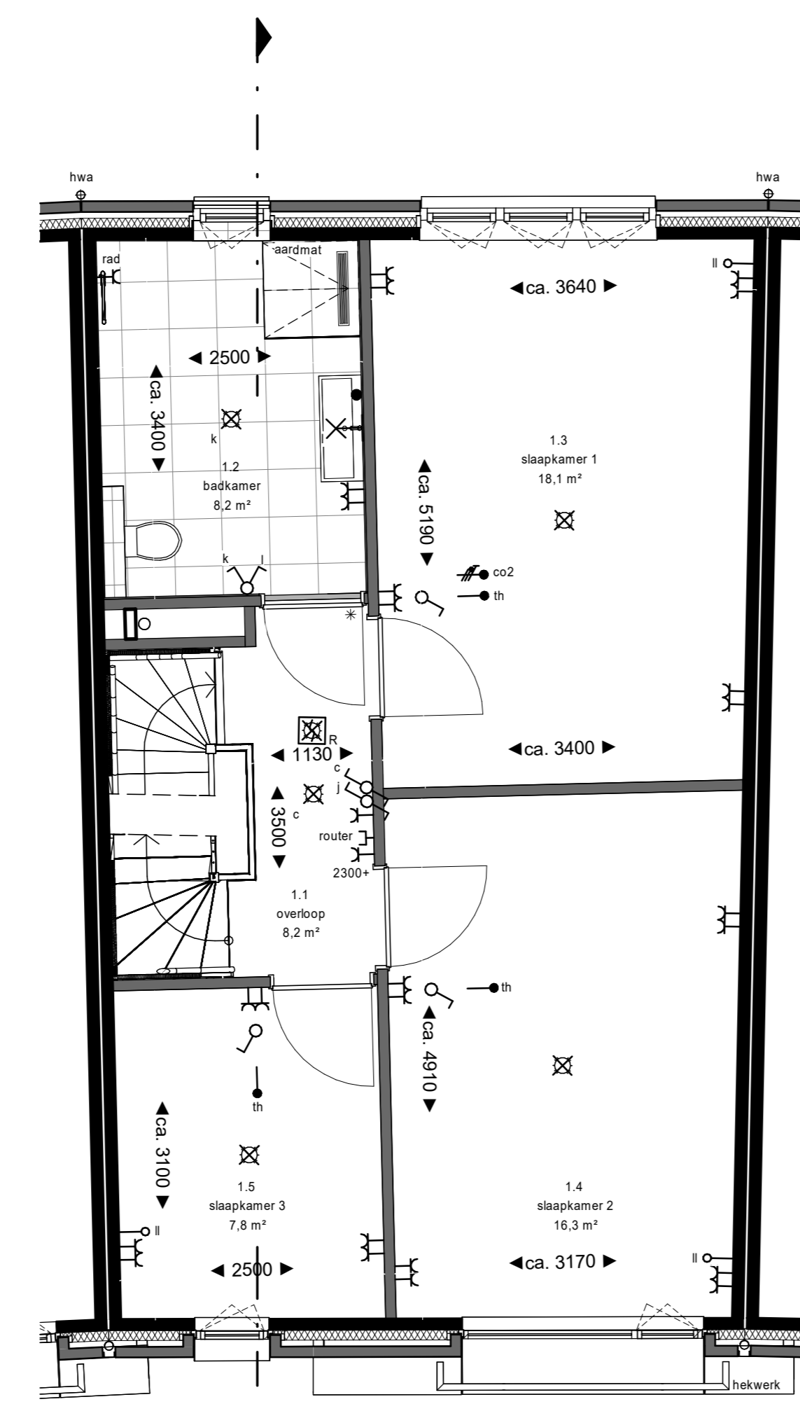
1e verdieping
