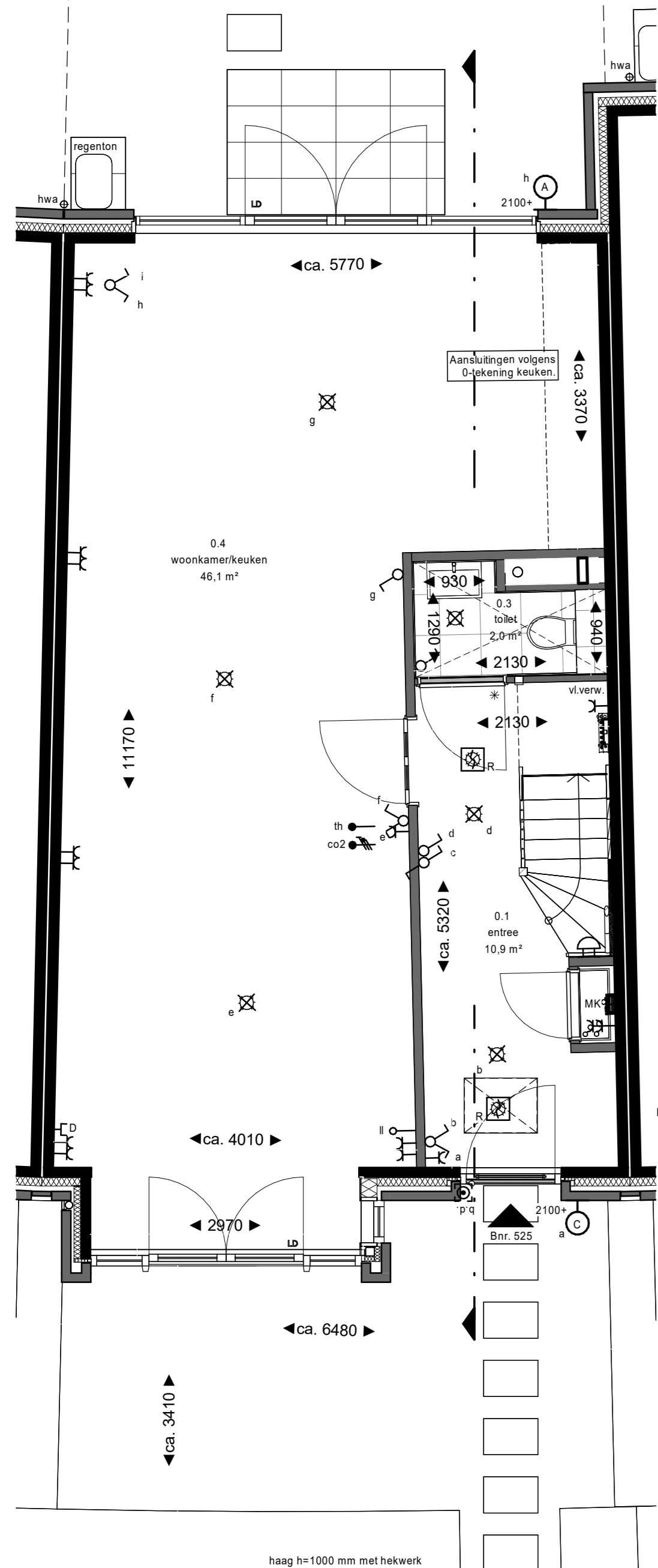
begane grond
