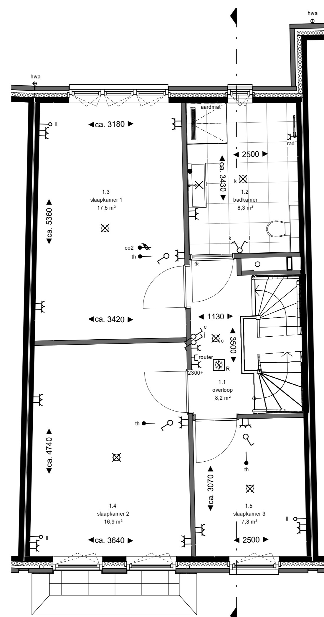
1e verdieping
