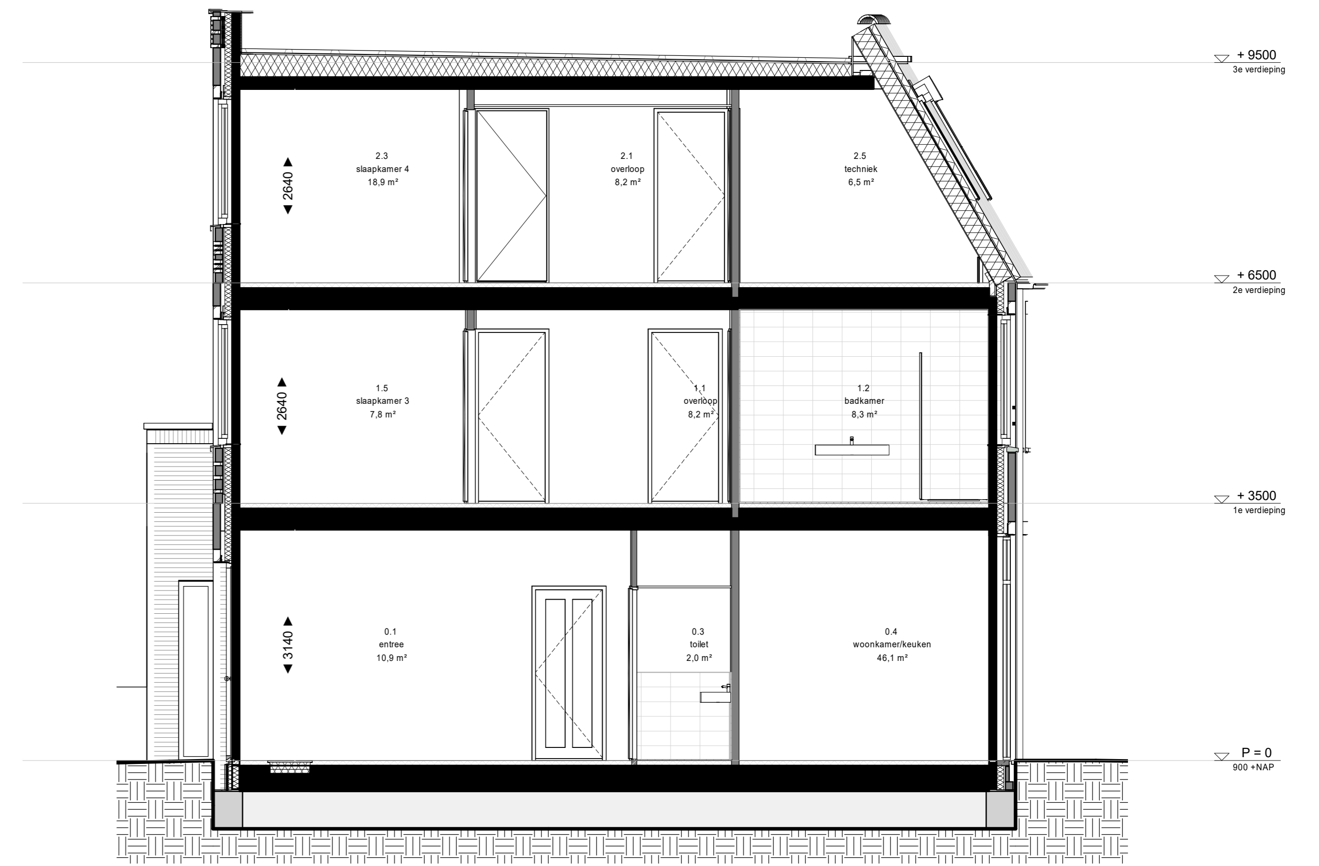
doorsnede
