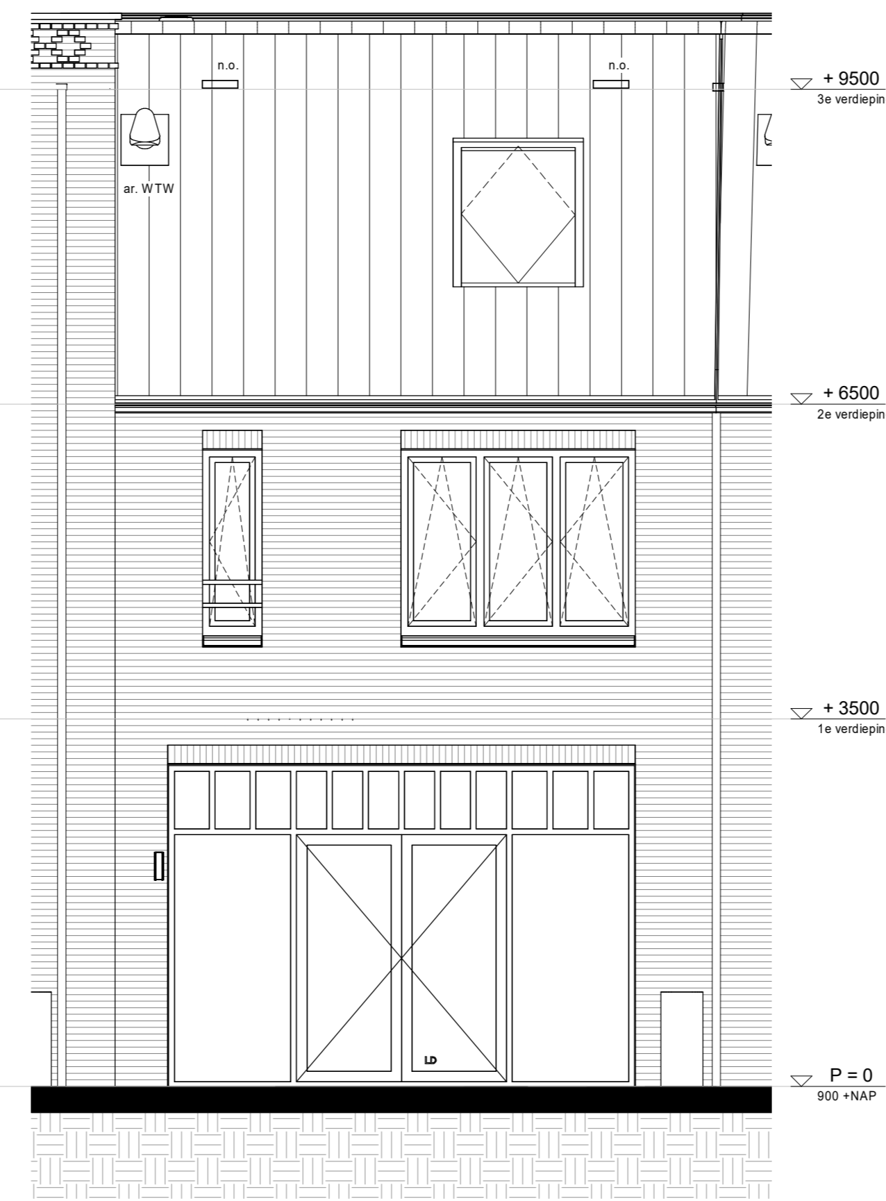
achtergevel
