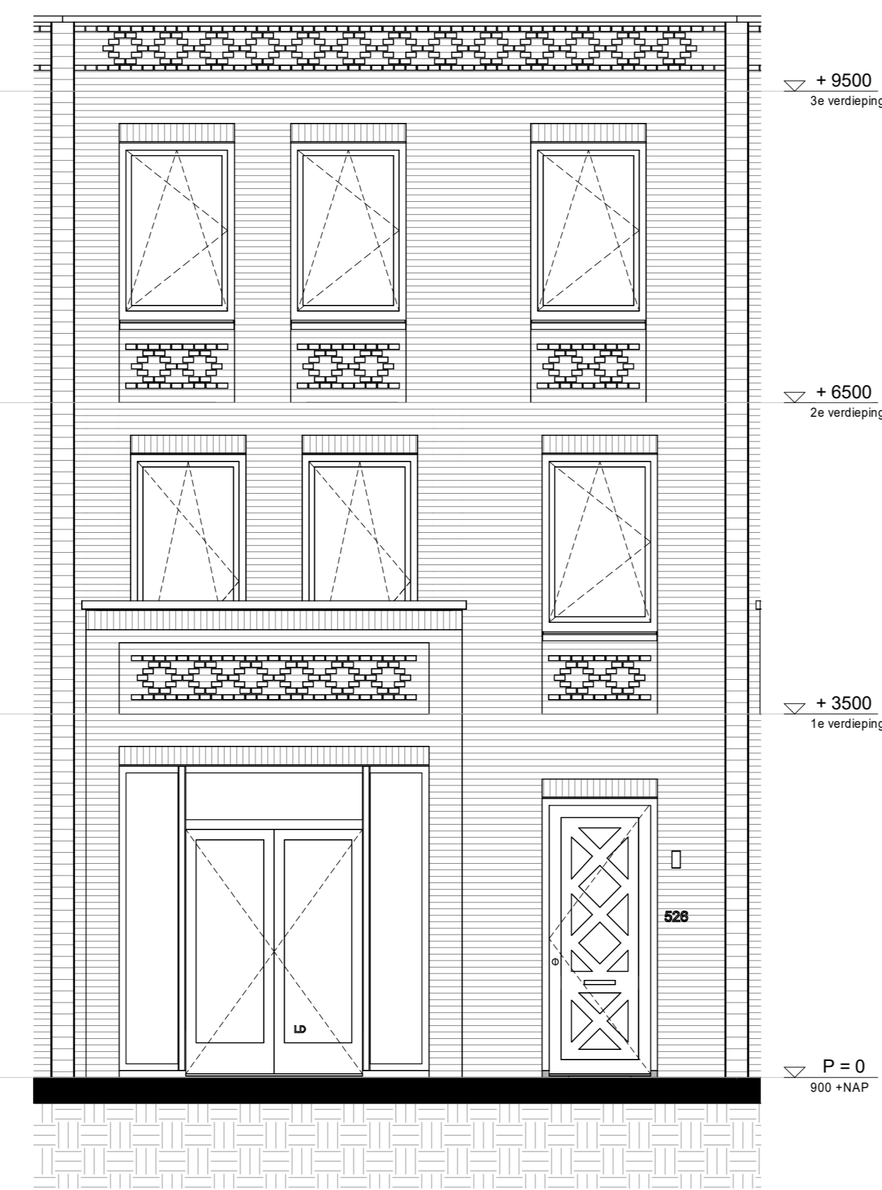
voorgevel
