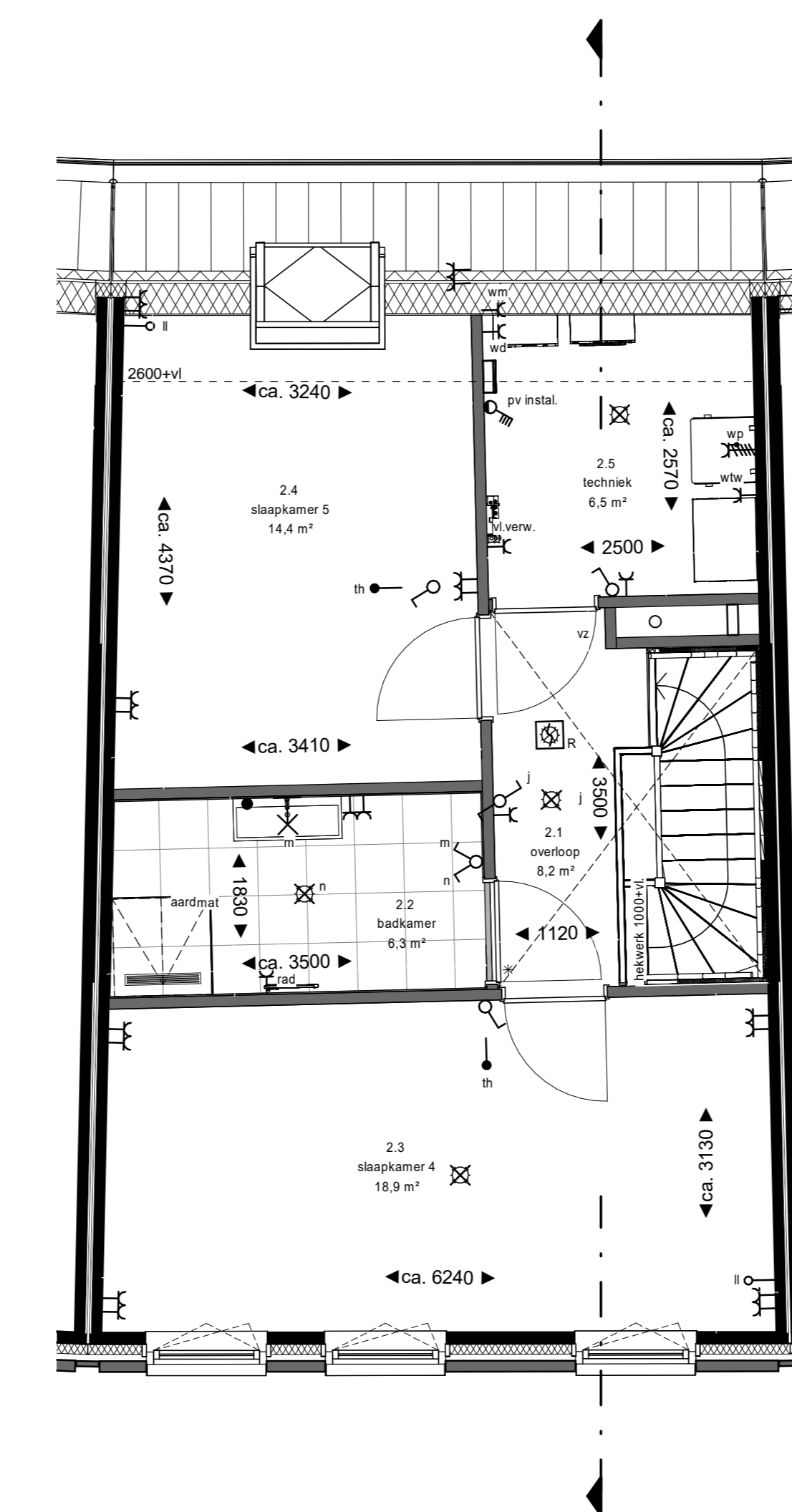
2e verdieping
