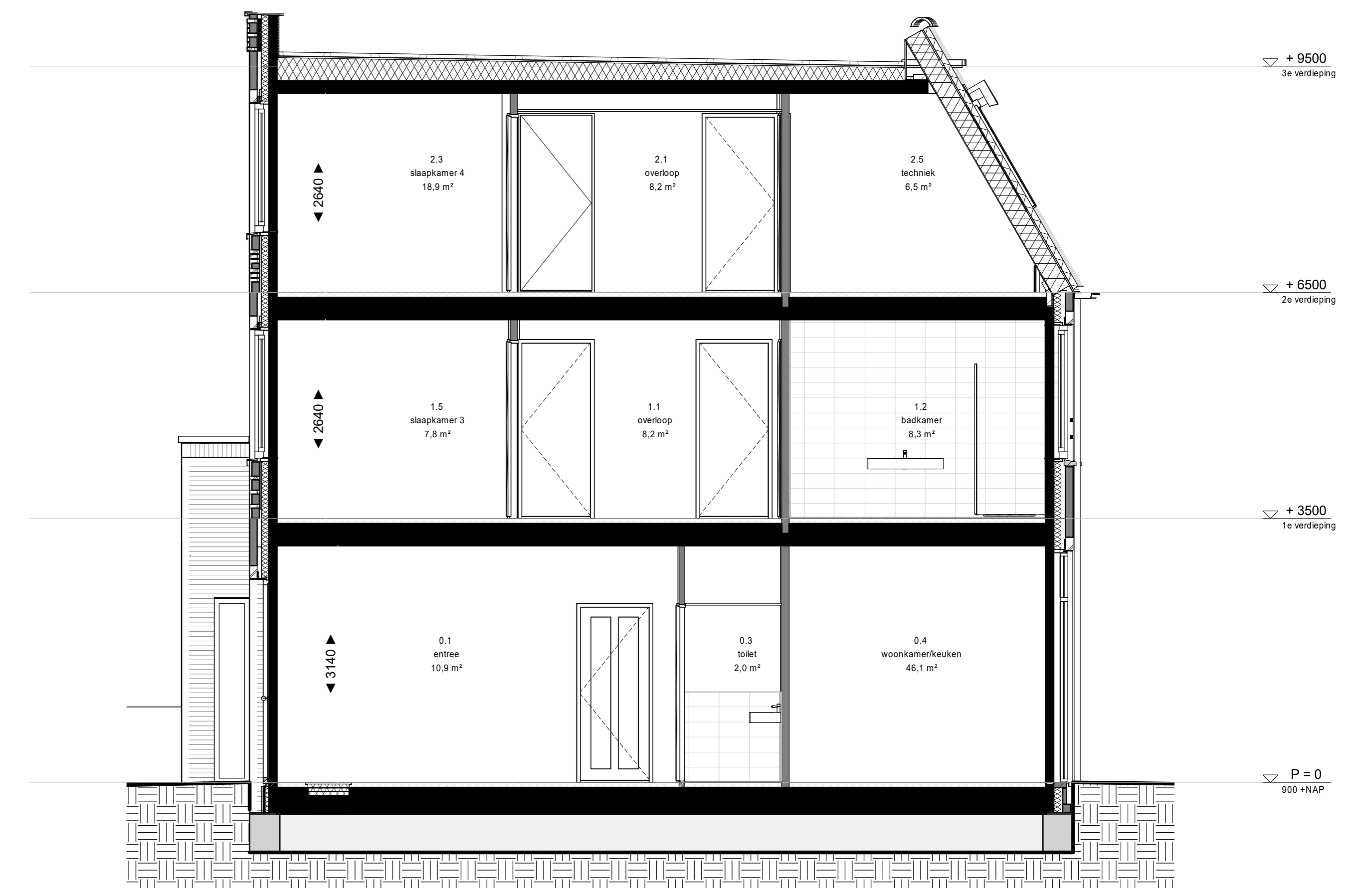
doorsnede
