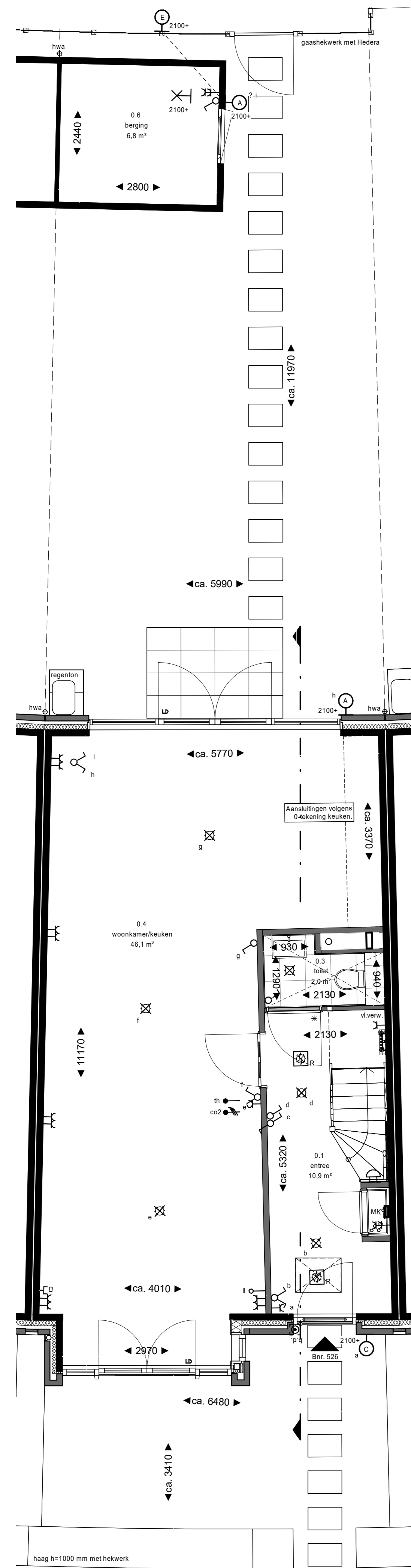
begane grond
