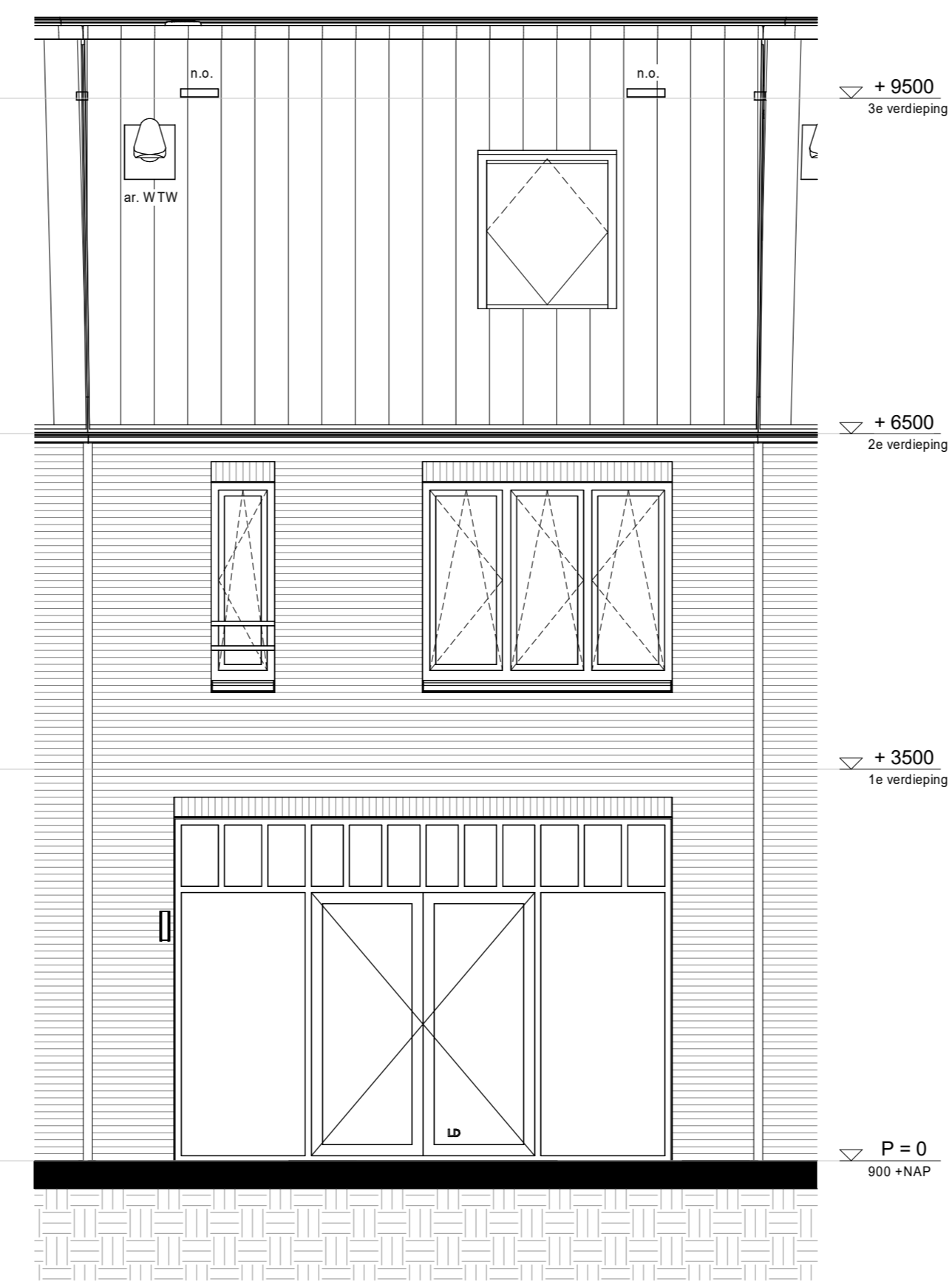
achtergevel
