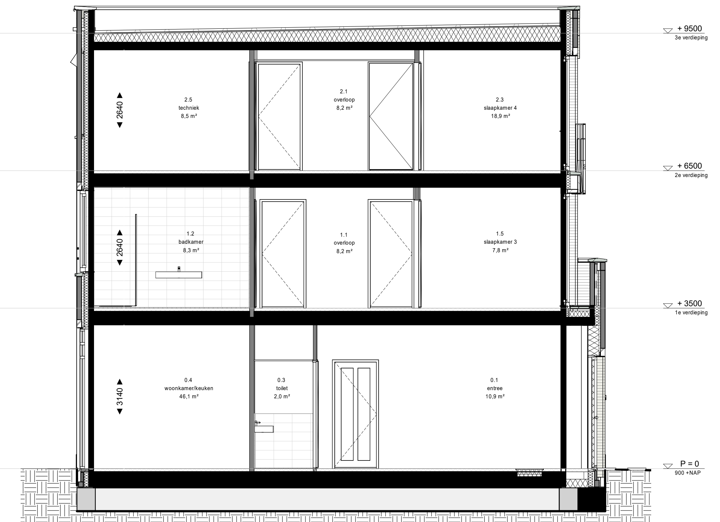
doorsnede
