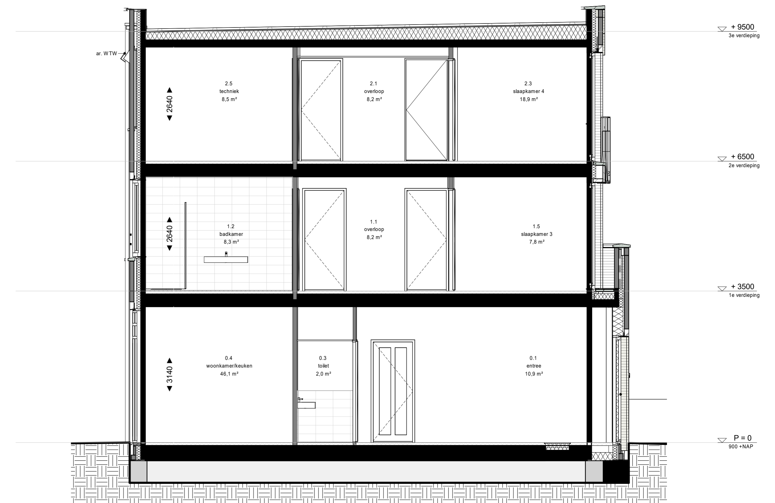
doorsnede
